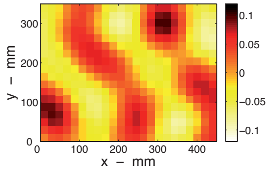
(b) Pressions identifiées à 1900 Hz
