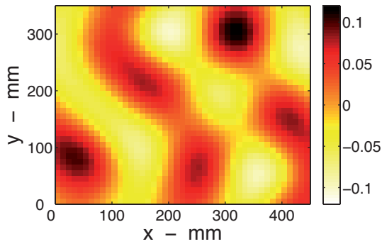
(a) Pressions de références à 1900 Hz
