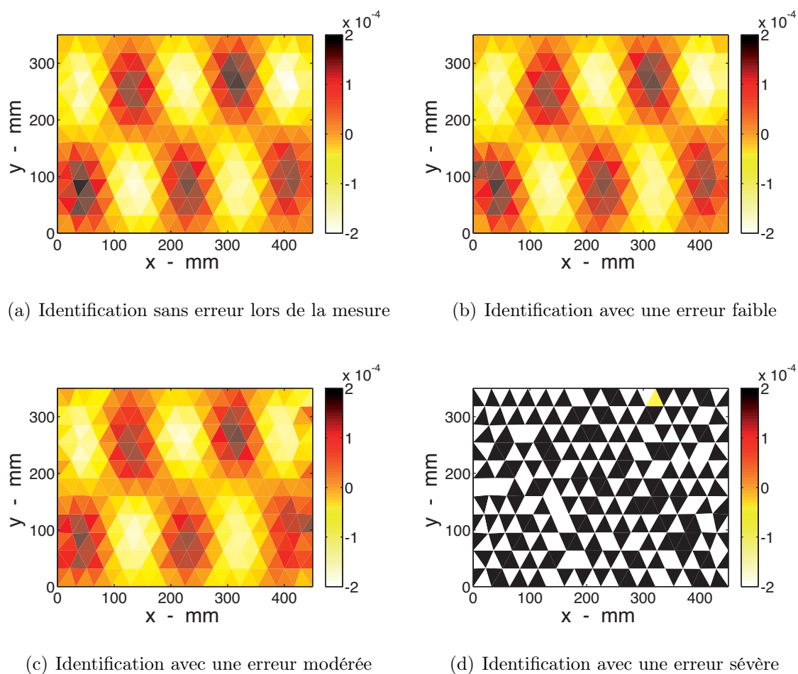
FIGURE 5.13 – Identification du champ de vitesses de la source à 1900 Hz
