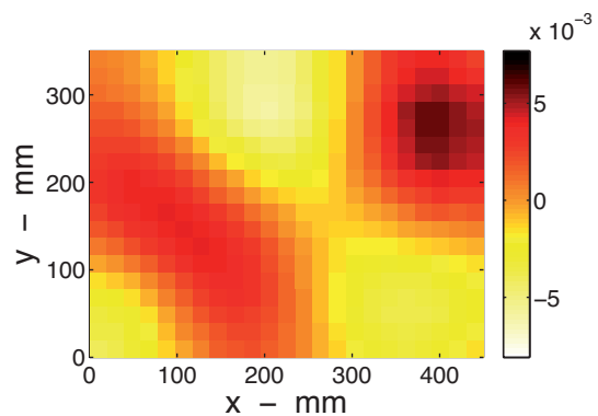
(d) Pressions identifiées à 800 Hz
