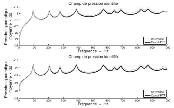
FIGURE 5 – Comparaison des spectres des pression et vitesse simulées et identifiées sur la plaque
