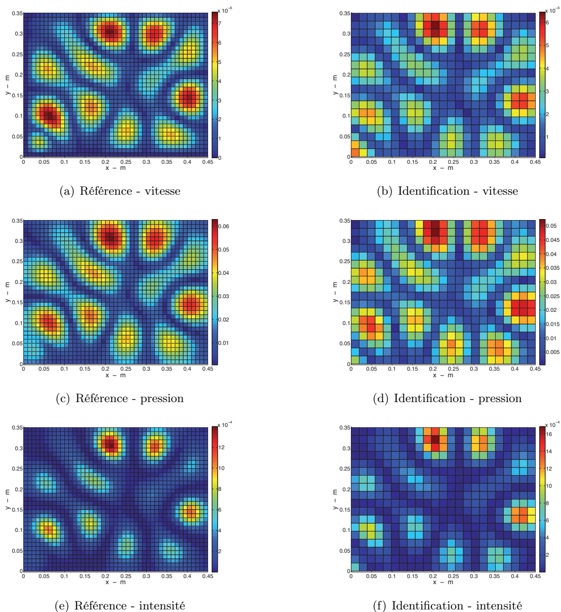
FIGURE 5 – Cartographies rétropropagées
