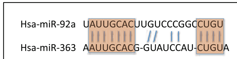
Figure 32. Comparaison entre les paralogues miR-92a et miR-363.
