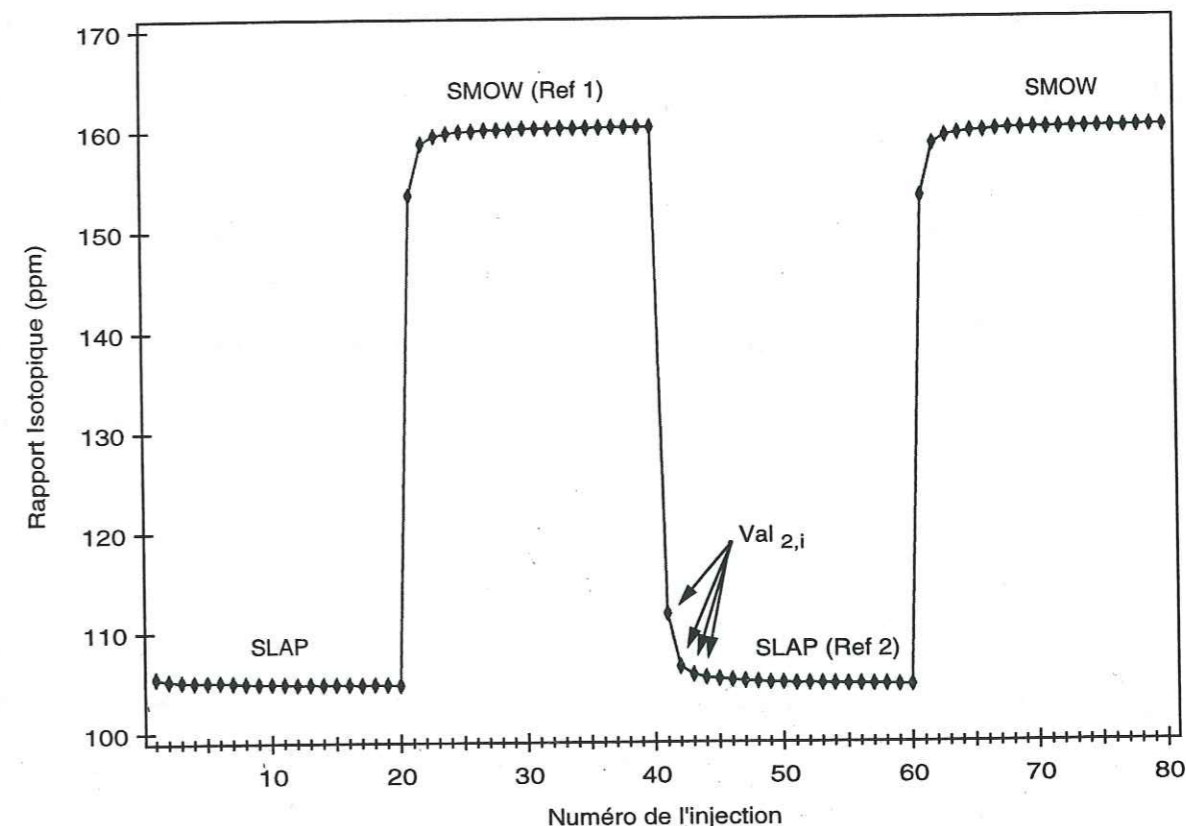
Figure 1-I-2 : Exemple type de calibration effectuée pour le calcul des coefficients mémoires.
