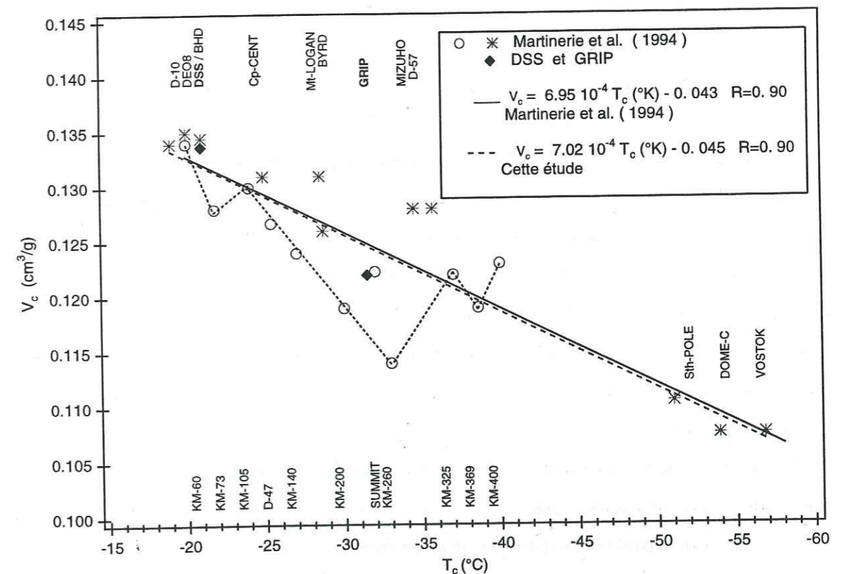
Figure 4-III-1 : Variation de la porosité au close-off en fonction de la température au close-off. Paramétrisation de V_c pour les périodes récentes.
