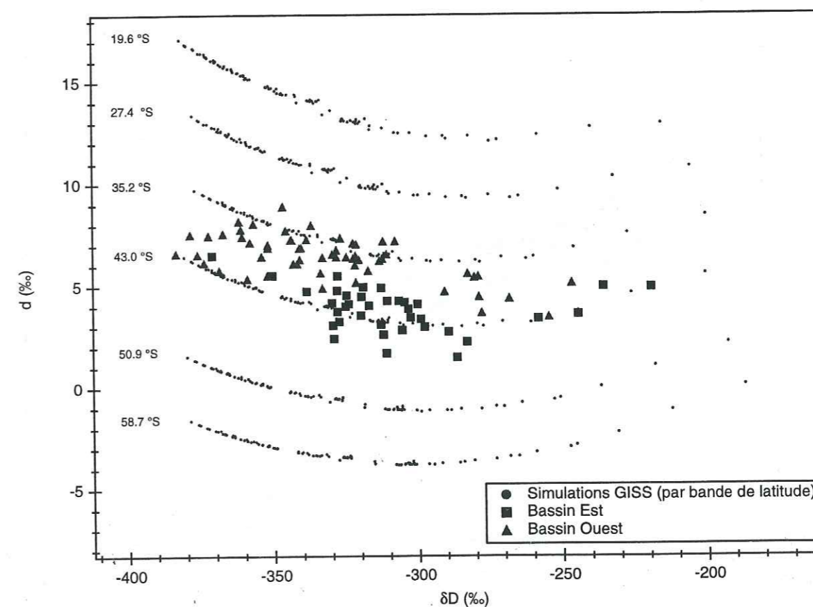
Figure 2-III-3 : Diagramme d- \delta D pour les simulations du MCIM, forcé par les \delta_0 du modèle ECHAM 3 (en haut) et du GISS (en bas). Comparaison aux données pour la région du Glacier Lambert.
