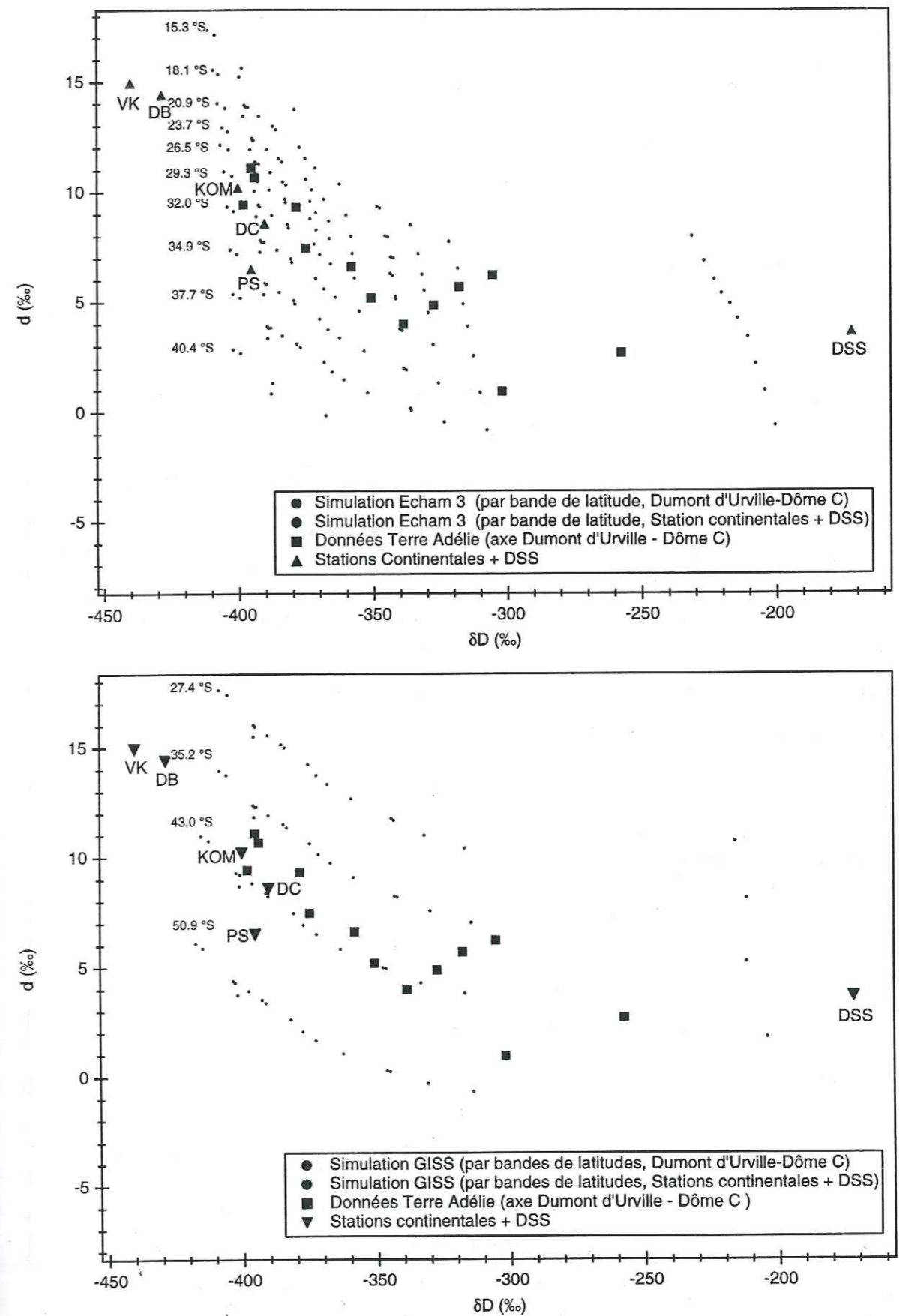
Figure 2-III-5 : Diagramme d- \delta D pour les simulations du MCIM, forcé par les \delta_0 du modèle ECHAM 3 (en haut) et du GISS (en bas). Comparaison aux données pour la région de la Terre Adélie et des stations antarctiques : Vostok, Dôme B, Dôme C, Pôle Sud, Komsomolskaya et DSS.
