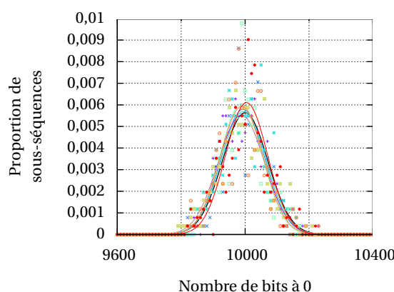
(b) Sortie du correcteur de von Neumann.
