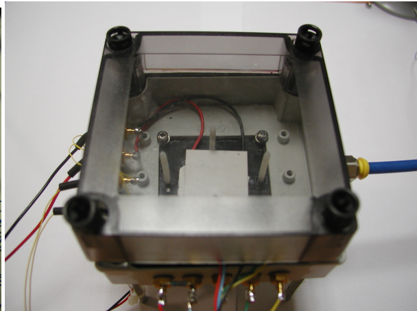
(b) Montage sous vide.
