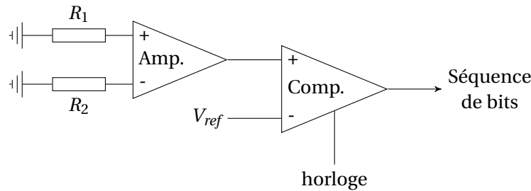
FIGURE 2.3 – Amplification différentielle du bruit thermique.
