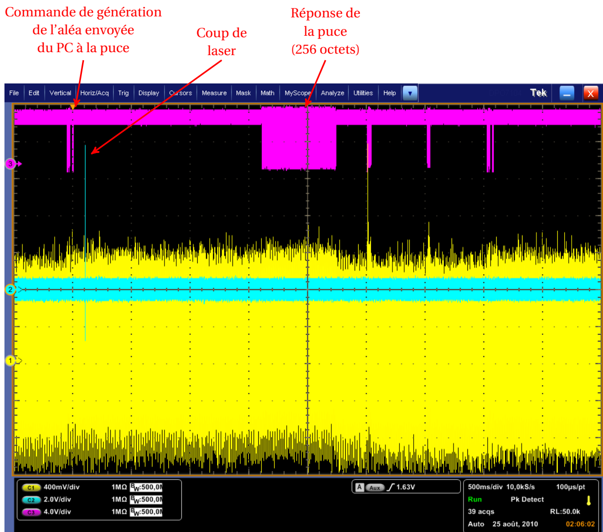
FIGURE 6.6 – Visualisation de la réponse de la puce et des différents signaux lors d'un coup de laser entrainant l'apparition de deux octets à 0.
