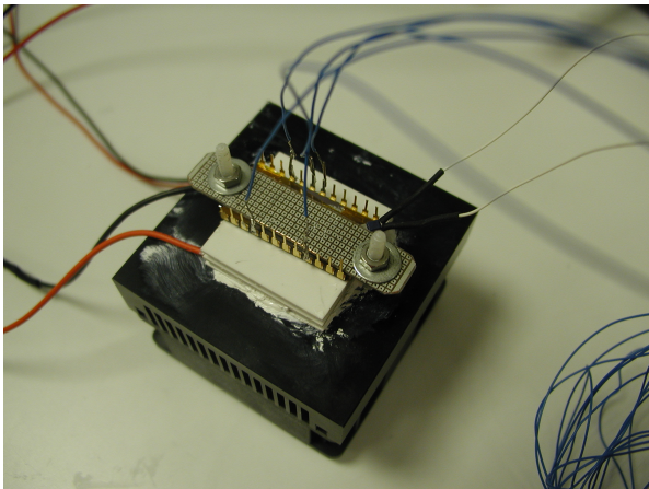
(a) Montage à l'air libre.
