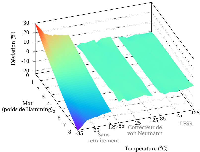
(b) Déviations dans la distribution des mots selon leur poids de Hamming.
