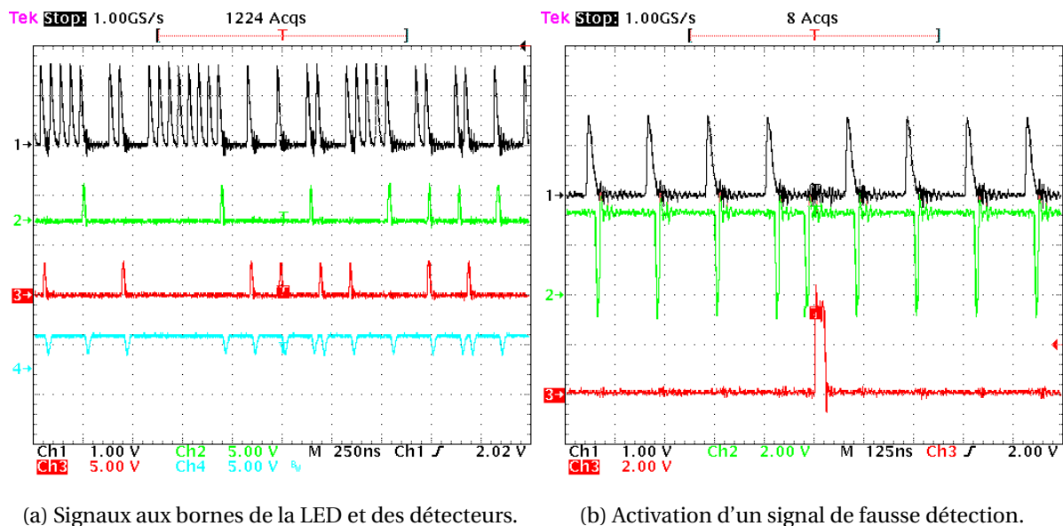
FIGURE 9.5 – Activation du signal d'erreur.
