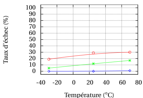
(d) Résultat des tests Rabbit (TestU01).
