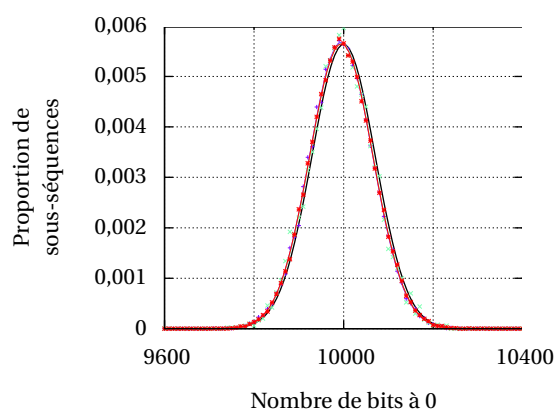
(c) Sortie du LFSR.
