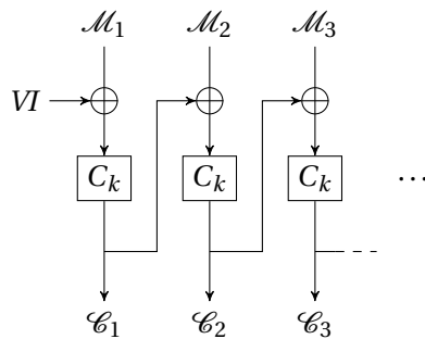
FIGURE 6.8 – Principe de fonctionnement du chiffrement pour un algorithme de chiffrement par blocs en mode CBC.
