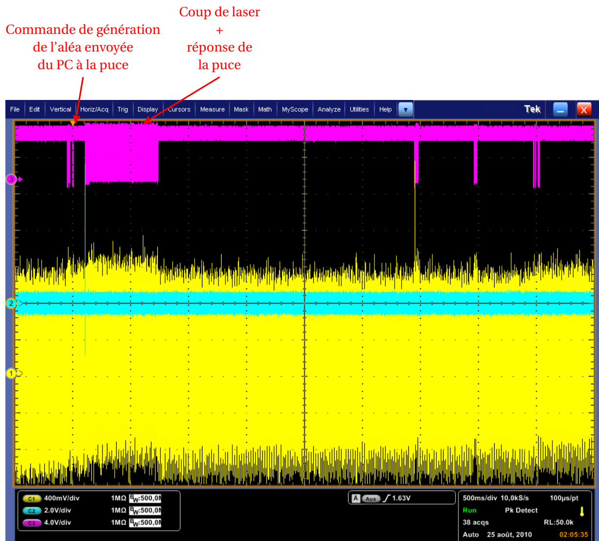
FIGURE 6.7 – Visualisation de la réponse de la puce et des différents signaux lors d'un coup de laser entrainant l'apparition d'une suite d'octets à 0.
