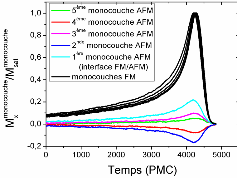
FIGURE 3.3.13 – Dépendance en temps de la composante suivant Ox de l'aimantation réduite des monocouches à B_C^+ pour l'interface plane ( D_y^{AFM}/J_{FM} = 0,06 ).
