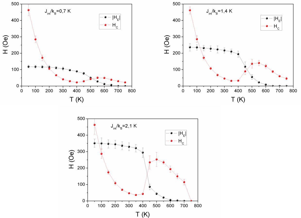
FIGURE 4.5.13 – Evolution des champs coercitif et d'échange en fonction de la température, pour une couche polydisperse ( J_{FM} \neq 0 ) avec différentes valeurs du couplage interfacial J_{int} ( J_{int}/k_B = 0,7 K en haut à gauche, J_{int}/k_B = 1,4 K en haut à droite et J_{int}/k_B = 2,1 K en bas).
