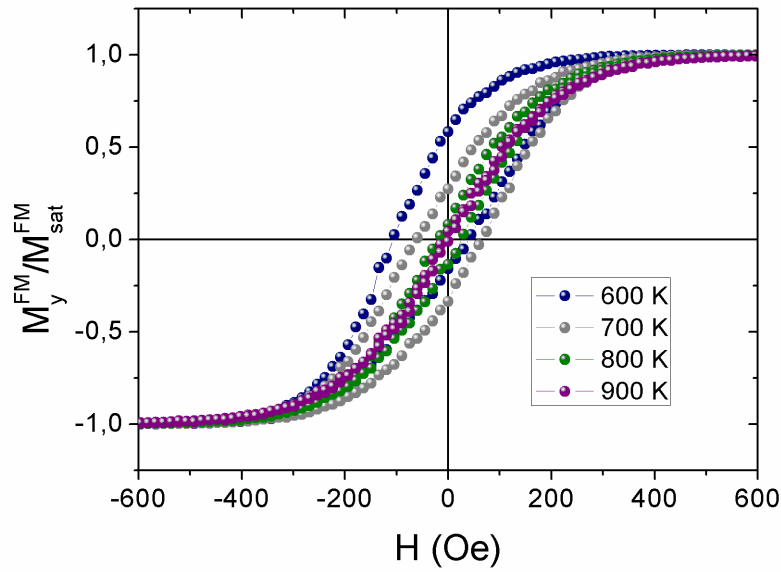
FIGURE 4.4.7 – Cycles d’hystérésis de la couche FM pour T \geq 600\text{K} ( J_{int} \neq 0 - J_{FM} = 0 ).
