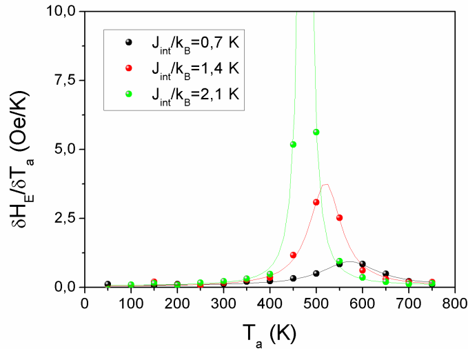
FIGURE 4.6.5 – Distributions de T_B^{AFM} pour différentes valeurs de J_{int} .
