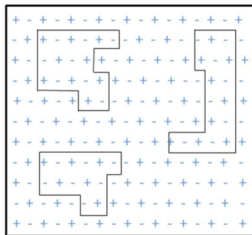
FIGURE 1.2.5 – Représentation schématique de l'effet de la rugosité sur l'orientation des spins interfaciaux AFM (les symboles + et - représentent les deux directions opposées des spins). Les traits continus représentent les marches (la hauteur des marches est d'un plan atomique).
