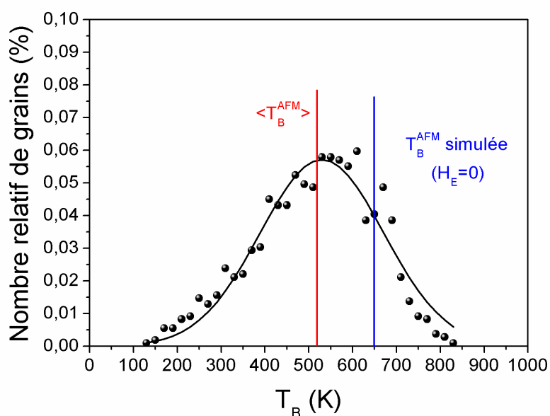
FIGURE 4.5.9 – Distribution des températures de blocage calculée des grains AFM ( \langle T_B^{AFM} \rangle = 515 K, \sigma = 138 K) ( J_{int} \neq 0 - J_{FM} = 0 ).
