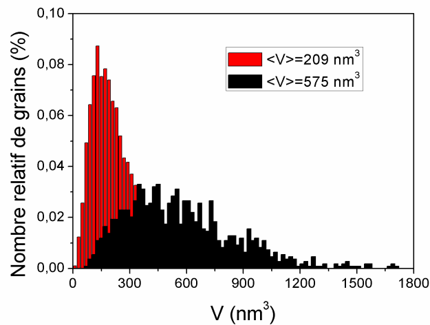
FIGURE 4.6.7 – Distribution volumique pour deux microstructures de volume moyen et d'écart-type différents (en rouge : \langle V \rangle = 209 \text{ nm}^3 et \sigma = 114 \text{ nm}^3 , en noir : \langle V \rangle = 575 \text{ nm}^3 et \sigma = 308 \text{ nm}^3 ).
