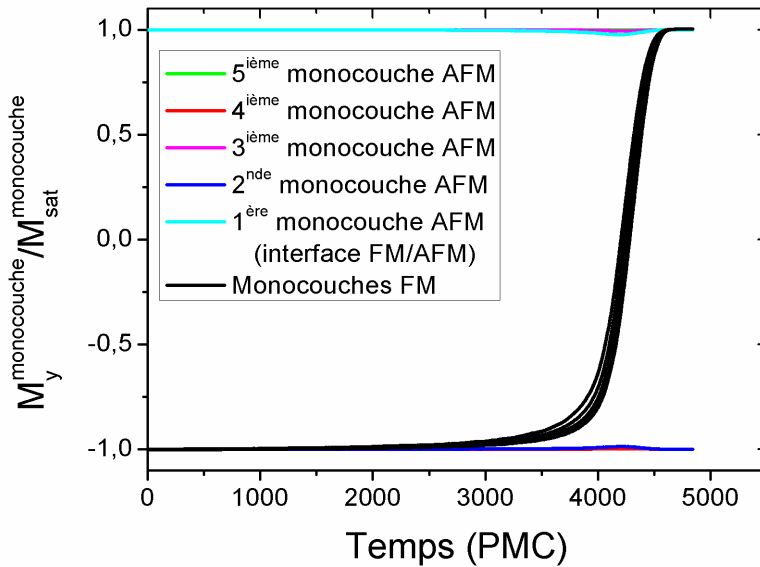
FIGURE 3.3.14 – Dépendance en temps de la composante suivant Oy de l'aimantation réduite des monocouches à B_C^+ pour l'interface plane ( D_y^{AFM}/J_{FM} = 0,06 ).
