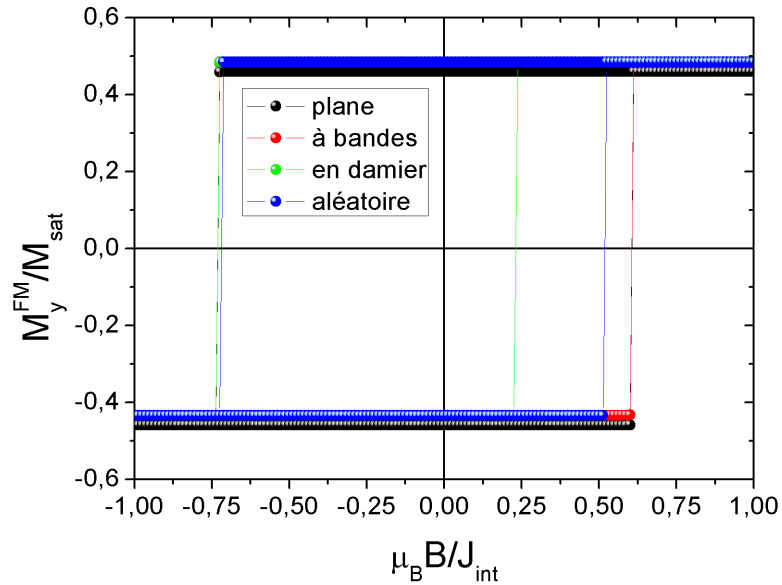
FIGURE 3.3.2 – Cycles d’hystérésis simulés pour les quatre interfaces avec l’état fondamental comme état initial. Le décalage vertical des interfaces rugueuses est dû au plan interfacial mixte qui peut être soit saturé, soit antiferromagnétique.
