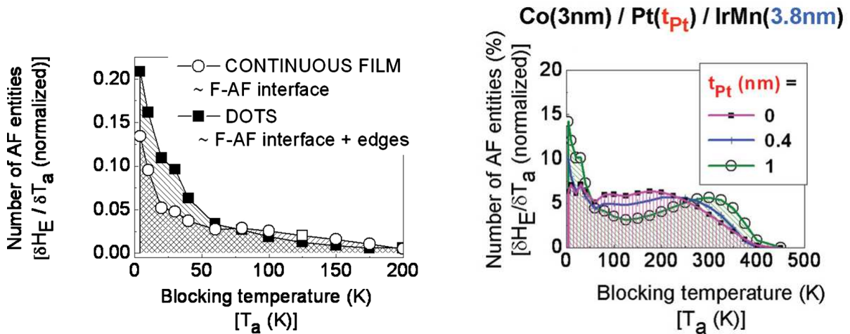
FIGURE 4.6.16 – Distributions de T_B^{AFM} obtenues expérimentalement pour un système constitué de réseau de plots (à gauche) [71] et d’un système présentant une couche de Platine à l’interface entre la couche FM (Co) et AFM (IrMn) (à droite) [90].
