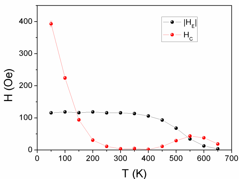
FIGURE 4.5.8 – Evolution des champs coercitif et d’échange en fonction de la température pour une distribution polydisperse ( J_{int} \neq 0 - J_{FM} = 0 ).
