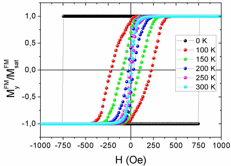
FIGURE 4.5.3 – Cycles d'hystérésis de la couche FM à différentes températures ( J_{int} = J_{FM} = 0 ).
