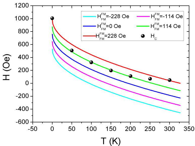
FIGURE 4.4.14 – Comparaison de H_{sw}(T) + H_E et H_C(T) pour différentes valeurs de H_{FM}^{FM} .
