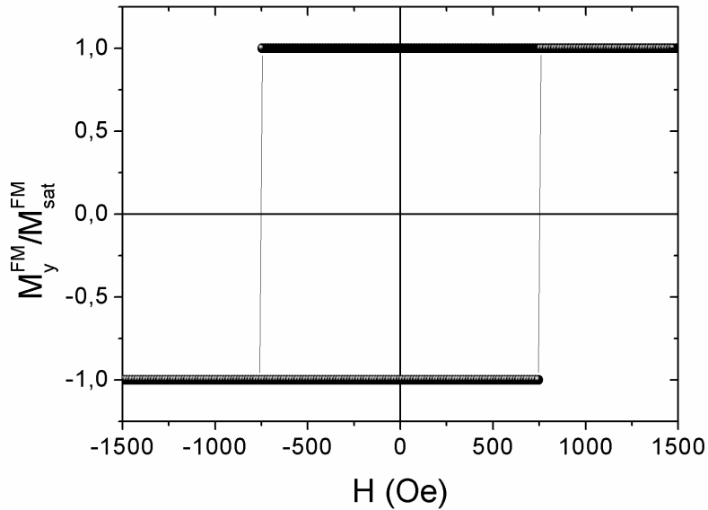
FIGURE 4.4.1 – Cycle d'hystérésis de la couche FM à très basse température ( T \approx 0 \text{ K} ) ( J_{int} = J_{FM} = 0 ).
