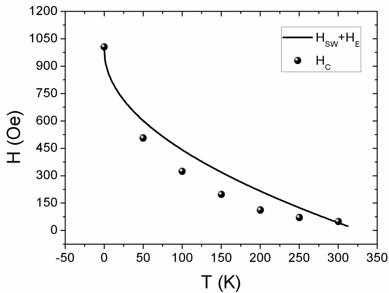
FIGURE 4.4.13 – Evolution du champ coercitif en fonction de la température ( J_{int} \neq 0 - J_{FM} \neq 0 ), comparaison à l'expression (4.4.4).
