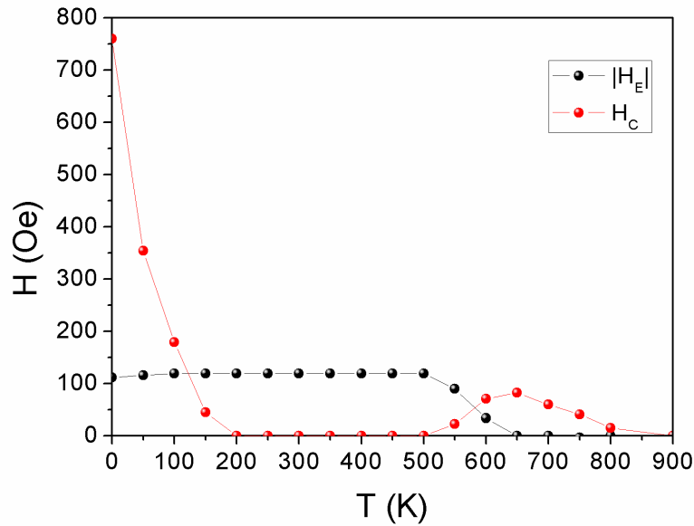
FIGURE 4.4.8 – Évolution des champs coercitif et d’échange en fonction de la température ( J_{int} \neq 0 - J_{FM} = 0 ).
