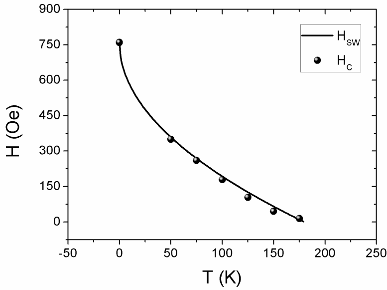
FIGURE 4.4.3 – Évolution du champ de retournement avec la température ( J_{int} = J_{FM} = 0 ), comparaison à l'expression (4.4.2).
