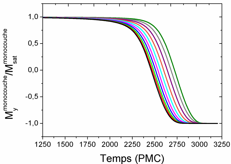
FIGURE 3.3.3 – Dépendance en temps de la composante suivant Oy de l’aimantation réduite des monocouches durant le premier retournement pour l’interface plane (de gauche à droite : interface libre à interface FM/AFM).
