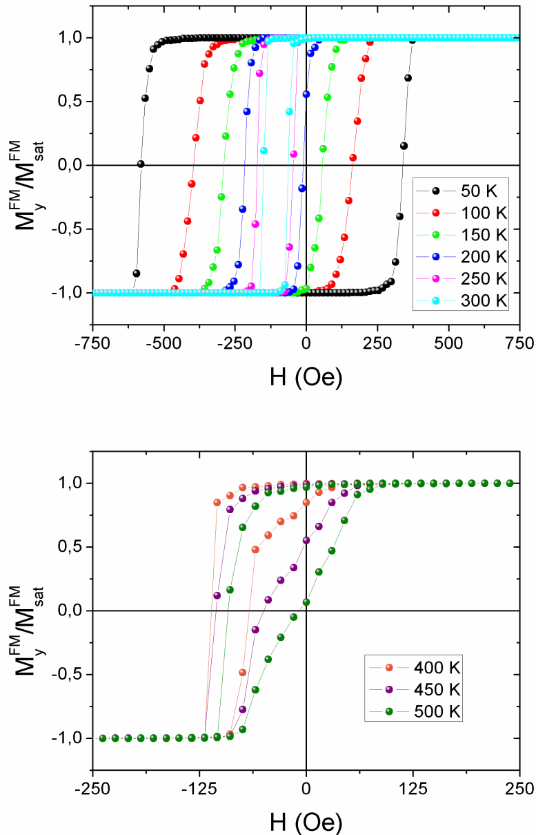
FIGURE 4.5.11 – Cycles d'hysteresis de la couche FM pour différentes températures ( J_{int} \neq 0 - J_{FM} \neq 0 ).
