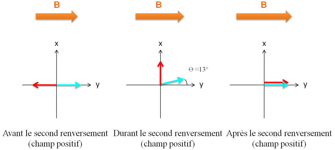
FIGURE 3.3.15 – Représentation schématique des moments FM et AFM à l'interface FM/AFM au cours du second retournement pour l'interface plane ( D_{AFM}^y/J_{FM} = 0,06 ).
