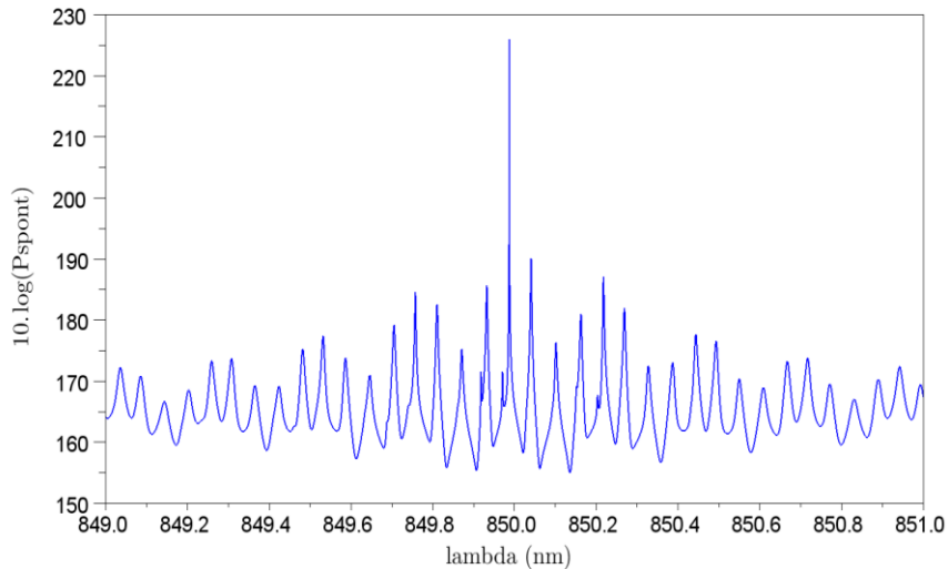
Figure 2-19: Spectre d'émission spontanée calculé pour un réseau de 0.4 nm de large, un laser de longueur 400 μm, des valeurs de réflectivité de 0.2 pour la facette droite du laser et 0.5 pour le filtre et une cavité externe de 5 mm (design 1)
