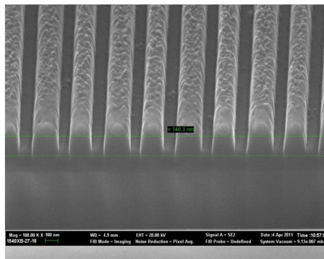
Figure 3-20 : Observation FIB d'un réseau résonant à deux atomes par maille
