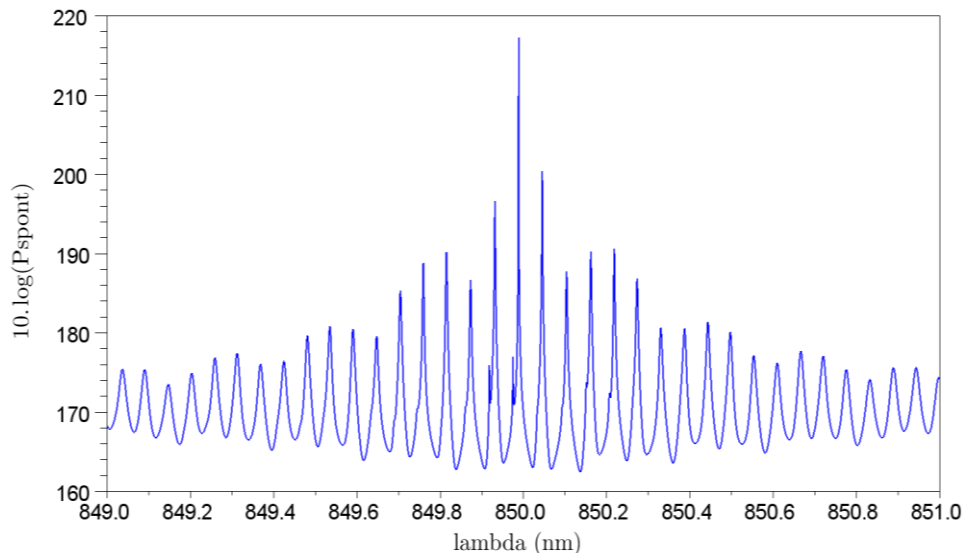
Figure 2-20 : Spectre d'émission spontanée calculé pour un réseau de 0.4 nm de large, un laser de longueur 400 μm des valeurs de réflectivité de 0.05 pour la facette droite du laser et 0.3 pour le filtre et une cavité externe de 5 mm (design 2)
