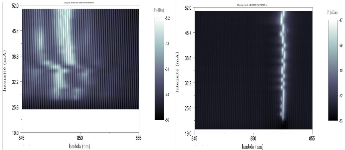
Figure 4-10 : Cartog a) : Centre optique d'une source laser Thalès en fonct b) : Centre optique d'une source laser Thalès en fonct situations : a) : sans réinjection et b) : avec réinjection du réseau résonant
