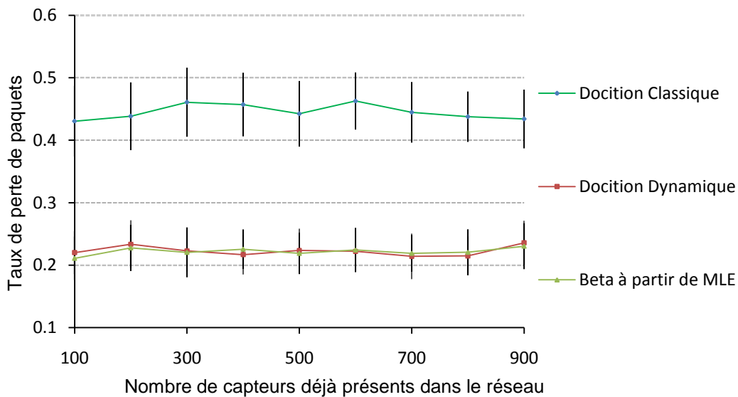
Figure 5.11: pourcentage d'overhead (graphe du haut) taux de perte (graphe inférieur), en fonction du nombre des nœuds existant déjà avant l'arrivée des nœuds étudiants
