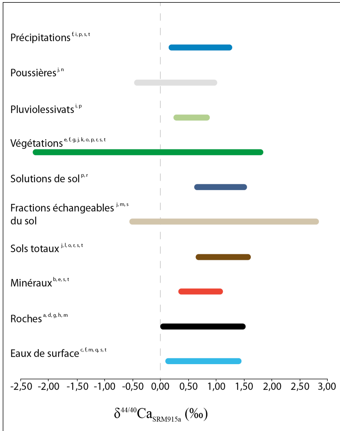
Figure 1.5 : Schéma récapitulatif des signatures isotopiques du Ca dans les différents réservoirs sur les continents. Les données sont issues de la littérature (Annexe 1). (a) Marshall et DePaolo (1982, 1989), (b) Skulan et al. (1997), (c) Zhu et MacDougall (1998), (d) Halicz et al. (1999), (e) Skulan et DePaolo (1999), (f) Schmitt et al. (2003), (g) Bullen et Bailey (2004), (h) DePaolo (2004), (i) Schmitt et al. (2005), (j) Wiengand et al. (2005), (k) Chu et al. (2006), (l) Pérakis et al. (2006), (m) Tipper et al. (2006), (n) Ewing et al. (2008), (o) Page et al. (2008), (p) Cenki-Tok et al. (2009), (q) Amini et al. (2009), (r) Holmden et Bélanger (2010), (s) Hindshow et al. (2011), (t) Farkas et al. (2011).
