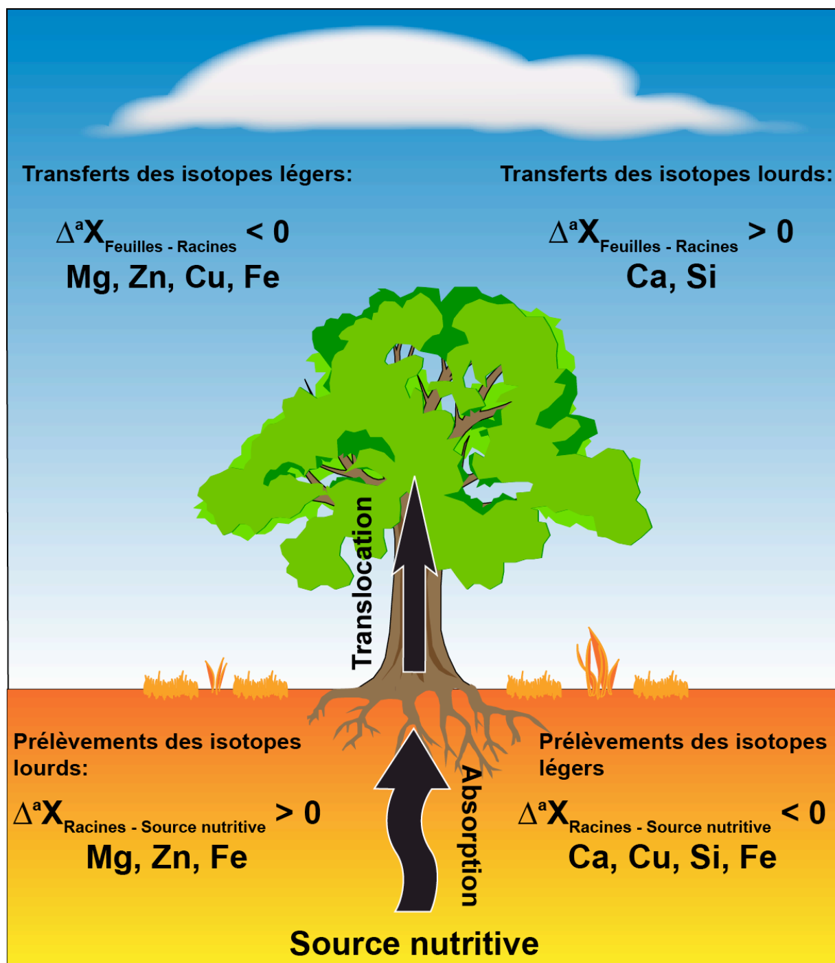
Figure I.6 : Variations des signatures isotopiques des isotopes stables non traditionnels ( ^aX = {}^{26}\text{Mg} , {}^{39}\text{Si} , {}^{44}\text{Ca} , {}^{57}\text{Fe} , {}^{65}\text{Cu} , {}^{66}\text{Zn} ) au sein des végétaux. Mg : Black et al. (2008), Bolou-Bi et al. (2010) ; Si : Ding et al. (2005), Opfergelt et al. (2006), Ding et al. (2008) ; Ca : Schmitt et al. (2003), Wiegand et al. (2005), Page et al. (2008), Cenko-Tok et al. (2009), Holmden et Bélanger (2010) ; Fe : Guelke and von Blanckenburg (2007) ; Cu : Weinstein et al., 2011, Jouvin et al. (2012) ; Zn : Weiss et al. (2005), Viers et al. (2007), Moynier et al. (2009), Aucour et al. (2011), Jouvin et al. (2012).
