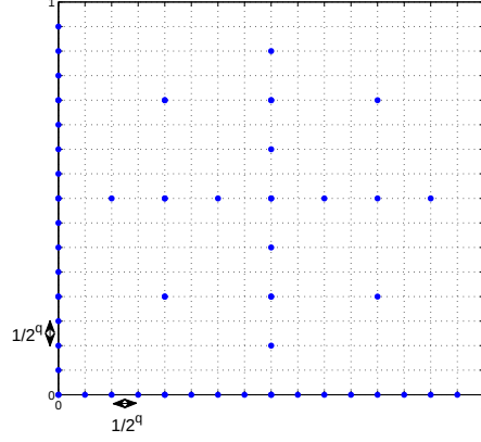
FIGURE 2.4 – Grille creuse pour l'interpolation de fonctions périodiques, avec q = 4 , d = 2 et \mathcal{X}_{k_1}^1 = \mathcal{X}_{k_2}^2 = \{0, 2^{-k_1}, \dots, (k_1 - 1) \times 2^{-k_1}\} .
