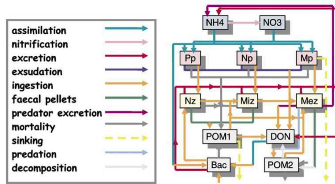
FIGURE 8.2 – Modèle biogéochimique. NH4 : Ammonium ; NO3 : nitrate ; Nz, Miz, Mez : nano-, micro-, mésozooplancton ; Pp, Np, Mp : pico-, nano-, microphytoplancton ; POM1, POM2 : matière organique particulaire de type 1 et 2 ; Bac : bactéries ; DON : azote organique dissous.
