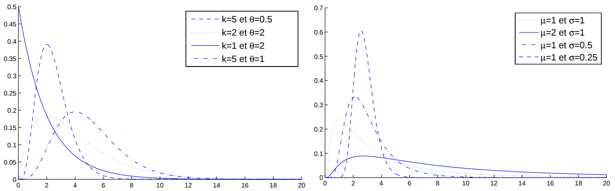
FIGURE 8.5 – Tracé des densités des distribution gamma f(x; k, \theta) = x^{k-1} \exp(-x/\theta) / (\Gamma(\theta) \theta^k) (à gauche) et des distributions log-normales f(x; \mu, \sigma) = \exp(-((\ln(x) - \mu)/\sigma)^2 / 2) / (x\sigma\sqrt{2\pi}) (à droite) pour quelques jeux de paramètres.
