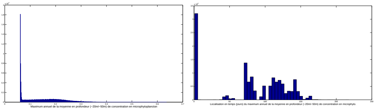
FIGURE 8.22 – Histogrammes représentant les valeurs (concentration en azote) (à gauche) et la localisation (jours) (à droite) du maximum annuel de concentration moyenne en mésophytoplancton entre -20m et -50m.
