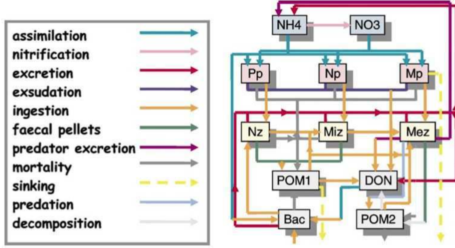
FIGURE 6.7 – Biogeochemical model (NH4 : Ammonium ; NO3 : nitrate ; Pp, Np, Mp : pico-, nano-, microphytoplankton ; Nz, Miz, Mez : nano-, micro-, mesozooplankton ; POM1, POM2 : type 1 and 2 particulate organic nitrogen ; Bac : bacteria ; DON : dissolved organic nitrogen).
