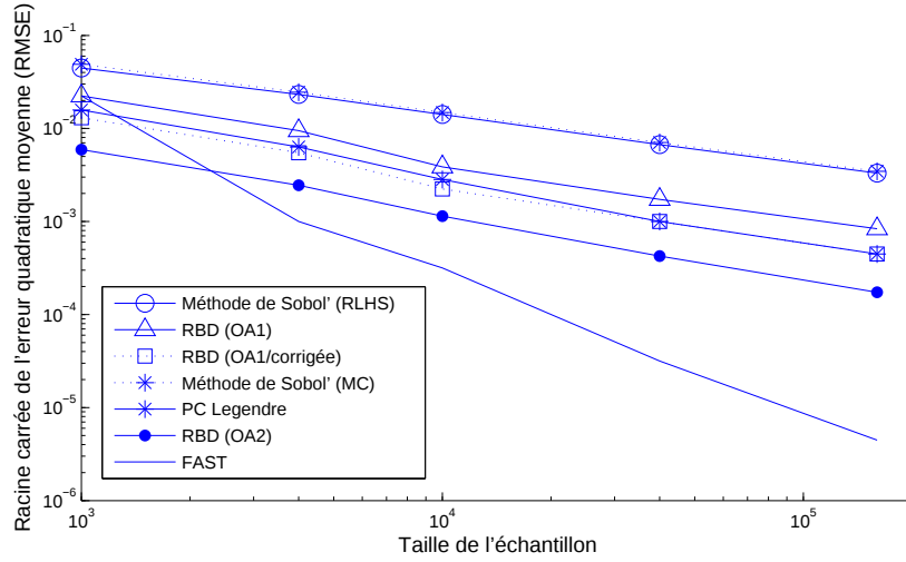
FIGURE 7.3 – Estimation des indices de Sobol' d'ordre 1 de la g-fonction ayant pour valeur 0.001.
