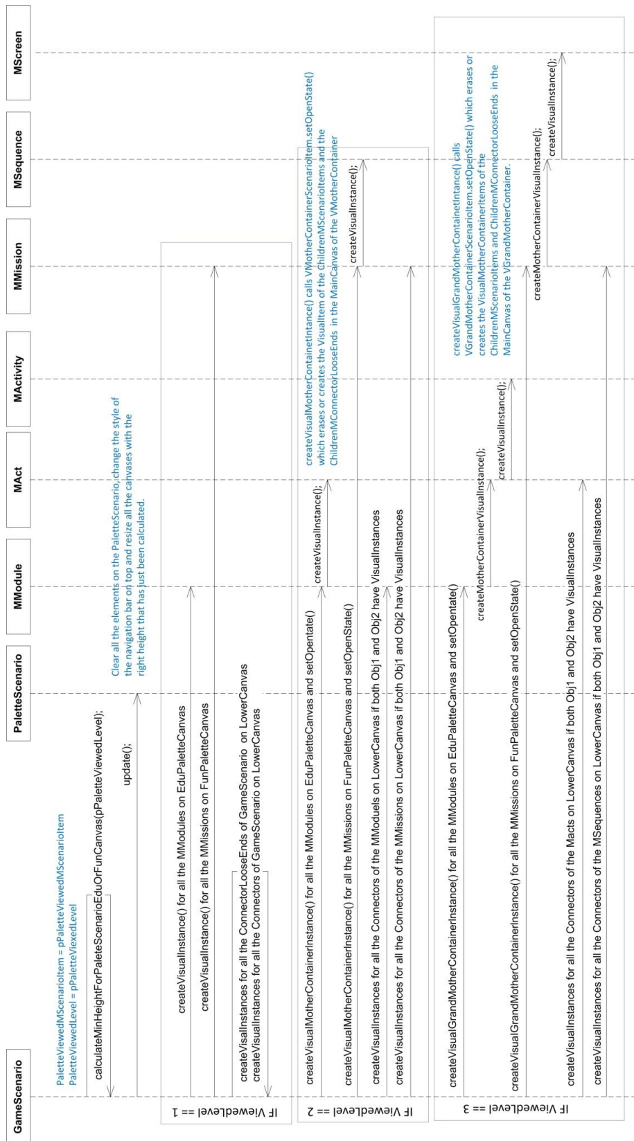
Fig 7 : Fonction ChangePaletteView()
