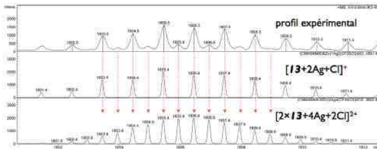
Figure 3-7. Profil isotopique du spectre ES-MS montrant la formation de la cage de coordination 14 .
