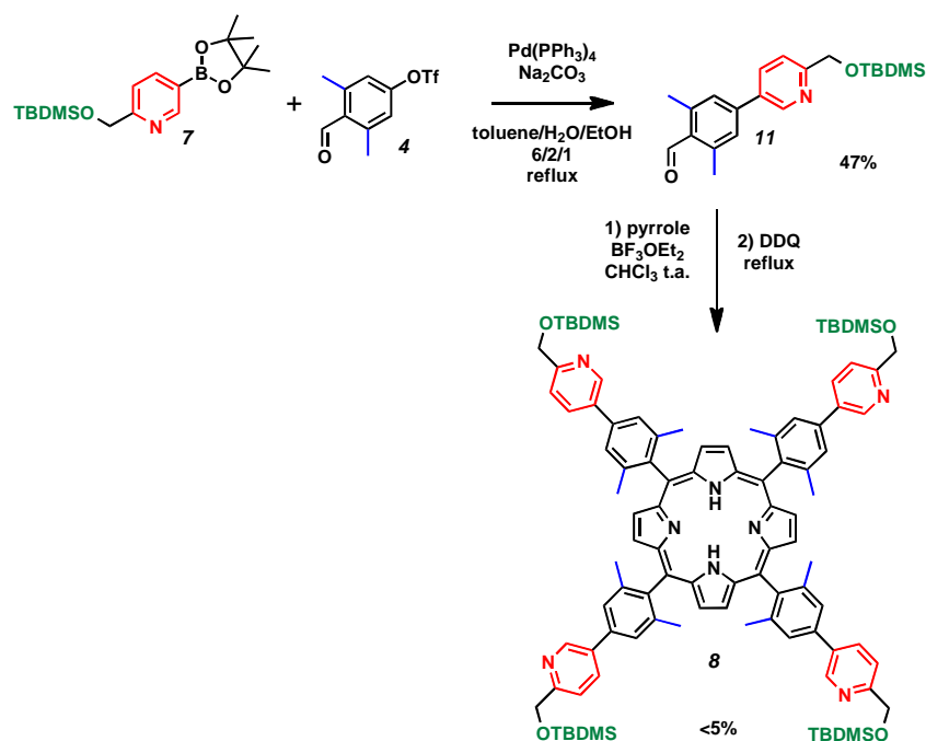
Figure 2-8. Synthèse directe de la porphyrine 8 par formation d'un formylbiaryl 11 .
