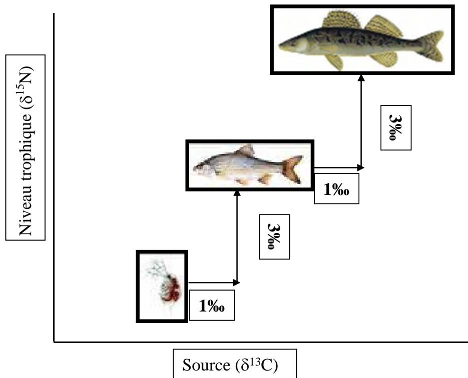
FIGURE II.2 – Reconstitution des relations trophiques grâce aux taux de fractionnement des isotopes stables du carbone et de l’azote, à travers un graphe \delta^{15}\text{N} - \delta^{13}\text{C} .
