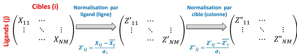
Figure 20 : Double transformation pour corriger et normaliser les scores d'arrimage brut. X_{ij} sont les scores d'arrimage brut. Z' et Z'' sont les scores-Z calculés pour chaque association. \sigma_j et \sigma_i correspondent aux déviations standards calculées pour les ligands j et les cibles i respectivement. N est le nombre total de ligands et M est le nombre total de cibles.
