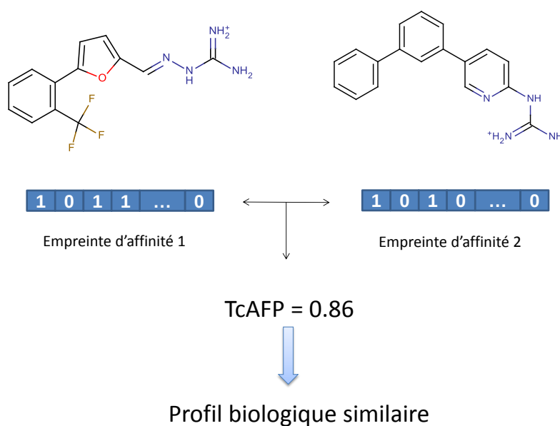
Figure 11 : Exemple de deux molécules possédant un profil biologique similaire (Tanimoto = 0.86 sur les empreintes d'affinités protéique) mais des faibles similarités structurales Tanimoto MACCS = 0.43 et Tanimoto ECFP_4 = 0.19
