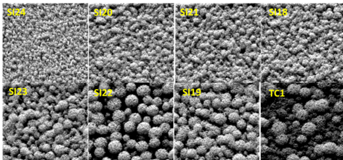
FIGURE 2.11 – Images panchromatiques ( 130m \times 130m ) simulées par le modèle DART/CESBIO à partir des maquettes de mangroves présentées dans la figure 2.5 et suivant la réponse du capteur Geosyde (angles solaires et de visée au zénith; d'après le projet TOSCA/CNES "FOTO-METRICS").
