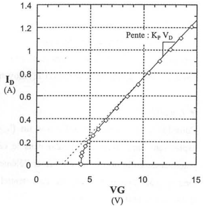
Figure 18 Tracé de I_D(V_G) à V_D=20mV . On voit que pour V_G suffisamment élevé, on tend vers une droite de pente K_P V_D mais pour laquelle on ne retrouve pas la tension de seuil par extrapolation. Les plots correspondent aux valeurs calculées à l'aide du modèle proposé paragraphe suivant.
