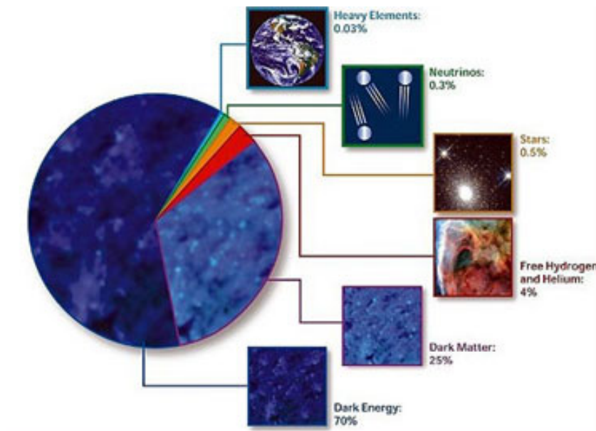
FIGURE 1.5 – Composition de l’Univers dans le modèle cosmologique \Lambda CDM (NASA).
