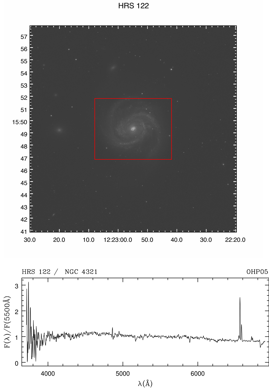
FIGURE 6.4 – Figures provenant de Boselli et al. (soumis). Figure du haut : Images SDSS en bande r de M 100 (HRS 122). En rouge la surface totale balayée par le spectromètre. Figure du bas : spectre normalisé à l'intensité moyenne entre 5400 et 5600 Å obtenu pour M 100 (HRS 122) entre 3600 Å et 6800 Å. La raie la plus importante à droite est la raie H \alpha entourée du doublet [NII].
