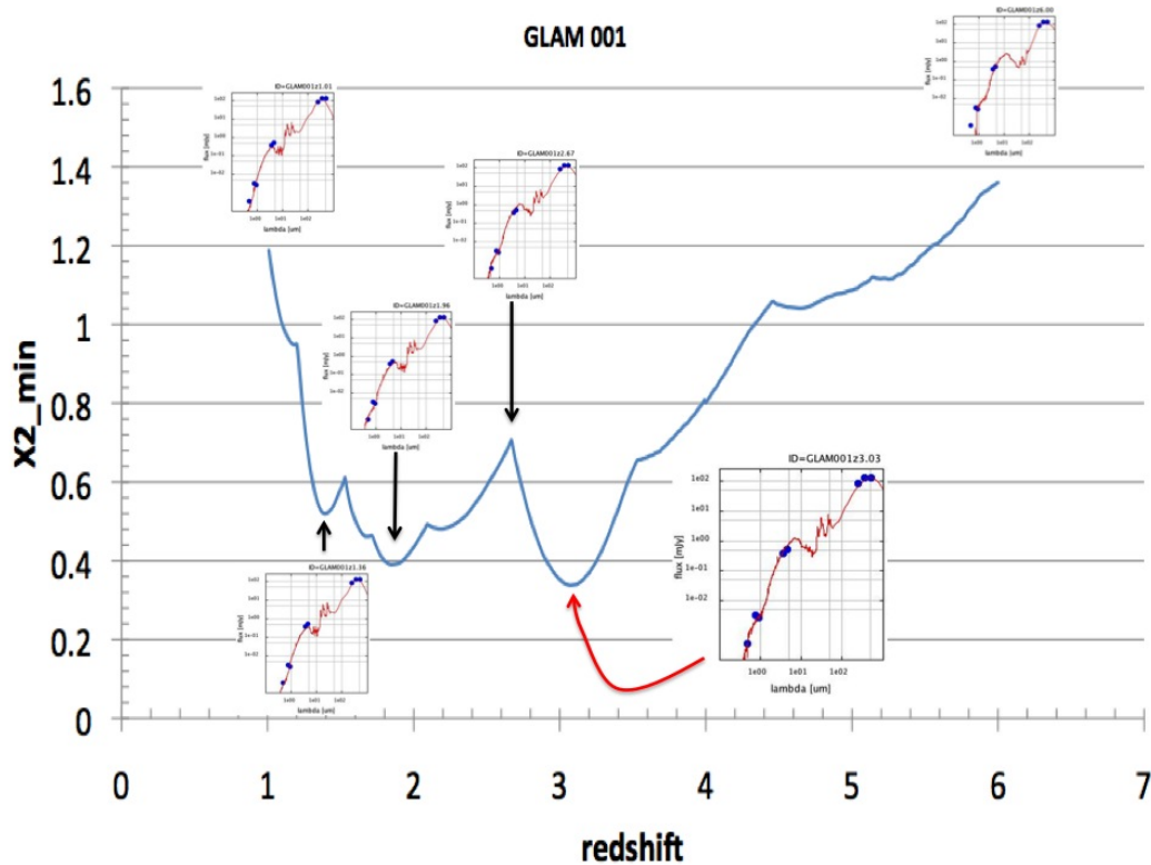
FIGURE A.8 – Ajustement de SED avec CIGALE. La courbe bleue correspond à la variation de \chi^2 en fonction du redshift. Les meilleures SED sont montrées, les points bleus correspondent aux données observationnelles ( g , i , z , 3.6, 4.5, 250, 350 and 500 \mu\text{m} ) et les courbes rouges sont les meilleurs modèles pour un redshift donné.
