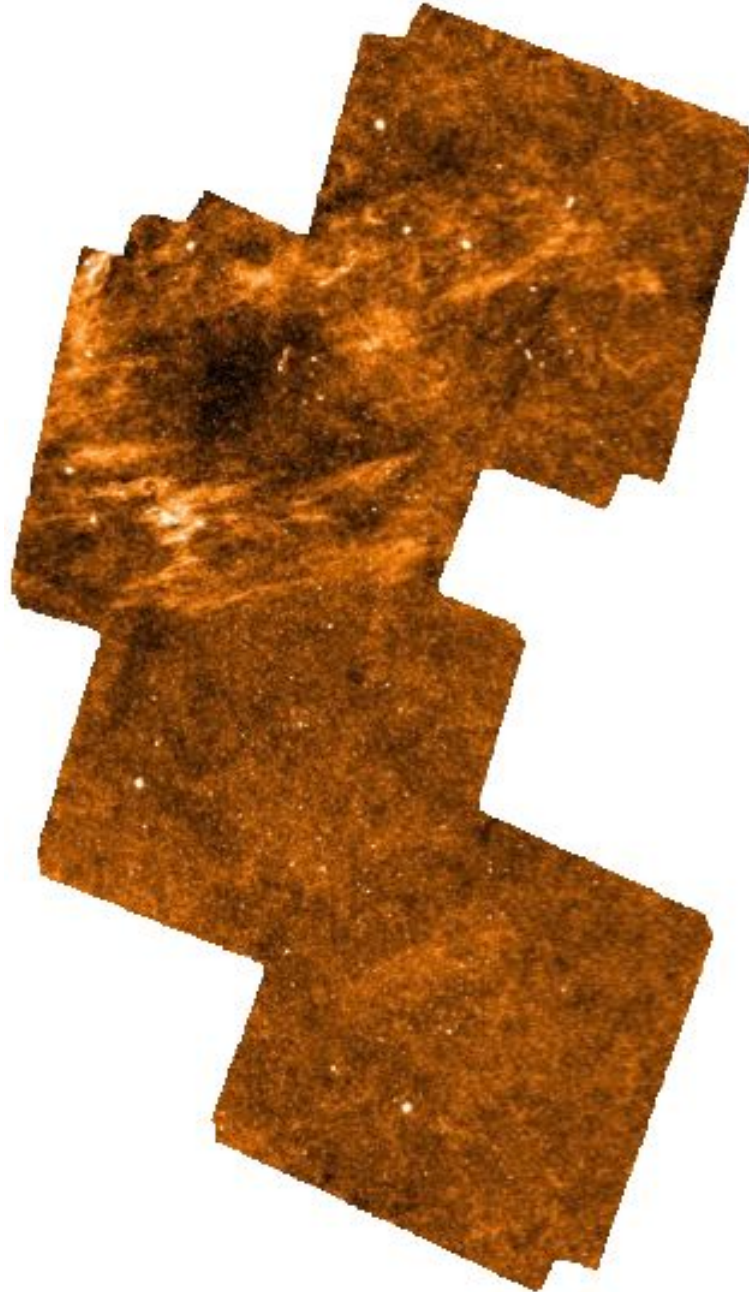
FIGURE 4.4 – Figure tirée de Davies et al. (2012) . Les quatre champs HeViCS couvrant une surface totale de 64^{\circ 2} à 250 \mu\text{m} . Les galaxies les plus brillantes sont visibles (points blancs), les traînées correspondent aux cirrus galactiques.
