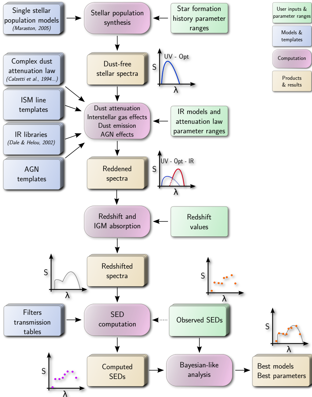
FIGURE 2.11 – Figure tirée de Roehly et al. (2011). Schéma d'exécution du programme CIGALE.
