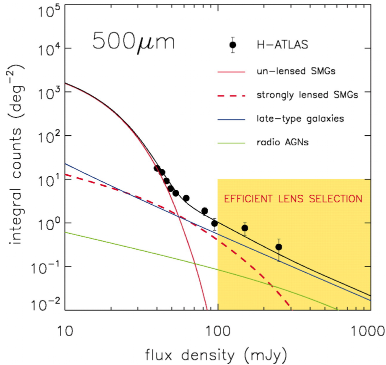
FIGURE A.9 – Figure tirée de Negrello et al. (2010) . Sélection des lentilles gravitationnelles à 500 \mu\text{m} . Les comptages à 500 \mu\text{m} voient la contribution de plusieurs populations : les galaxies submillimétriques à haut redshifts, les galaxies proches de types tardifs, et les galaxies radio alimentées par un AGN.
