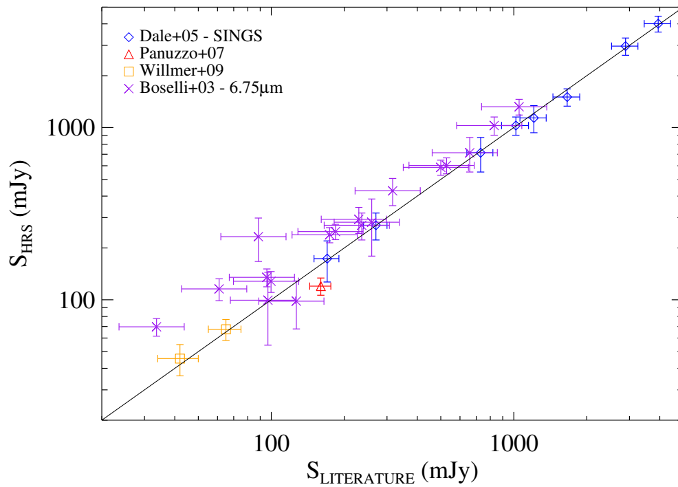
FIGURE 6.2 – Comparaison entre les densités de flux Spitzer /IRAC mesurées et les densités de flux Spitzer /IRAC et ISO (6.75 \mu\text{m} ) disponibles dans la littérature pour certaines galaxies.
