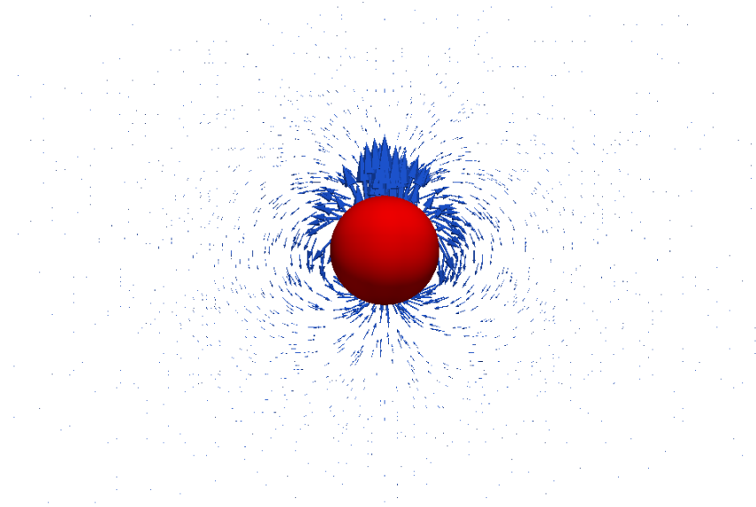
FIGURE 8.13 – Champ de vitesse d'un squirmer seul
