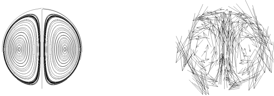
FIGURE 5.11 – Lignes de courant et champ de vitesse du contrôle dans le cas de deux particules éloignées
