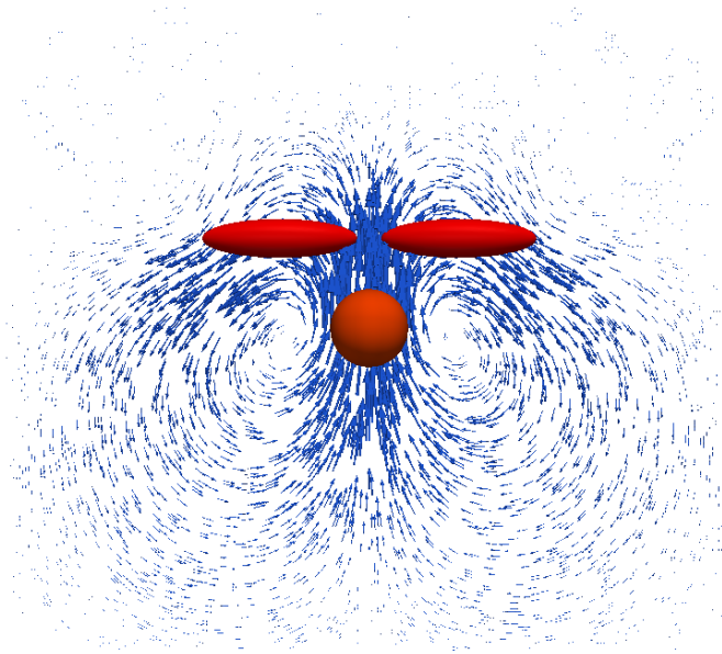
FIGURE 8.10 – Champ de vitesse d'un puller
