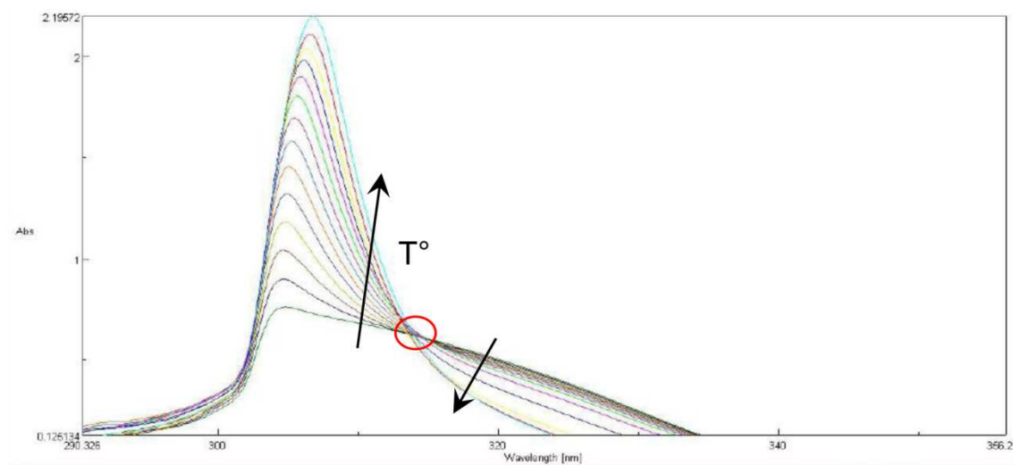
Image VI-10 : Spectroscopie UV/Visible à différentes températures d'une solution de Bis-C3 dans du trichlorobenzène
