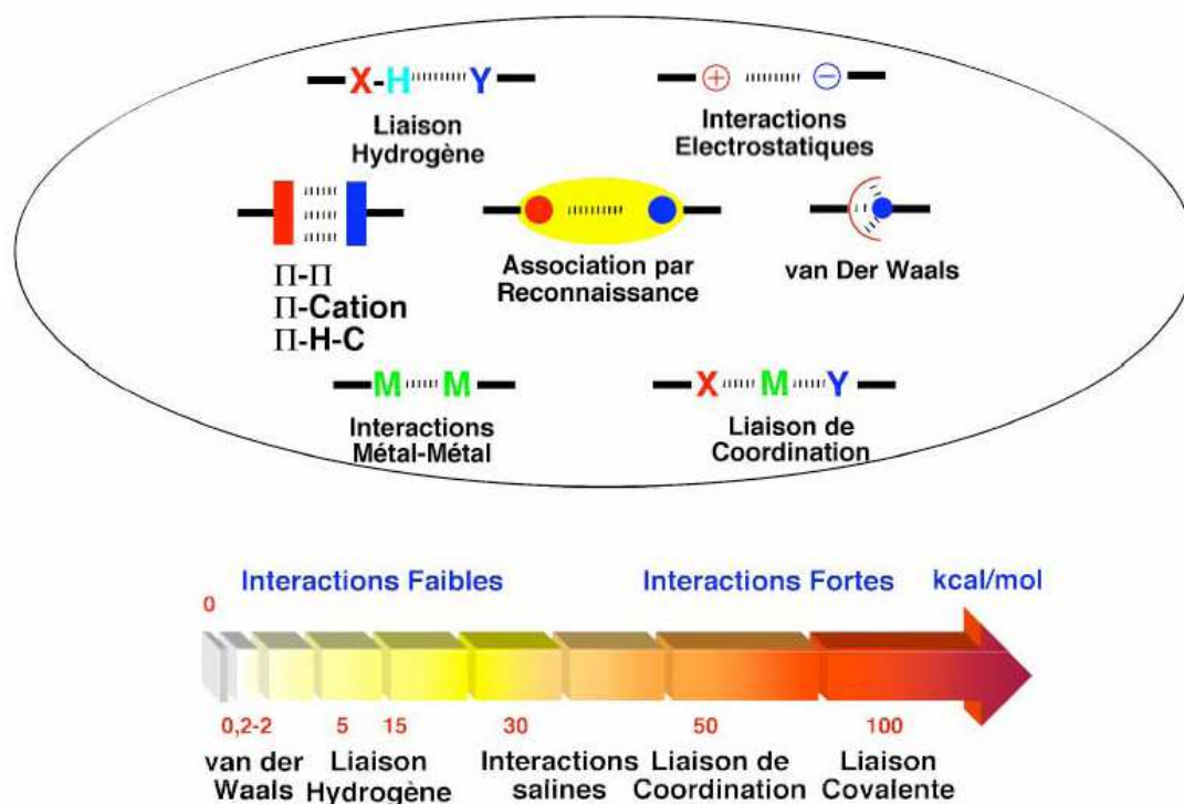
Image I-1 : Différents types d'interactions supramoléculaires et leurs énergies respectives par rapport à celle d'une liaison covalente
