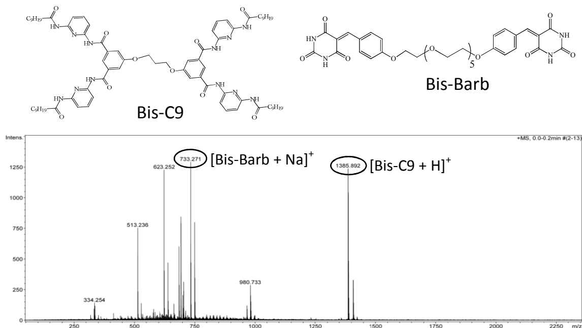
Image III-25 : En haut, représentation des monomères Bis-C9 et Bis-Barb ; en bas, spectre de masse ESI (mode positif) du mélange de Bis-C9 et Bis-Barb à 5 mM dans C_2D_2Cl_4
