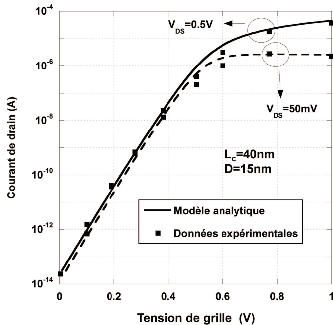
FIGURE 7.10: Courant de drain en fonction de la tension de grille pour un transistor MOSFET à nanofil de diamètre 15nm et de canal 40nm ; Comparaison entre le modèle analytique et des données expérimentales.
