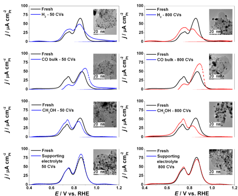
Figure 5. Voltampéromes d'électroxydation de \text{CO}_{\text{ads}} mesurés sur Pt/Vulcan XC 72(40 wt. %) avant/après 50 ou 800 cycles entre 0,05 et 1,23 V vs RHE dans des solutions contenant de l'hydrogène, du monoxyde de carbone ou du méthanol. Les encarts montrent des images MET représentatives du catalyseur après 50 ou 800 cycles de potentiel. Electrolyte: 0,1 M \text{HClO}_4 , \nu = 0,020 \text{ V s}^{-1} , T = 20 \text{ }^\circ\text{C} .
