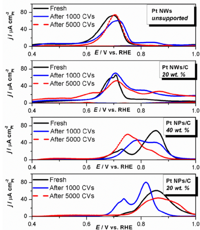
Figure 15. Voltampérométries d'électrooxydation de \text{CO}_{\text{ads}} mesurées sur des nanofils de Pt supportés ou non sur Vulcan XC72 et sur des électrocatalyseurs de référence Pt/Vulcan XC 72 20 et 40 wt. % après un test de vieillissement réalisé dans 0,1 M \text{HClO}_4 , à \nu = 0,2 \text{ V s}^{-1} et T = 60 \text{ }^\circ\text{C} .
