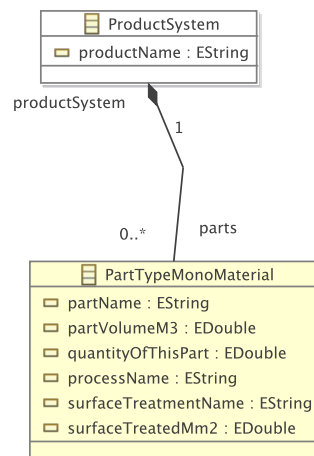
FIGURE A.11 – Exemple de méta-modèle des données de sortie de l'activité de CAO
