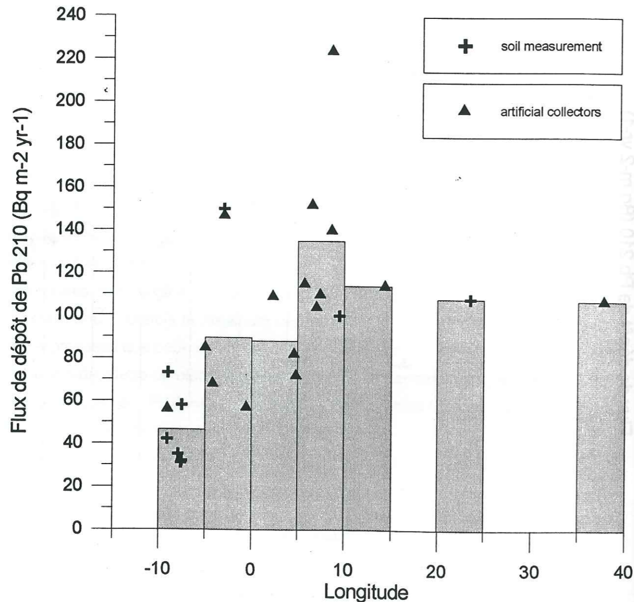
Figure IV.7: Distribution en longitude du flux de dépôt annuel de ^{210}\text{Pb} (en \text{Bq m}^{-2} \text{an}^{-1} ) en Europe, entre 30^\circ et 60^\circ\text{N} ; Les barres grises représentent les moyennes de flux par bande de 5^\circ de longitude.
