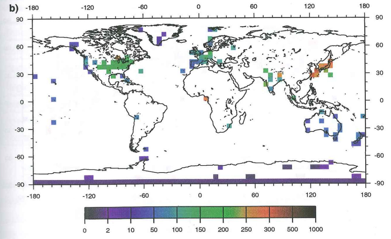
Figure IV.14: La base de données synthétisée; (a) concentration de plomb 210 dans l'air de surface (en mBq SCM-1); (b) flux de dépôt de plomb 210 (en Bq m -2 an -1 ).
