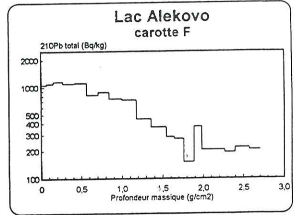
Figure 2. Profil de ^{210}\text{Pb} total dans les sédiments
