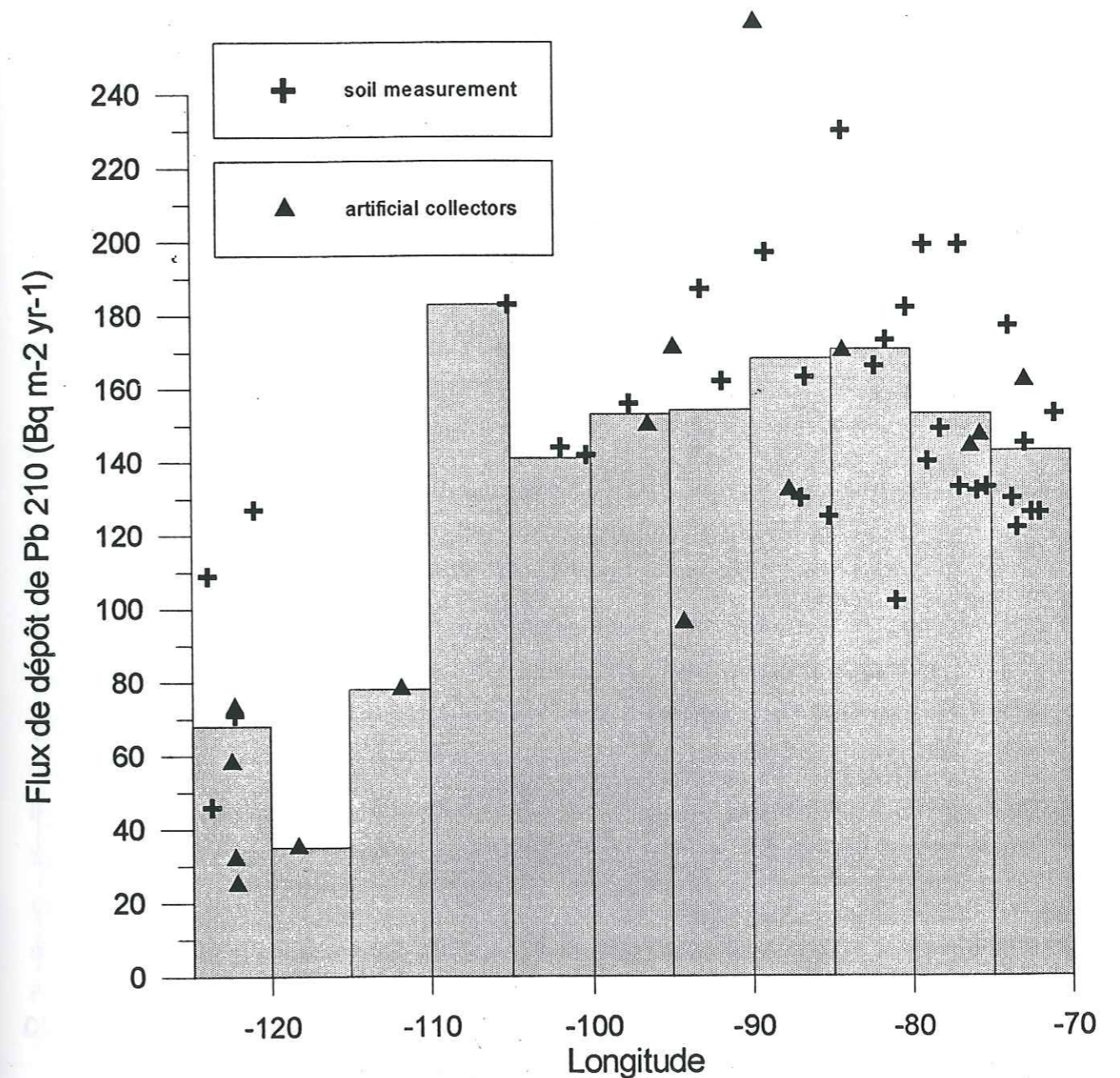
Figure IV.6: Distribution en longitude du flux de dépôt annuel de ^{210}\text{Pb} (en \text{Bq m}^{-2} \text{ an}^{-1} ) en Amérique du Nord, entre 30^\circ et 60^\circ\text{N} ; Les barres grises représentent les moyennes de flux par bande de 5^\circ de longitude.
