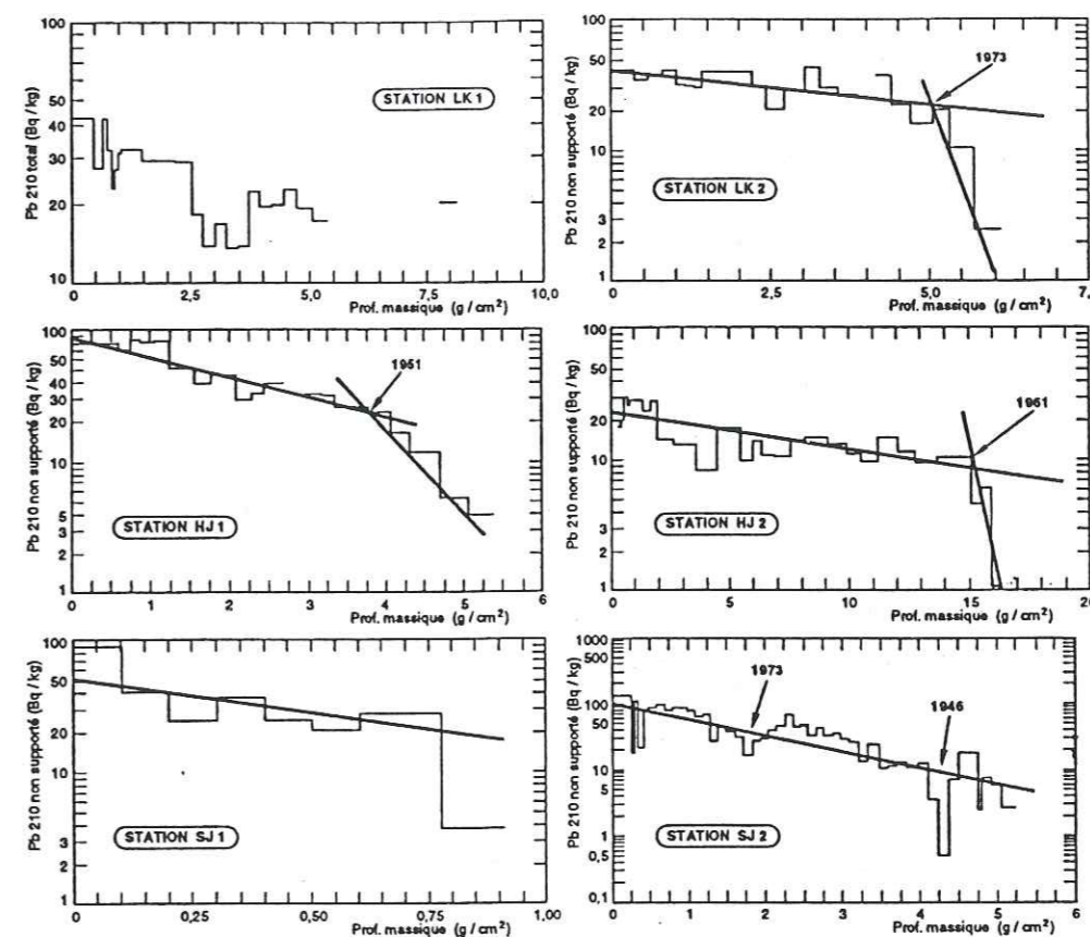
Figure 3 Variations du 210 Pb en fonction de la profondeur pour l'ensemble des stations étudiées. 210 Pb versus depth for all stations.
