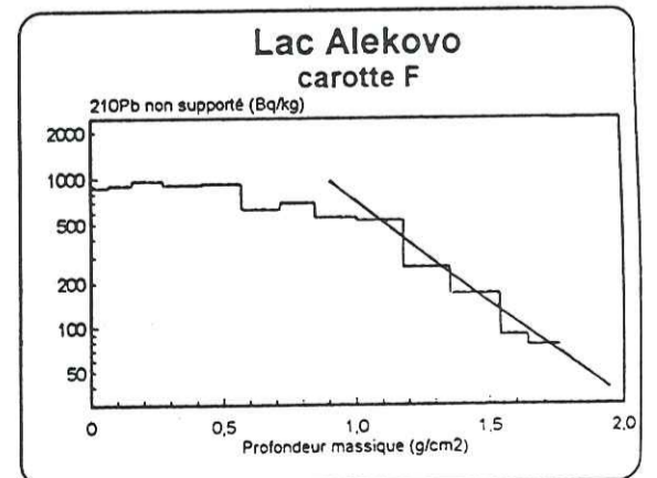
Figure 3. Profil de ^{210}\text{Pb} non supporté dans les sédiments
