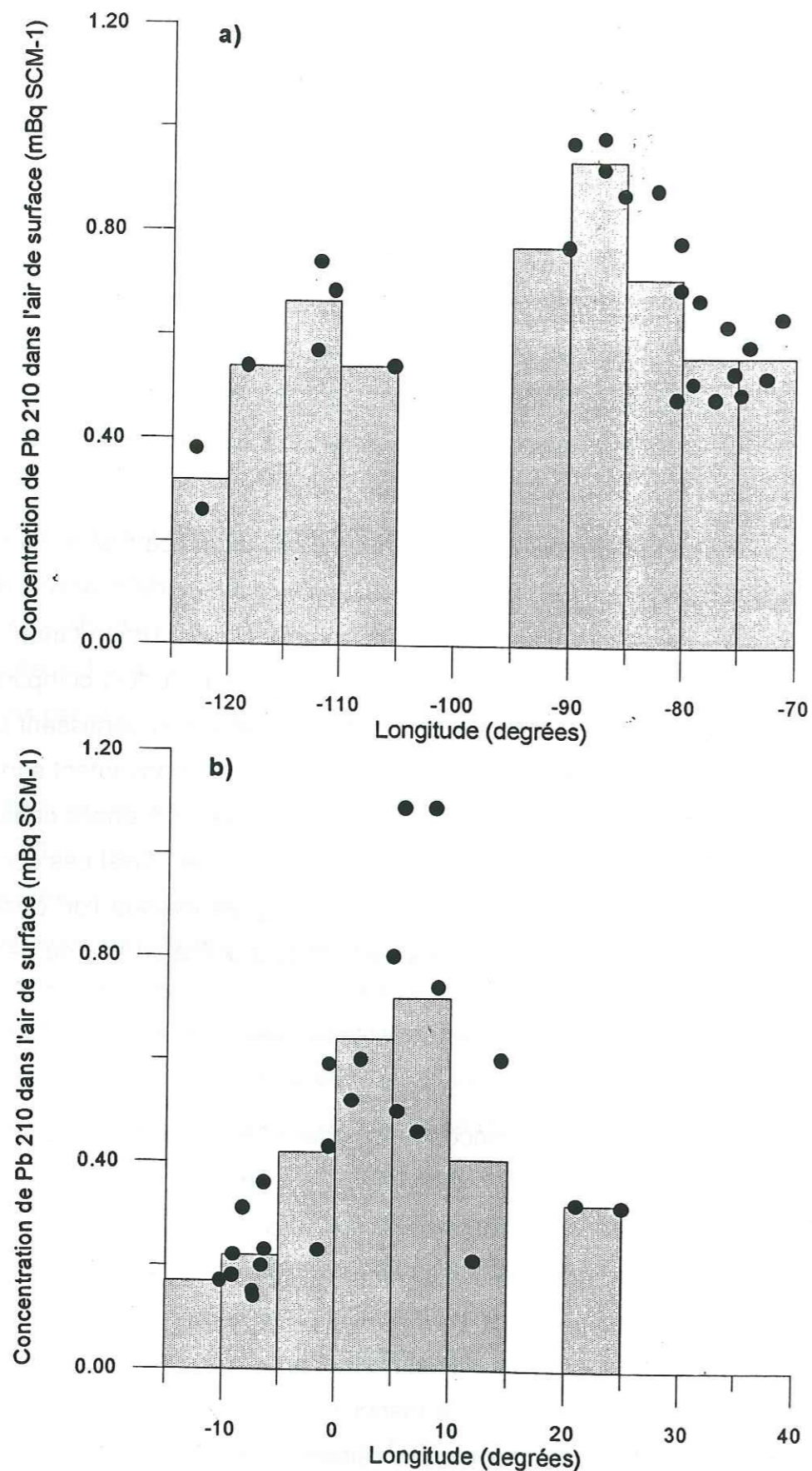
Figure IV.1: Distribution en longitude de la concentration de 210 Pb dans l'air de surface (en mBq SCM -1 ) (a) en Amérique du Nord et (b) en Europe, entre 30°N et 60°N; Les barres grises représentent les moyennes de concentration par bande de 5° de longitude
