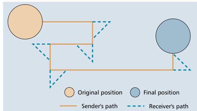
FIGURE 2.10 – Un exemple de dead-reckoning [Joslin et al. , 2004].
