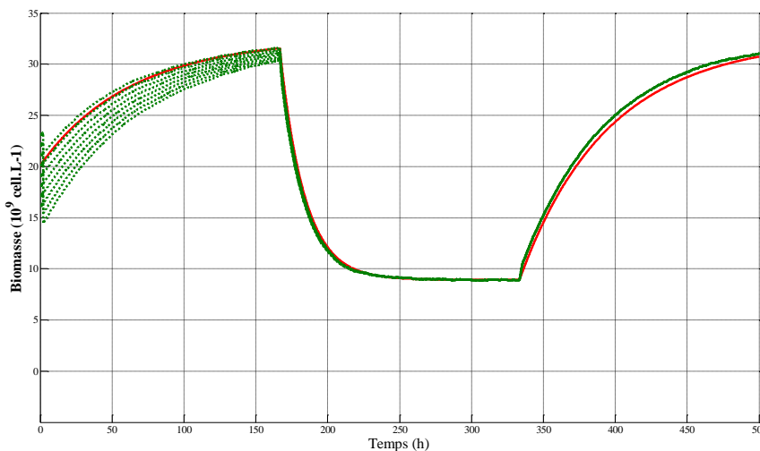
Figure 4.9 : Observateur asymptotique : Estimation de la concentration de biomasse avec une désadaptation de l’initialisation, cas nominal (modèle en trait plein, estimations en trait discontinu)
