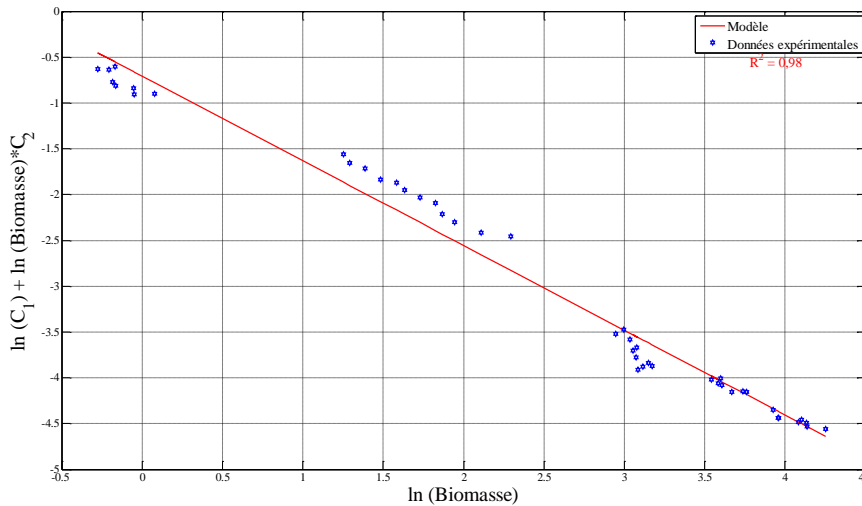
Figure 3.9 : Identification des coefficients C_1 et C_2
