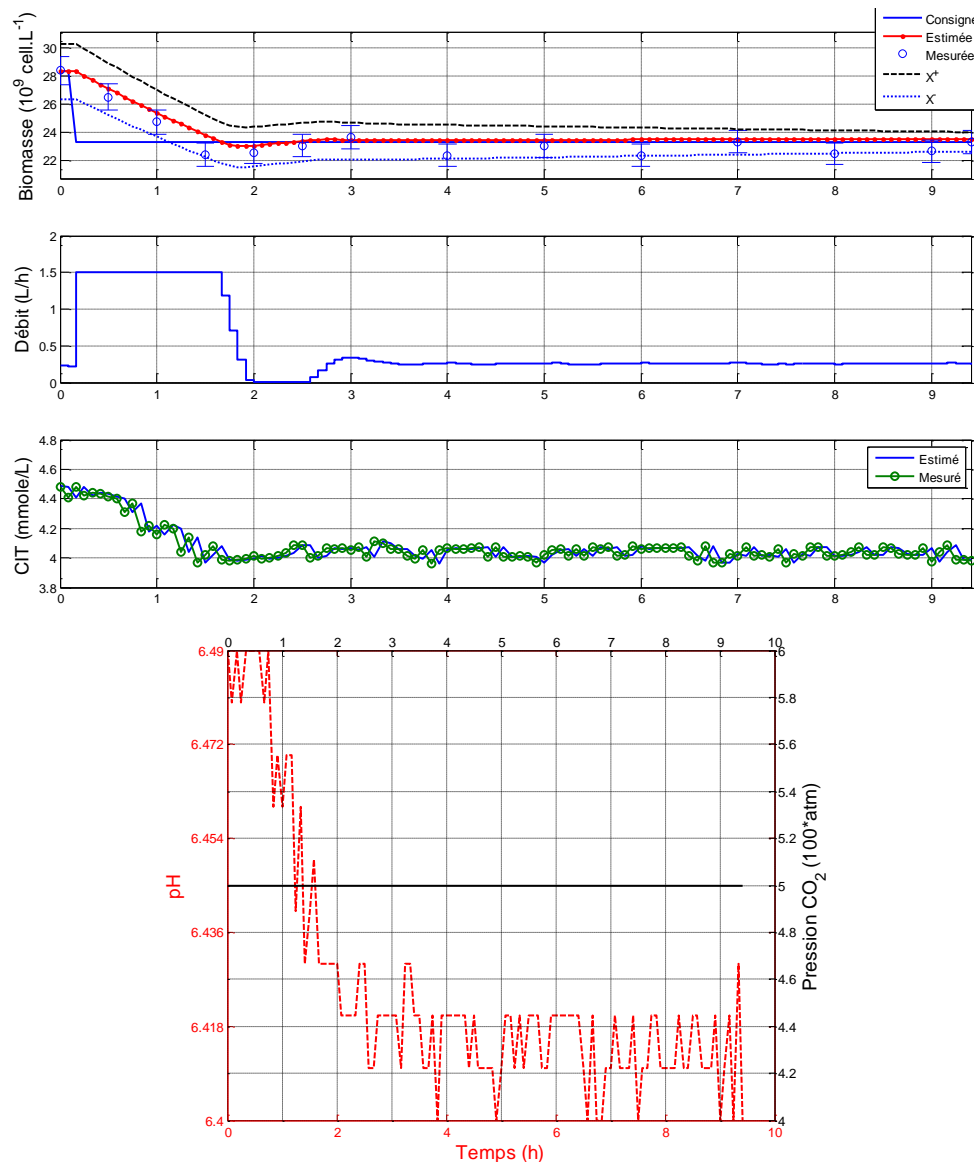
Figure 5.22 : Commande GMC couplée à l'observateur par intervalles pour un échelon de consigne de 28,3 à 23,3 \text{ } 10^9 \text{ cell. L}^{-1} à t = 30 \text{ mn}
