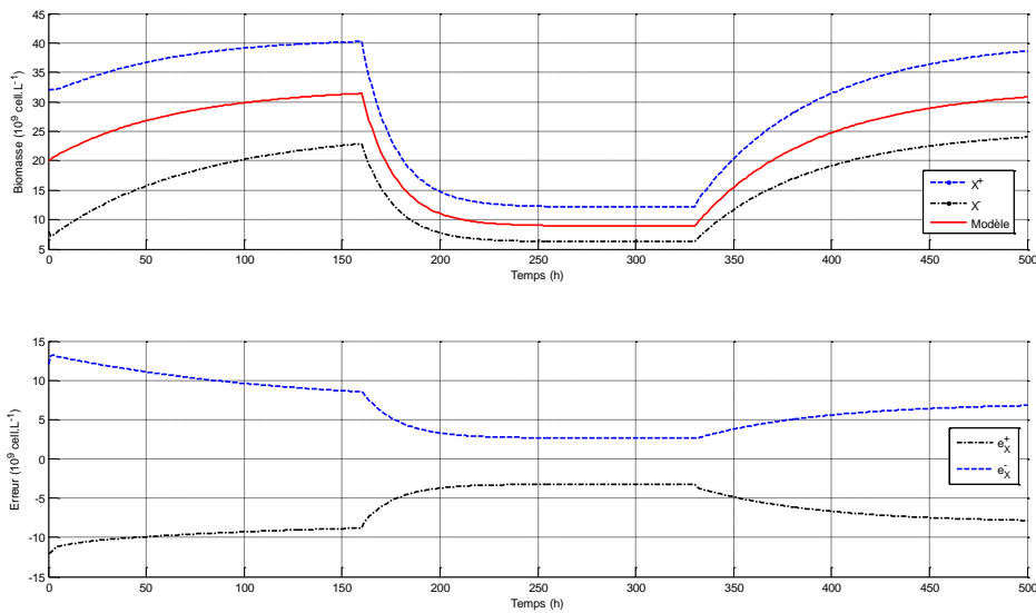
Figure 4.22 : Analyse de la robustesse de l’observateur par intervalles : estimation de la concentration de biomasse et erreur d’estimation avec des incertitudes de 20% sur k_{LA} et Y_{X/CIT}
