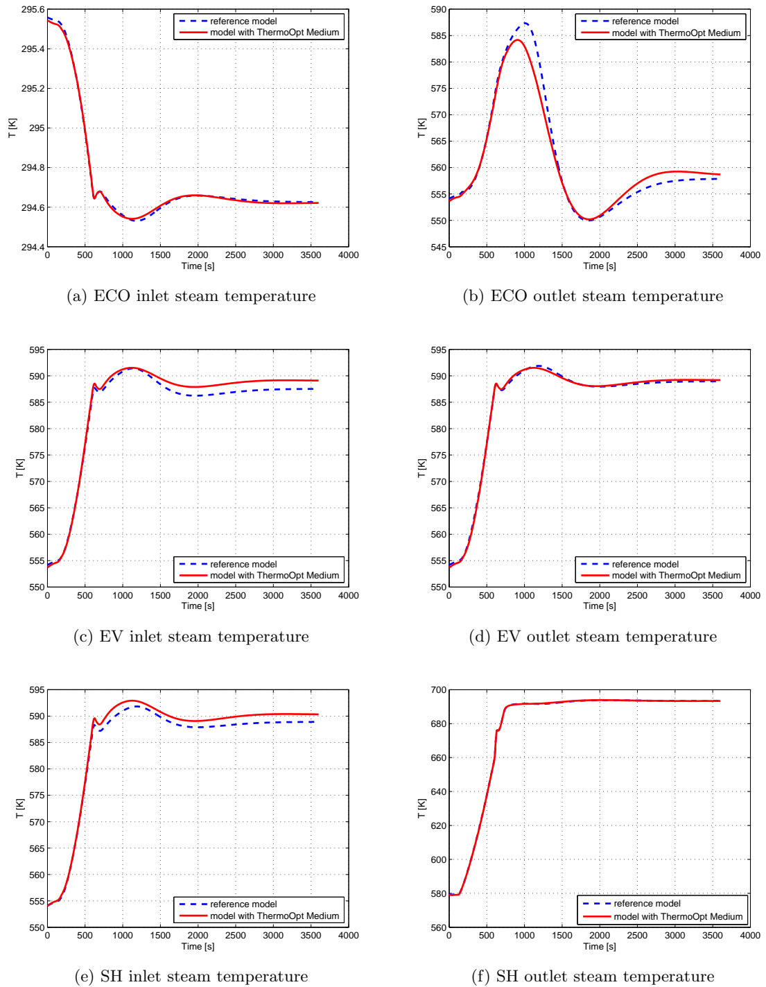
Figure 4.12: Validation Scenario I: steam temperature in HRSG
