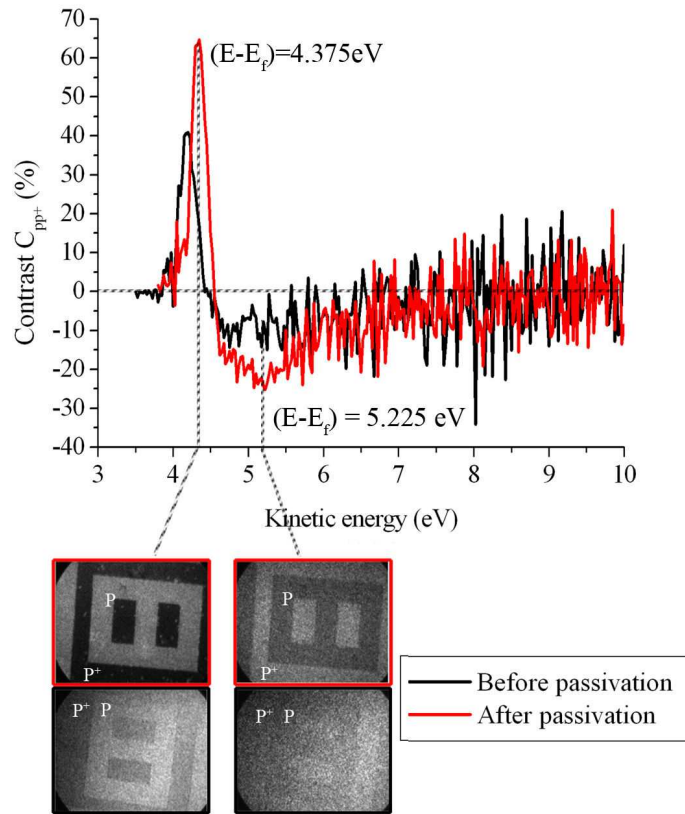
Figure 6.11: Evolution du contraste C_{P/P+} en fonction de l'énergie cinétique des électrons secondaires avant et après passivation. Les images présentées ont été extraites des séries à deux énergies cinétiques : (E-E_f)=4.375 eV and 5.225 eV.
