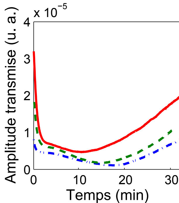
FIGURE 6.2 – Aire sous l'enveloppe en fonction de temps avec différentes fractions liquides \phi_\ell , mousse de laponite avec le gaz C_2F_6 . La distance d est fixe, d = 2 mm. \phi_\ell = 3\% (ligne en tirets pointillés), \phi_\ell = 5\% (ligne en tirets) et \phi_\ell = 8\% (ligne simple).
