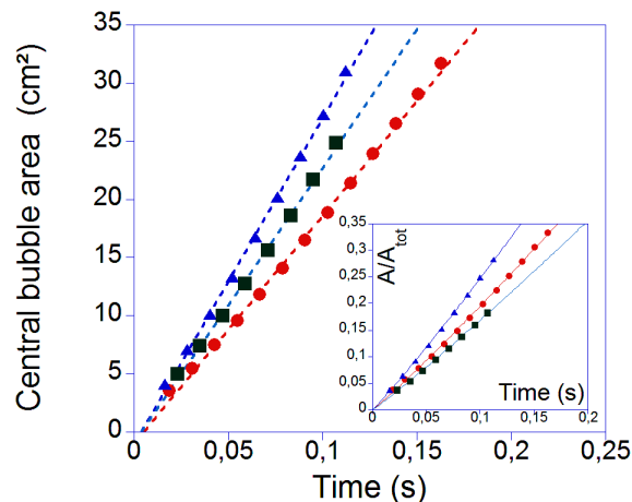
FIGURE 3.15 – Exemples de l'évolution temporelle de l'aire de la bulle centrale A(t) dans le régime gonflage pur. \bullet : P_0 = 403 Pa, L = 0.33 cm, A_{\text{tot}} = 95 cm 2 , e = 0.06 cm, a = 0.019 cm ; \blacksquare : P_0 = 630 Pa, L = 0.15 cm, A_{\text{tot}} = 110 cm 2 , e = 0.04 cm, a = 0.021 cm ; \blacktriangle : P_0 = 750 Pa, L = 0.13 cm, A_{\text{tot}} = 136 cm 2 , e = 0.06 cm, a = 0.022 cm. Les lignes en pointillés sont des ajustements avec une équation linéaire, avec t = 0 s correspondant au début de gonflage. Insert : évolution temporelle renormalisée de l'aire A(t)/A_{\text{tot}} avec un ajustement par l'équation (4.13).
