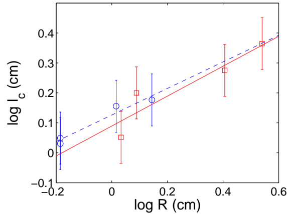
FIGURE 3.20 – Largeur de doigt en fonction du rayon effectif de la bulle centrale R = \sqrt{A/\pi} , avec les paramètres : (( \square )) e = 0,06 cm, L = 0,148 \pm 0,011 cm, dA/dt = 234 \pm 21 cm 2 /s; ( \circ ) e = 0,06 cm, L = 0,334 \pm 0,004 cm, dA/dt = 196 \pm 1 cm 2 /s. Les points expérimentaux ( \square ) sont ajustés par une droite avec une loi de puissance 0,50 \pm 0,15 , et les points ( \circ ) avec 0,44 \pm 0,08 .
