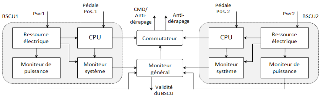
Figure V.3 : Système BSCU
