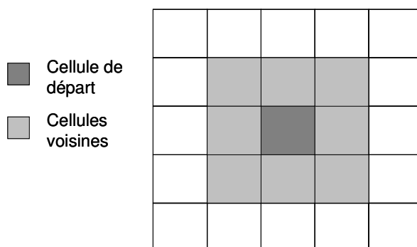
Figure IV.7.2 : Représentation de la structure du voisinage de type Moore, utilisée pour les déplacements des individus en recherche d'hôtes.
