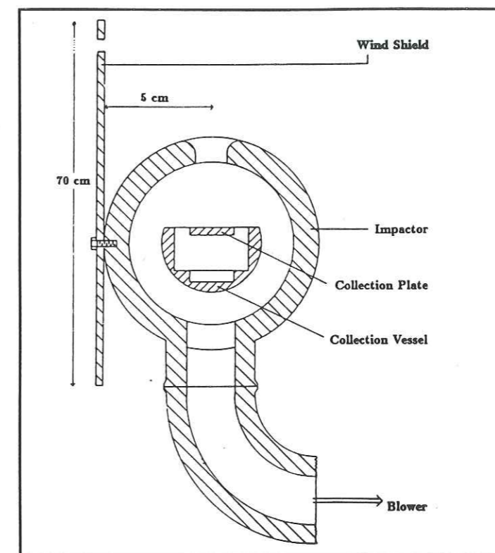
Figure 5.2: Coupe du dispositif de prélèvement des gouttelettes d'eau des nuages (d'après Kruisz et al., 1993).
