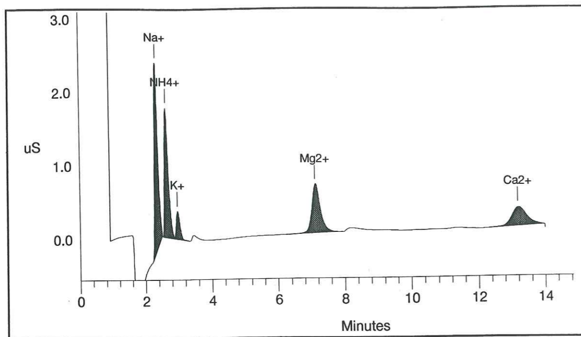
Figure 3.20: Exemple de chromatogramme obtenu avec une colonne CS10. Na^+ : 26 ng.g^{-1} , NH_4^+ : 16 ng.g^{-1} , K^+ : 8 ng.g^{-1} , Mg^{2+} : 8 ng.g^{-1} , Ca^{2+} : 8 ng.g^{-1} .
