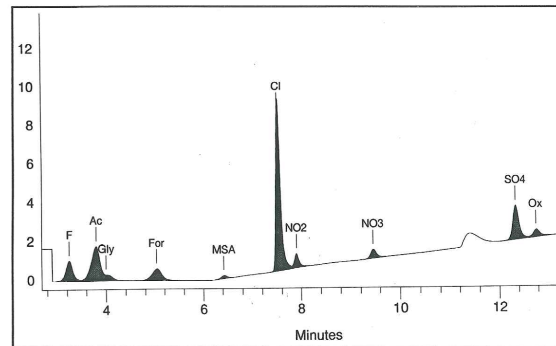
Figure 3.12: Chromatogramme obtenu avec une colonne AS5.
