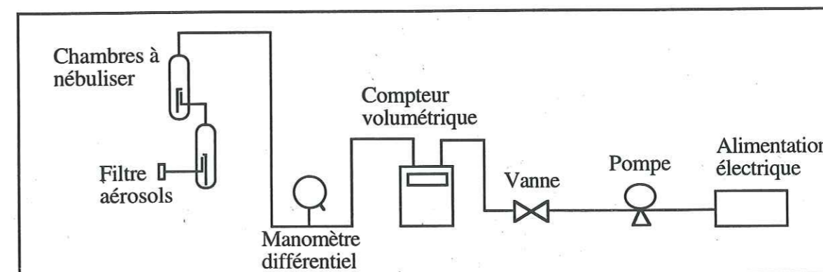
Figure 3.9: Ligne de prélèvement des chambres à brouillard.
