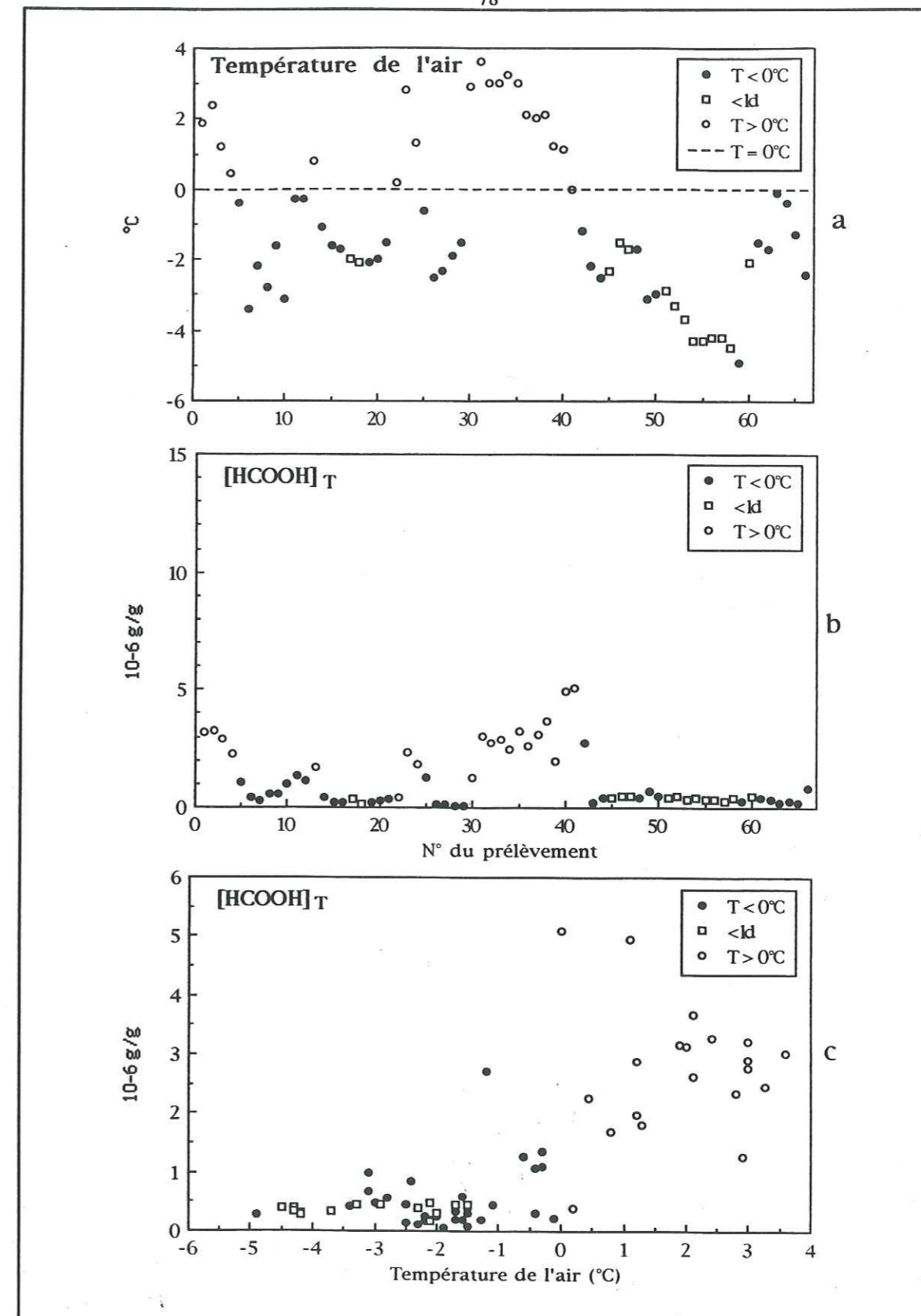
Figures 5.4: a- Moyenne de la température de l'air T durant chaque prélèvement, b- concentration en formiate dans l'eau récoltée [HCOOH]_T , c- [HCOOH]_T en fonction de T . Les concentrations sont exprimées en \mu g \cdot g^{-1} .
