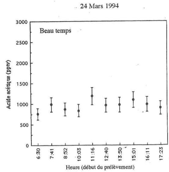
Figures A2: Suivis journaliers des concentrations atmosphériques d'acide acétique (exprimées en pptv) sur le campus de Saint-Martin d'Hères (Isère).
