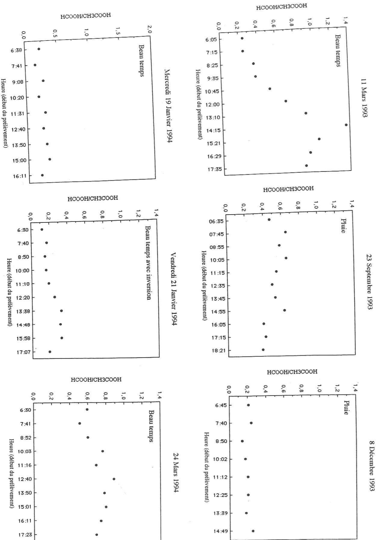
Figures A3: Suivis journaliers du rapport des concentrations [HCOOH]/[CH3COOH] sur le campus de Saint-Martin d'Hères (Isère).
