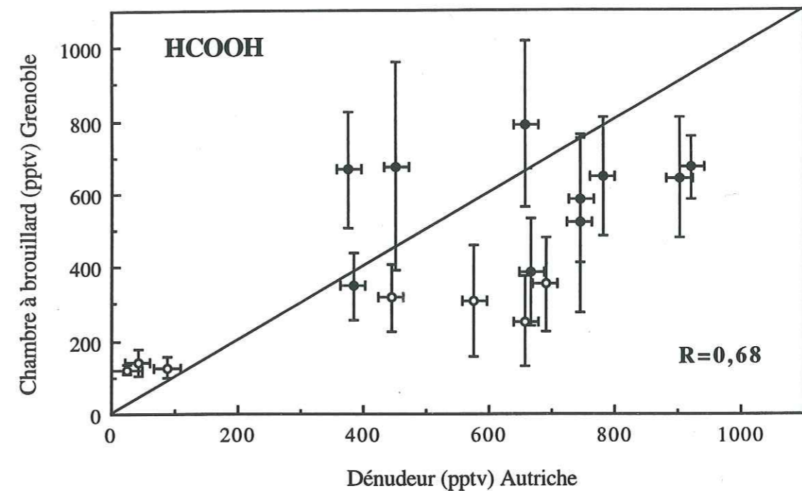
Figure 4.4: Comparaison entre les teneurs en \text{HCOOH} mesurées à Sönnblick sur les tubes dénudeurs (par les Autrichiens) et dans la chambre à brouillard (ce travail). (●): toutes les mesures composant la moyenne sont supérieures ou égales à la limite de détection, (○): une mesure au moins est inférieure à la limite de détection.
