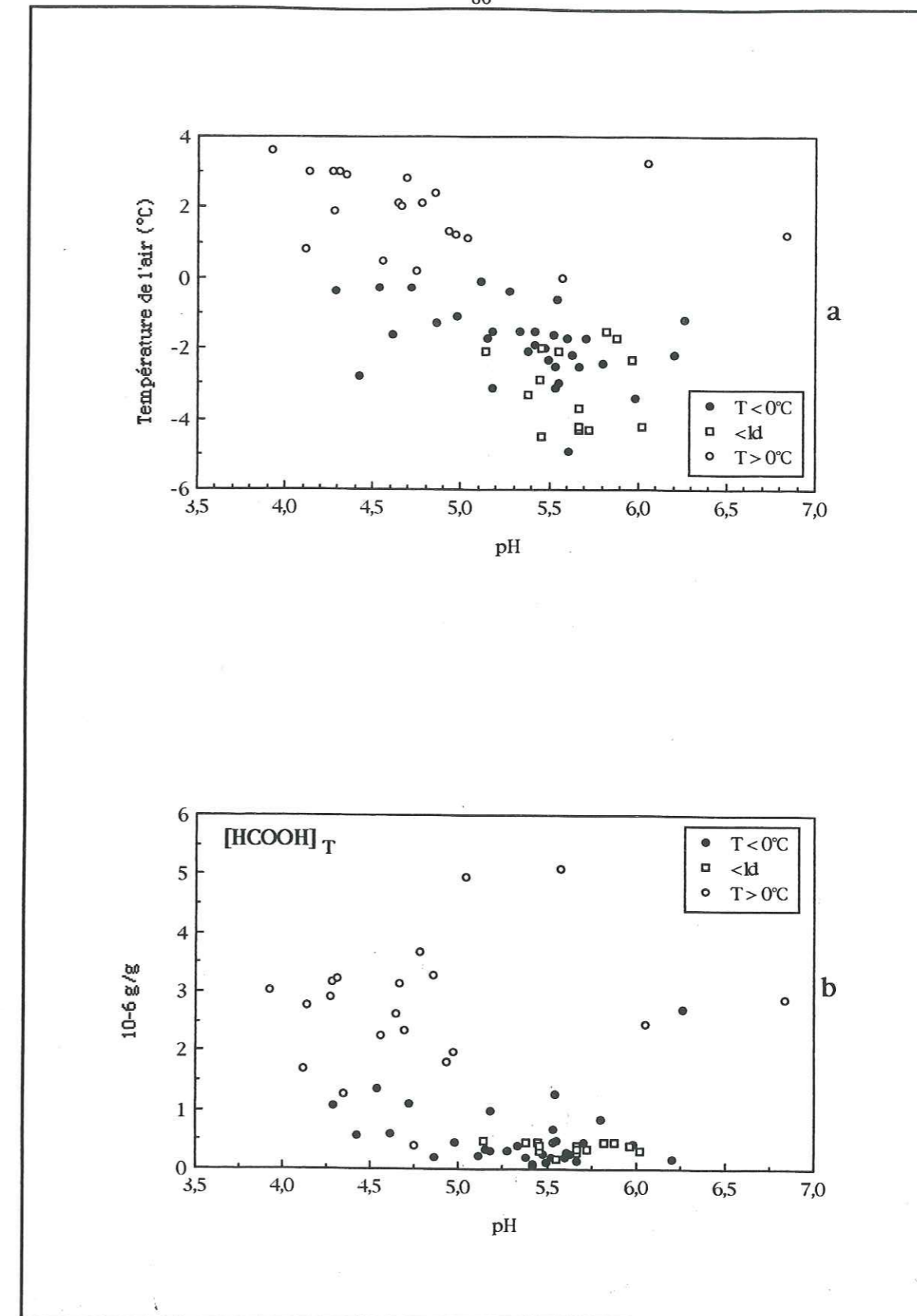
Figures 5.5: Température de l'air T en ^\circ\text{C} (a) et [\text{HCOOH}]_T exprimée en \mu\text{g}\cdot\text{g}^{-1} (b), en fonction du pH de l'échantillon.
