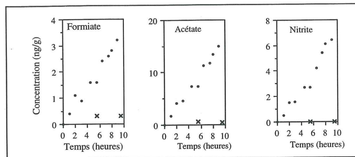
Figure 3.1: Evolution en fonction du temps des concentrations en \text{HCOO}^- , \text{CH}_3\text{COO}^- et \text{NO}_2^- de piluliers remplis d'eau ultra-pure en échange (·) ou non (x) avec l'atmosphère d'une salle sans poussières dans une hotte à flux laminaire.
