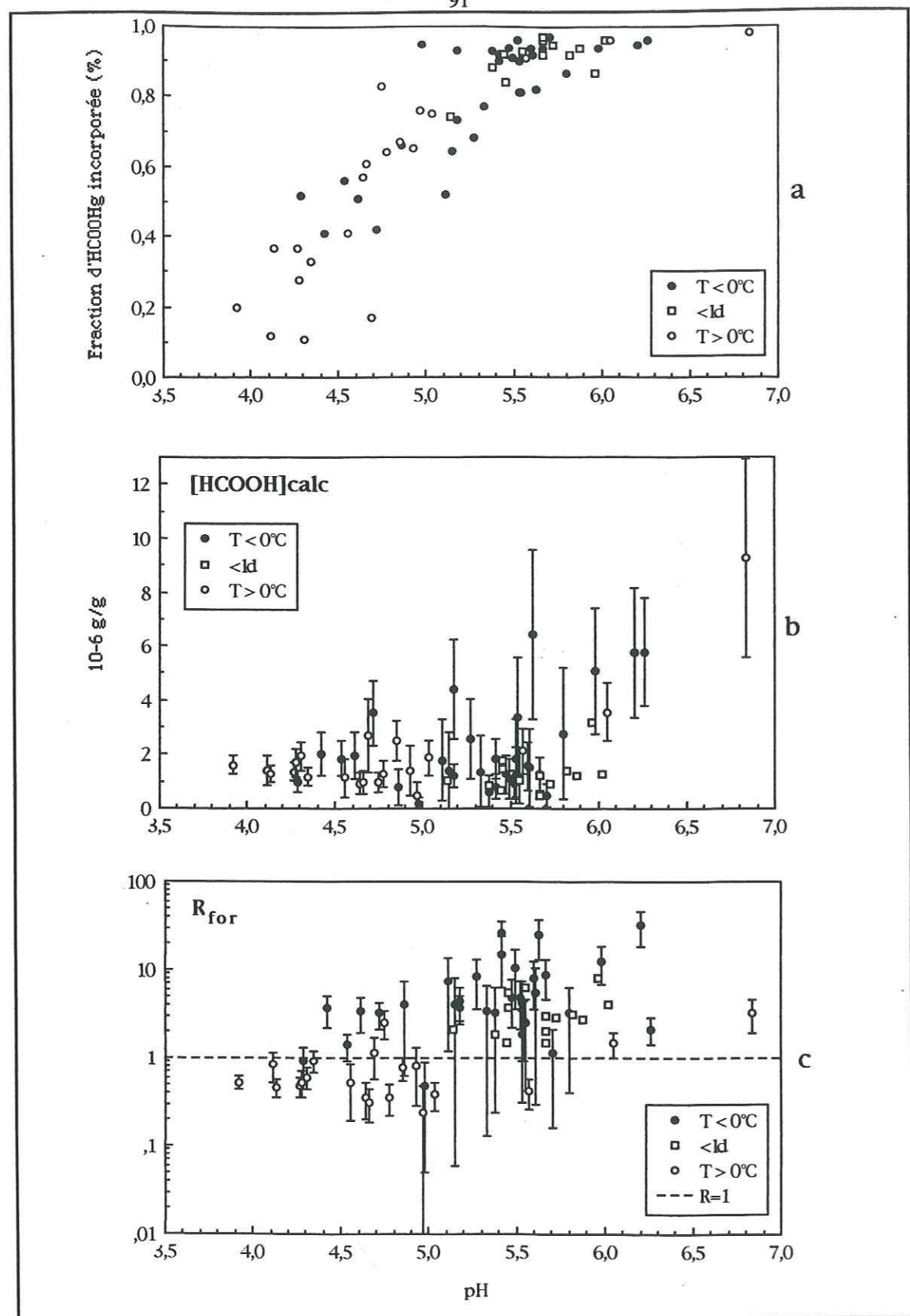
Figures 5.9: Fraction \epsilon d'HCOOH g incorporée en phase aqueuse (a), [HCOOH] calc ( \mu\text{g}\cdot\text{g}^{-1} ), b) et écart à la loi de Henry R_{\text{for}} (c), en fonction du pH des échantillons.
