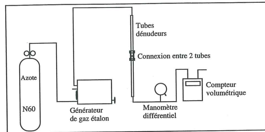
Figure 3.16: Dispositif expérimental pour la calibration des dénudeurs.
