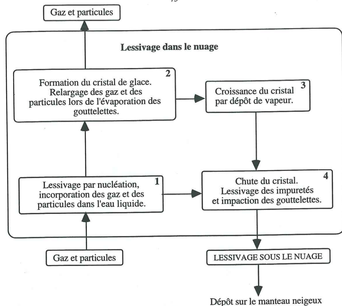
Figure 5.1: Lessivage des impuretés lors de la formation et de la sédimentation des cristaux de glace.
