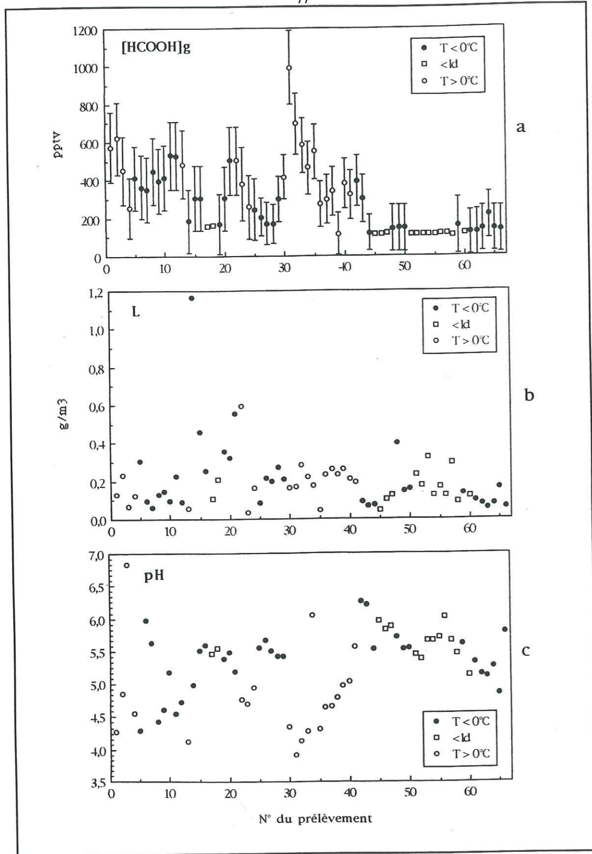
Figures 5.3: a- Concentrations en acide formique dans la phase gazeuse [HCOOH]_g (pptv), b- Moyennes sur la durée du prélèvement de la teneur en eau du nuage L ( g \cdot m^{-3} ), c- pH de la solution d'eau récoltée.
