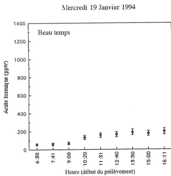
Figures A1: Suivis journaliers des concentrations atmosphériques d'acide formique (exprimées en pptv) sur le campus de Saint-Martin d'Hères (Isère).
