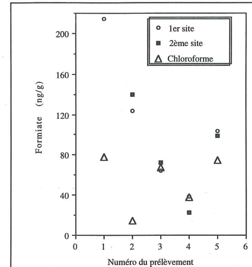
Figure 3.19: Comparaison des concentrations en formiate, entre des échantillons de neige fraîche stockés avec du chloroforme à température ambiante, et des échantillons prélevés en deux endroits différents et conservés au froid.
