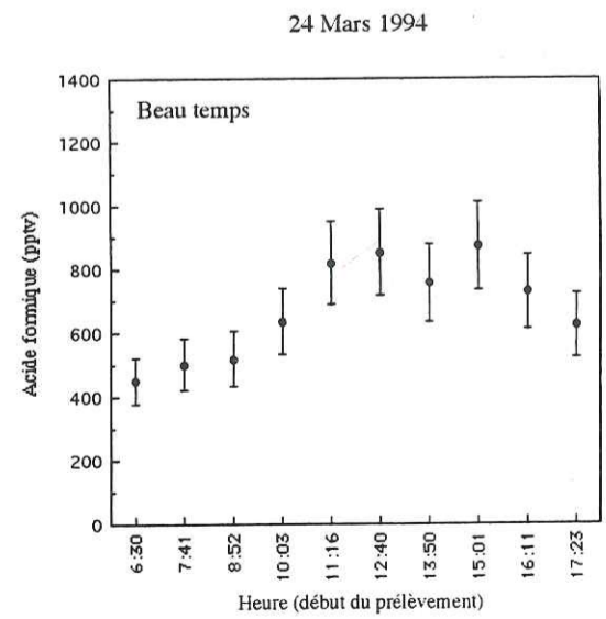
Figures A1: Suivis journaliers des concentrations atmosphériques d'acide formique (exprimées en pptv) sur le campus de Saint-Martin d'Hères (Isère).
