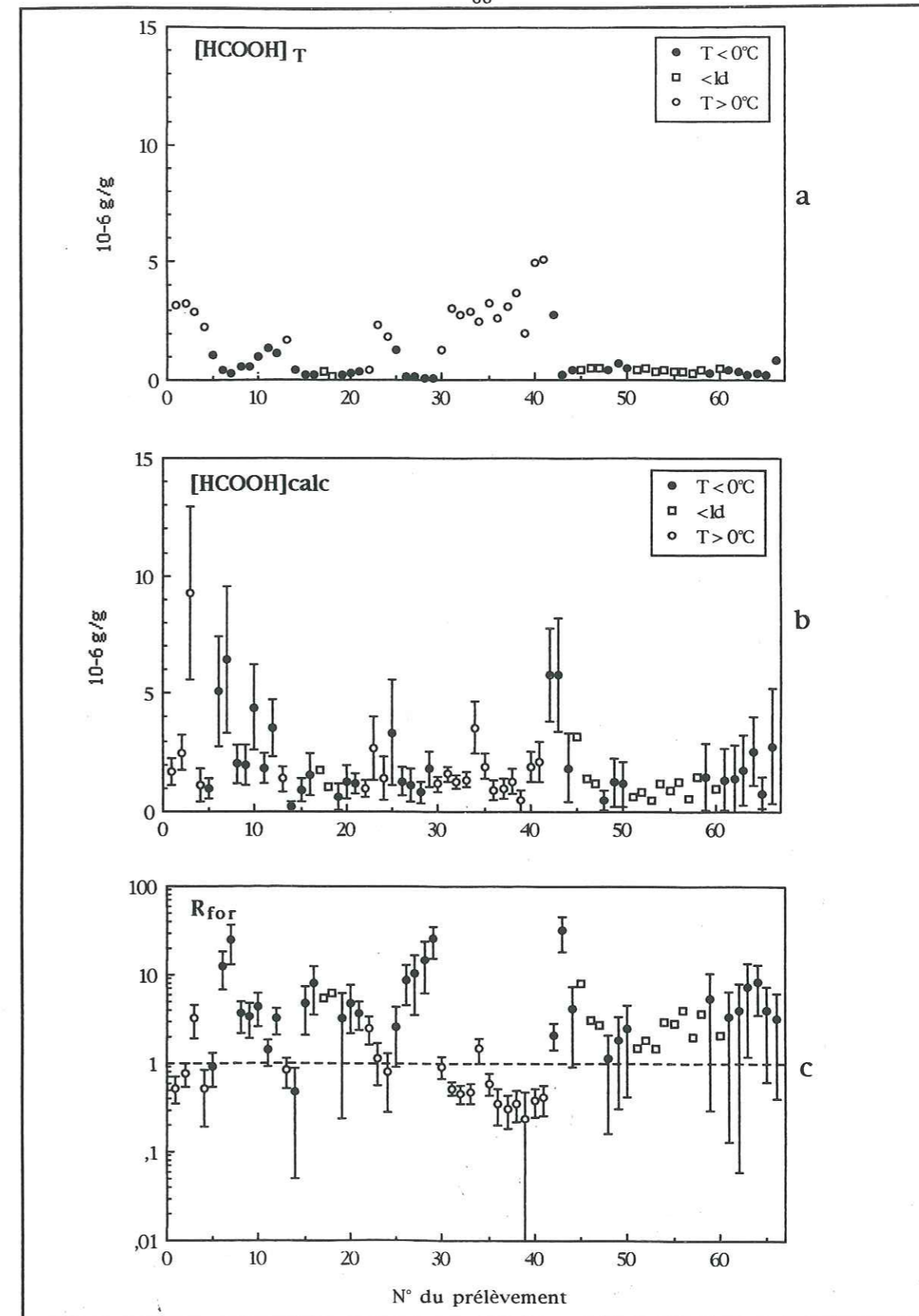
Figures 5.8: [HCOOH]_T (a), [HCOOH]_{calc} (b) exprimées en \mu g \cdot g^{-1} et écart à la loi de Henry R_{for} (c), pour chacun des prélèvements.
