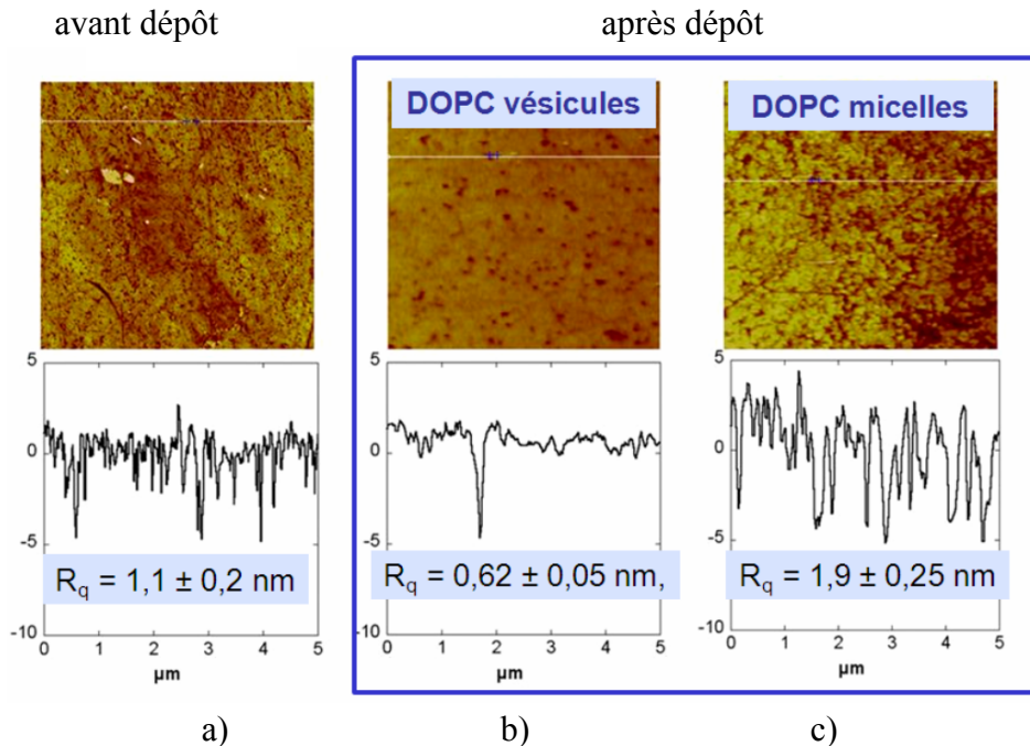
Figure 80. Variation des profils de rugosité mesurés par AFM (surface de 5 \times 5 \mu\text{m} ) pour la surface en verre « poli » : (a) avant dépôt, après nettoyage et (b-c) après dépôt, avec des bicouches de \text{DOPC}_v (b) et respectivement \text{DOPC}_m 2 incubations (c)
