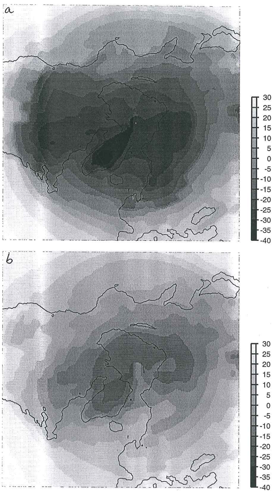
figure IV.19 : températures moyennes annuelles ( ^{\circ}\text{C} ) au sol issues des simulations LMD5ter interpolées sur la grille 50x50 km:
