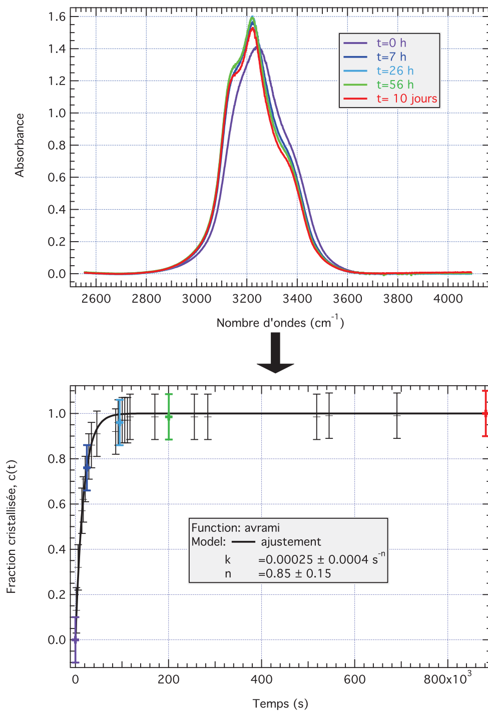
FIGURE 3.27 – Evolution de la fraction cristalline à 135 K au cours du temps. Aux fractions cristallisées en couleur s'associent les modes vibrationnels ( \nu_1 et \nu_3 ) de la glace d'eau, acquis à des instants t singuliers. Cette évolution est décrite par une loi d'Avrami.
