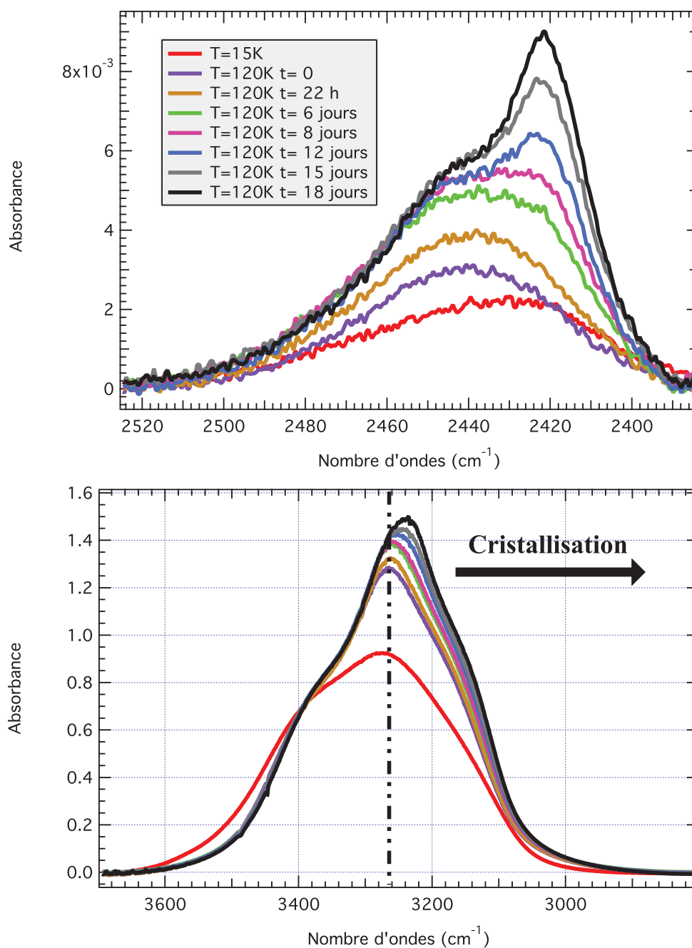
FIGURE 3.22 – En haut- Évolution à 120 \text{ K} et au cours du temps du mode vibrationnel \nu_{OD} (HOD) à \sim 2420 \text{ cm}^{-1} , congestionné dans la bande infrarouge caractéristique de \text{CD}_3\text{OD} ( \sim 2500\text{-}2350 \text{ cm}^{-1} ). En bas- Évolution des modes vibrationnels d'étiirements symétrique et antisymétrique de la glace d'eau ( \nu_1 et \nu_3 ) ( \sim 3300 \text{ cm}^{-1} ) à 120 \text{ K} et au cours du temps. Le déplacement vers les basses fréquences de ces modes indiquent que le mélange est en cours de cristallisation.
