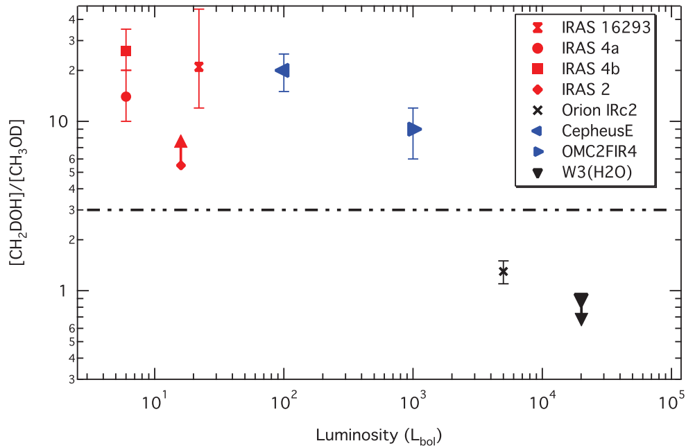
FIGURE 4.8 – Les rapports d’abondance R = \frac{[CH_2DOH]}{[CH_3OD]} , entre les isotopologues deutérés du méthanol, déduits des observations d’étoiles massives (en noir), d’étoiles de masse intermédiaire (en bleu) et d’étoiles de faible masse (en rouge). Ces rapports sont tracés en fonction de la luminosité de l’étoile. Les différents rapports et luminosités sont extraits de Parise et al. (2006) pour les étoiles de faible masse et de Jacq et al. (1993) pour le coeur chaud et dense Orion IRc2. Les autres rapports sont déduits de nos observations. A noter que la limite supérieure reportée dans la table 4.5 pour la protoétoile massive G24.78+0.08 n’est pas présente sur la figure. Cette absence est liée à l’identification incertaine de la raie de CH_3OD à 133.9254 GHz. La ligne en pointillée représente la valeur de R prédite par un modèle de chimie sur les grains ( Charnley et al. , 1997).
