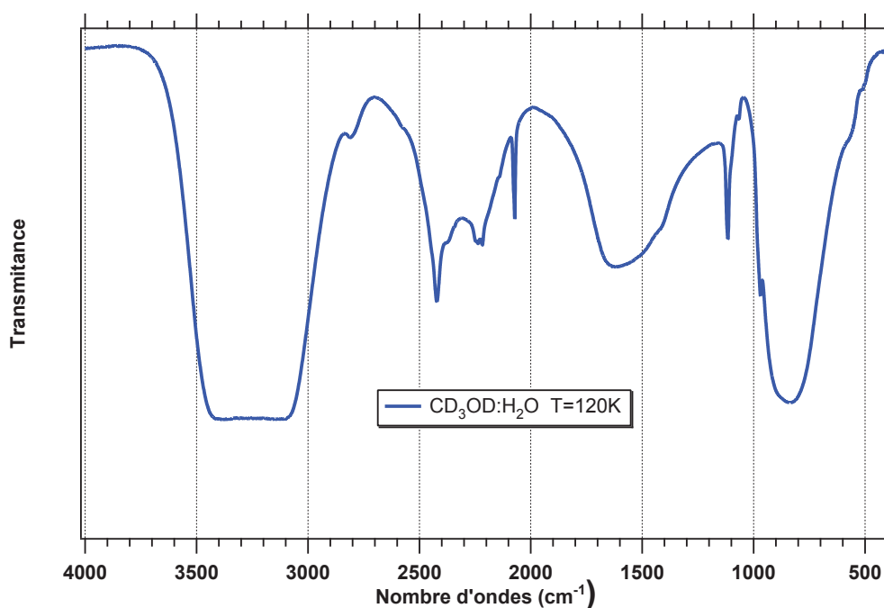
FIGURE 2.3 – Spectre infrarouge d'un mélange de glace d'eau et de méthanol à 120 K.
