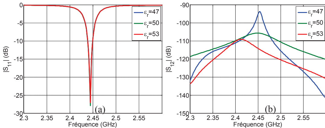
Figure IV-41 – Coefficient de réflexion (a) et de transmission (b) pour différentes valeurs de permittivité
