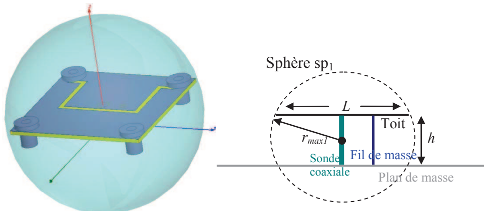
Figure II-46 – Sphère sp_1 ou sphère de Chu englobant le toit de l'antenne
