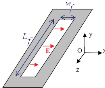
Figure II-25 – Modélisation d'une fente courte excitée par un champ électrique à polarisation uniforme
