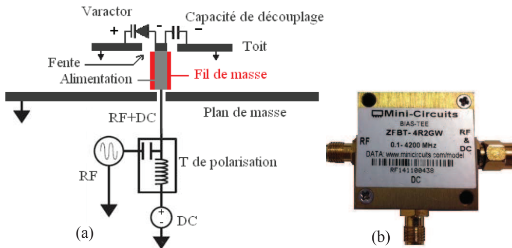
Figure III-25 – Circuit de polarisation de la diode varicap (a) et T de polarisation (b)
