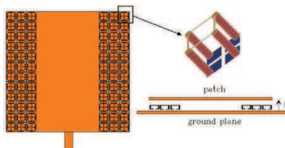
Figure I-26 - Géométrie de l'antenne microruban réalisée sur un substrat partiel d'une couche et 3 colonnes de matériau magnétique artificiel [I.60]
