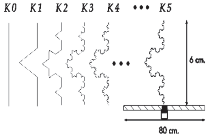
Figure I-15 – Monopoles à géométrie fractale de Koch [I.40]
