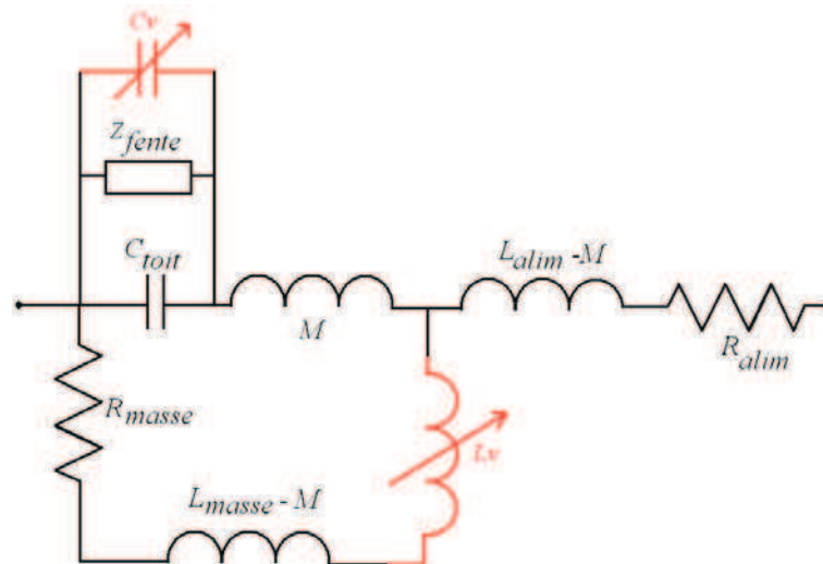
Figure III-55 – Circuit équivalent de l'antenne à la fréquence de résonance basse
