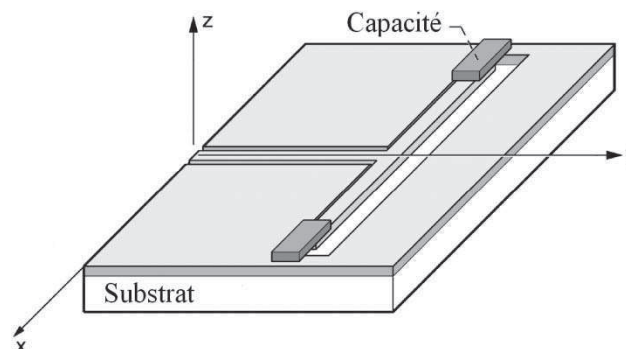
Figure I-11 - Antenne à fente avec charge capacitive [I.37]
