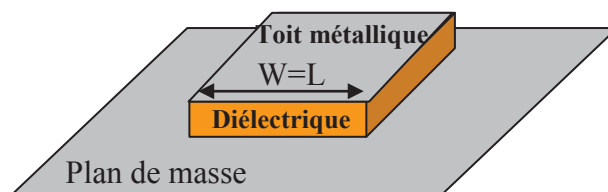
Figure I-18 – Antenne microruban avec substrat diélectrique
