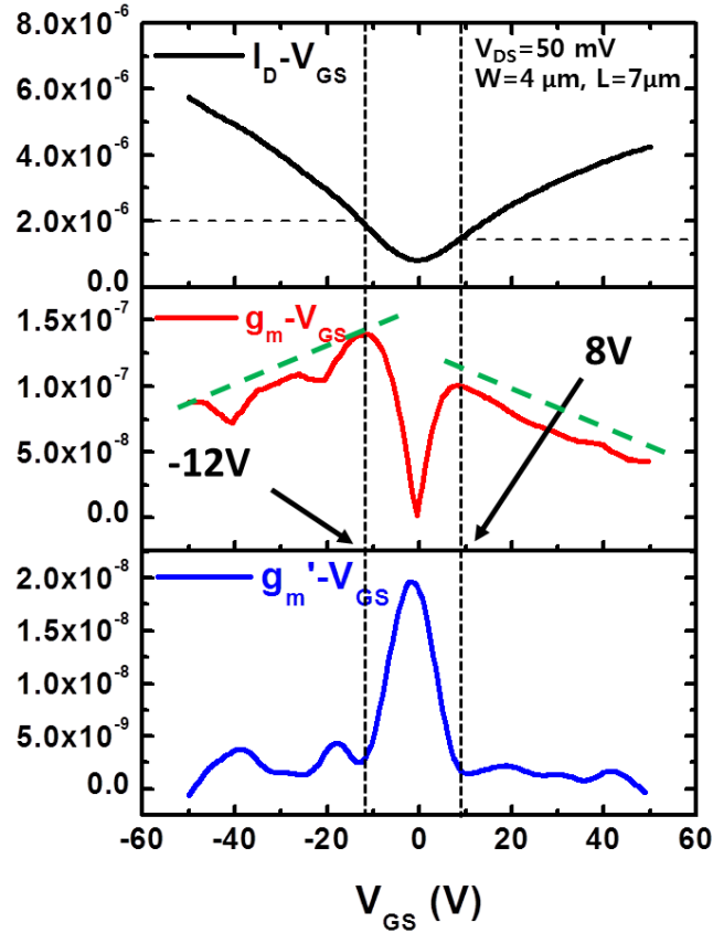
Figure 19 Les caractérisations I_D-V_{GS} et g_m-V_{GS} d'un G-FETs.
