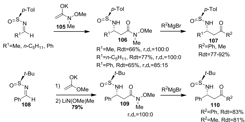
Schéma II.22 : Synthèse de \beta -aminocétone chirales
