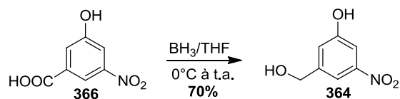
Schéma III.56 : Synthèse de l'alcool benzylique 364
