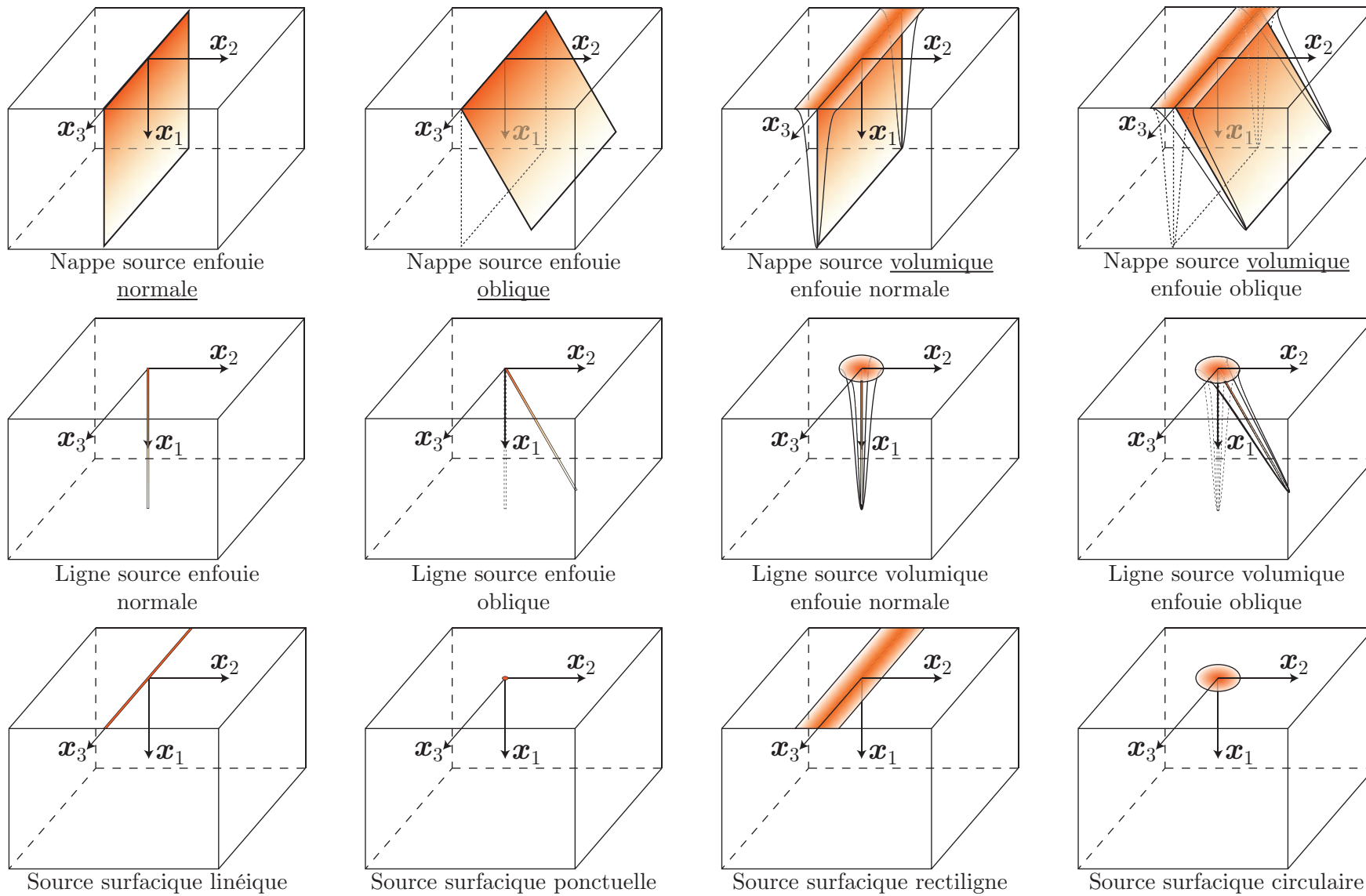
Fig. 1.1 – Représentation schématique des différentes sources acoustiques considérées dans ce manuscrit.
