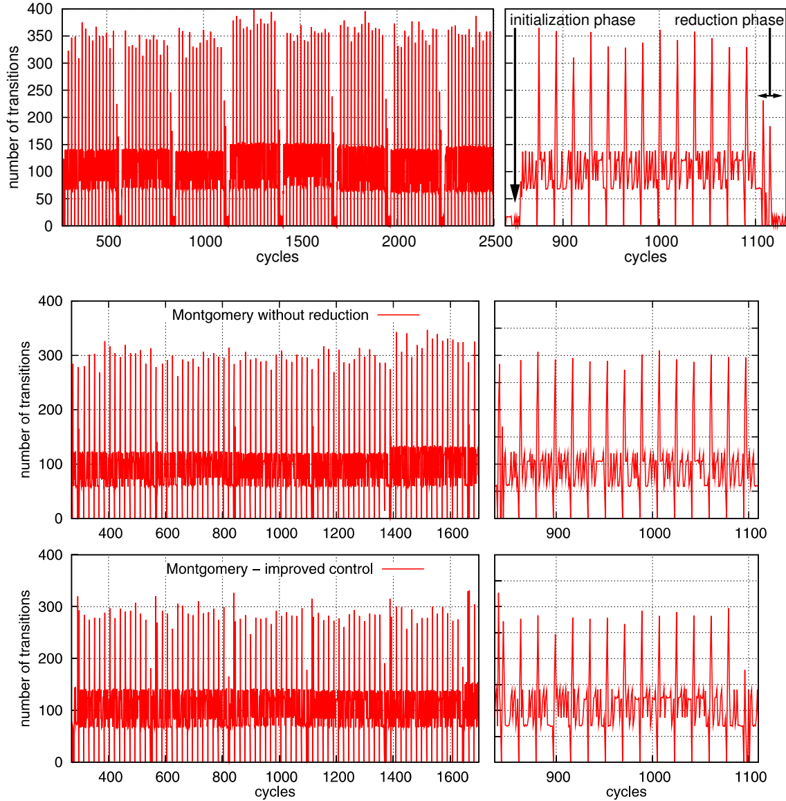
FIGURE 4.: L'activité utile de solution basé sur l'algorithme de Montgomery.
