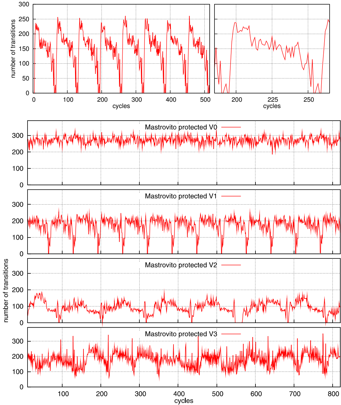
FIGURE 5.: L'activité des solutions basées sur la conception de Mastrovito (4 versions).
