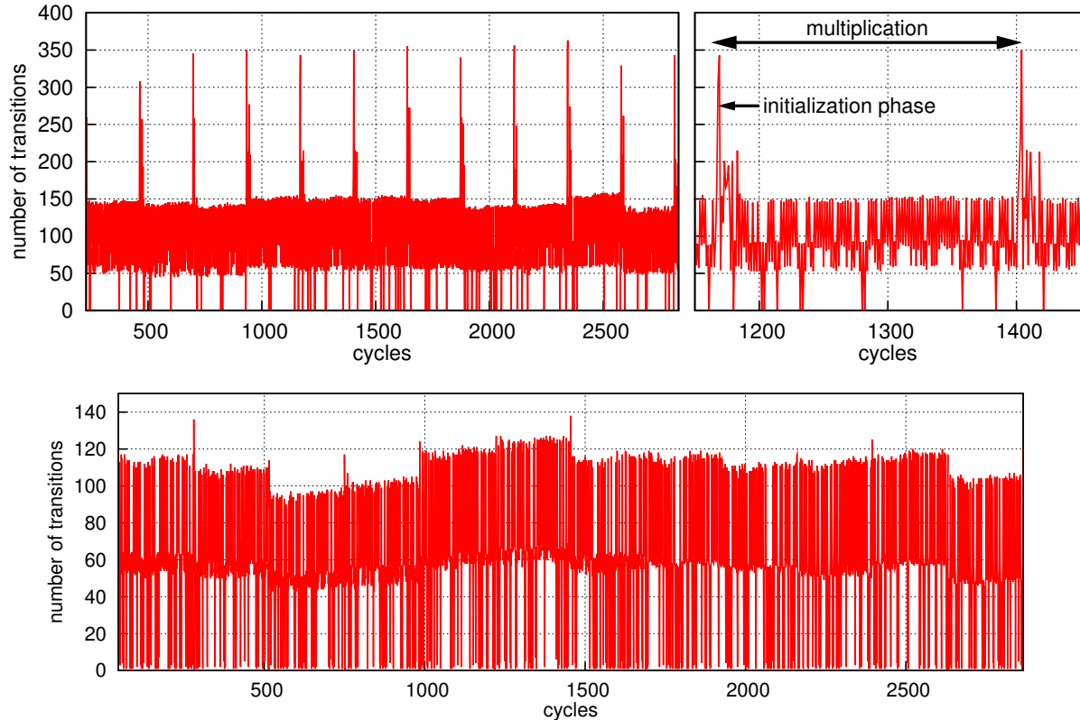
FIGURE 3.: L'activité utile de la solution classique
