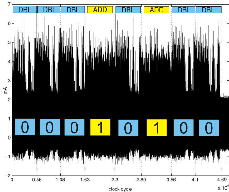
FIGURE 1.: L'exemple de SPA (analyse simple de consommation) d'algorithme 1
