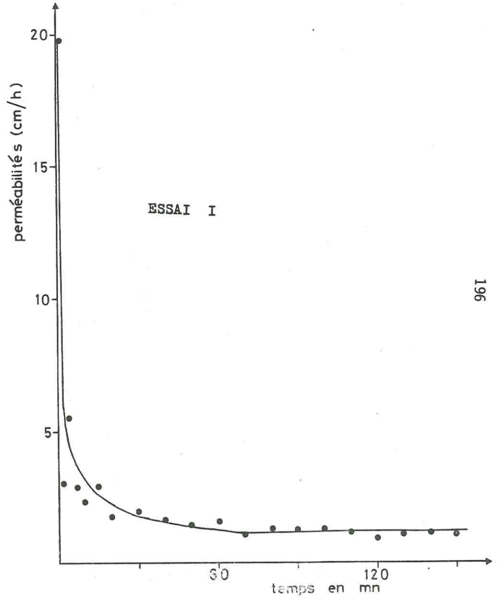
Figure n°56 : Courbes ( perméabilités - temps ) interprétatives des essais d'infiltration.
