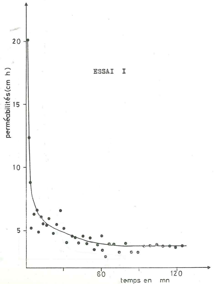
Figure n°57 : Courbes ( perméabilités - temps ) interprétatives des essais d'infiltration.
