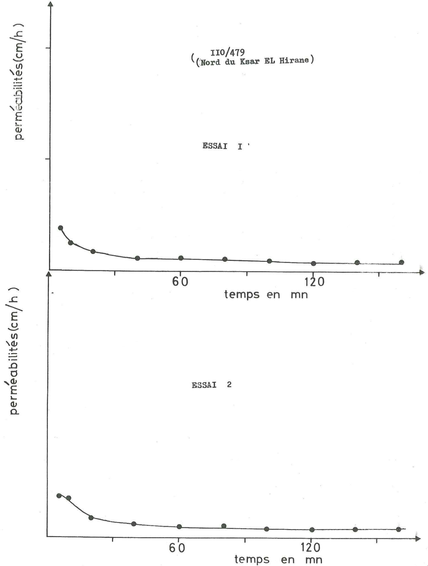
Figure n°62 : Courbes ( perméabilités - temps ) interprétatives des essais d'infiltration.
