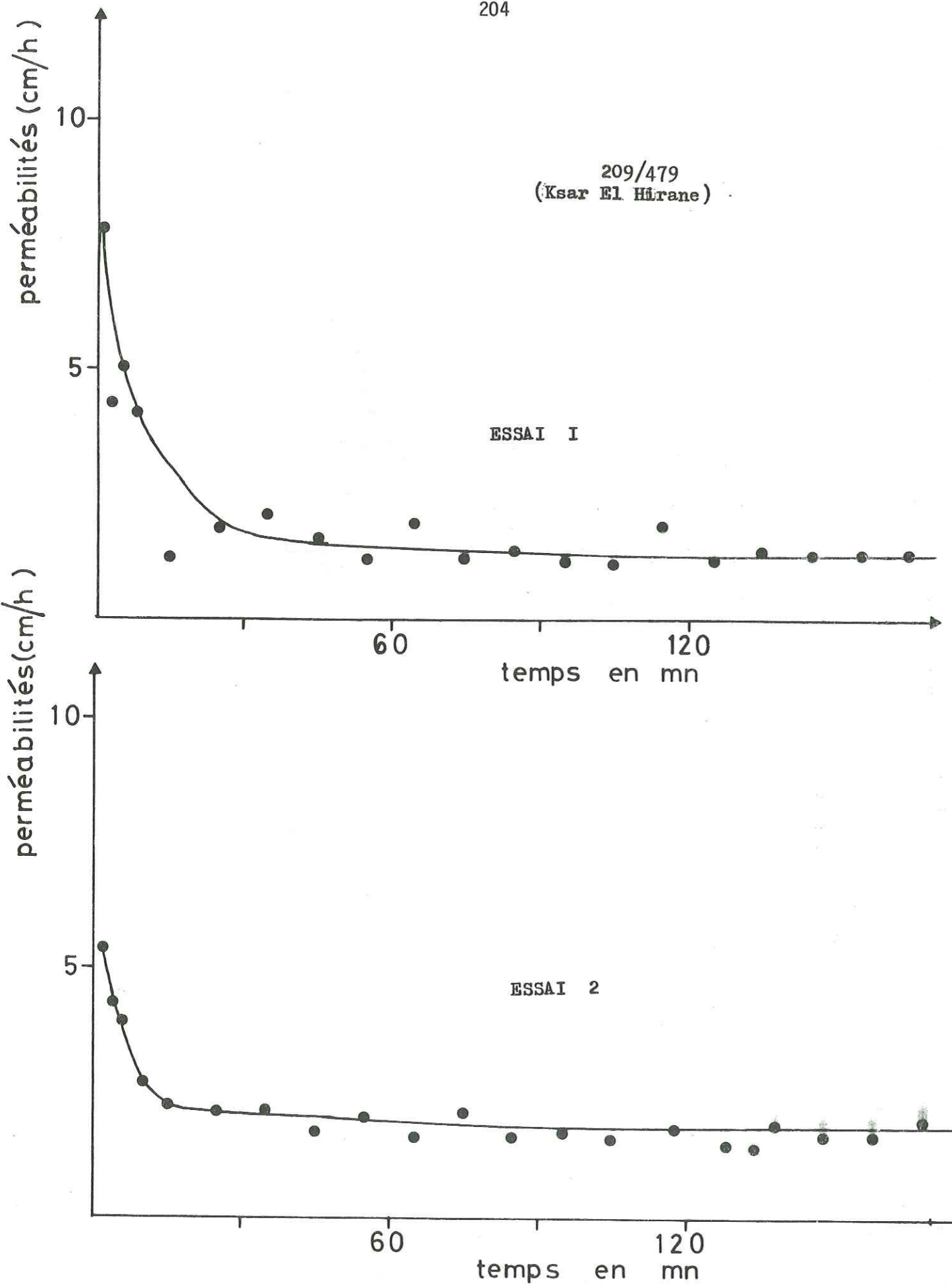
Figure n°63 : Courbes ( perméabilités - temps ) interprétatives des essais d'infiltration.
