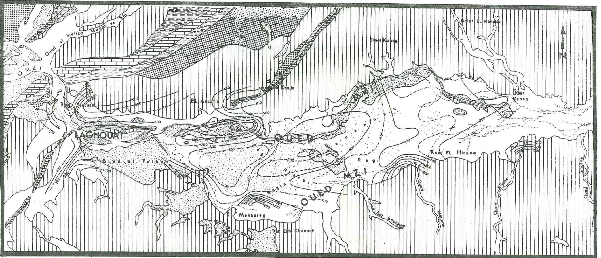
Carte de la résistivité des eaux de la vallée de l'oued M'Zi. ( période du 1 au 10 /05 /1980 ).
