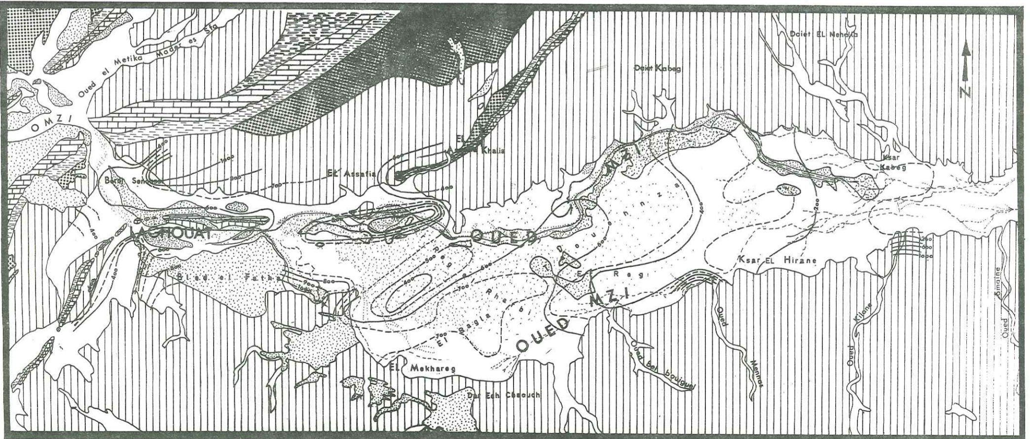
Carte de la résistivité des eaux de la vallée l' oued M'Zi. ( periode du 20 / 06 au 5 /07 / 1980 )..
