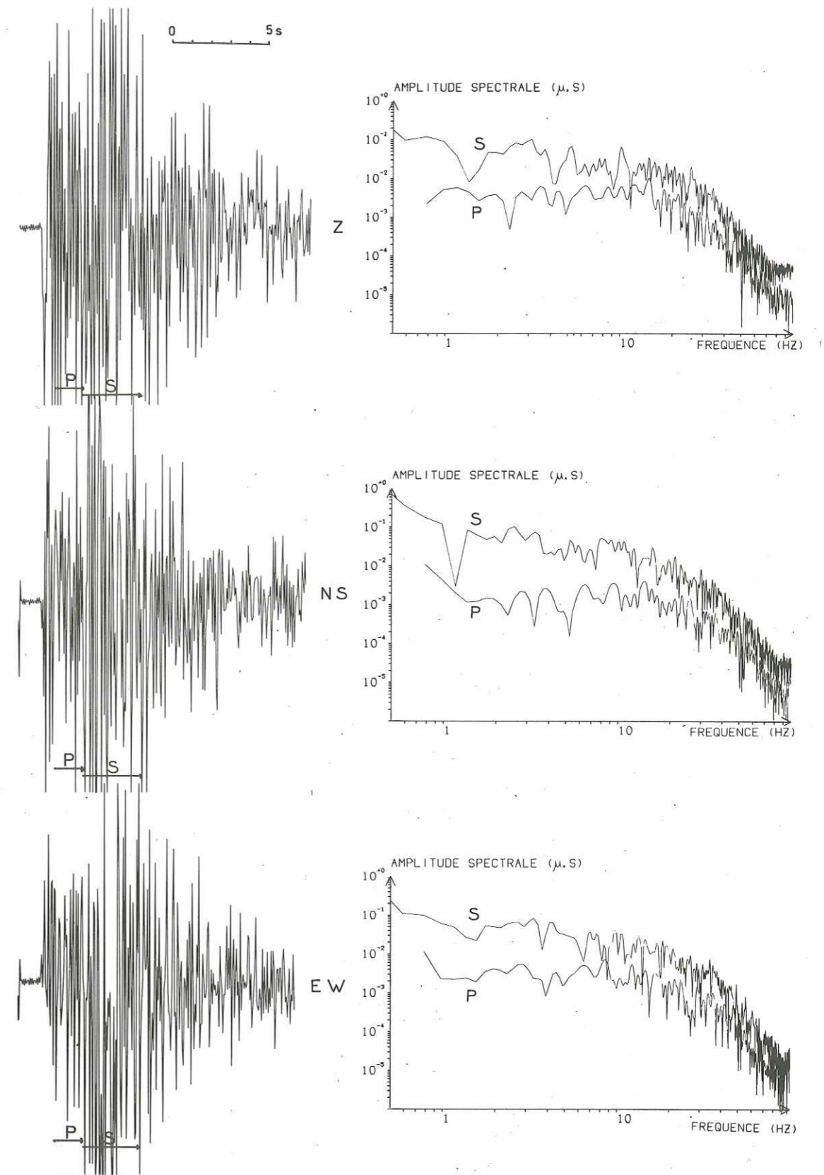
Figure III.6 (suite) Influence de la coda de l'onde P sur le spectre de l'onde S, pour les trois composantes de la station TES (séisme N° 11). Les flèches sur les sismogrammes indiquent les échantillons utilisés pour les deux phases.
