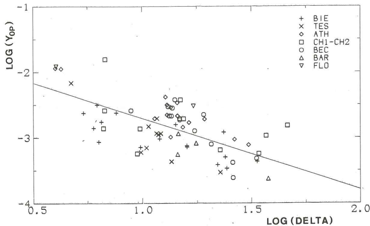
Figure IV.5 Vérification de la validité de la loi d'expansion géométrique en 1/\Delta . Valeurs du niveau plat Y_0 portées en fonction de la distance hypocentrale pour chaque couple séisme-station. Les niveaux plats ont été normalisés de façon à ce que tous les séismes aient le même moment sismique. En haut pour l'onde S, en bas pour l'onde P.
