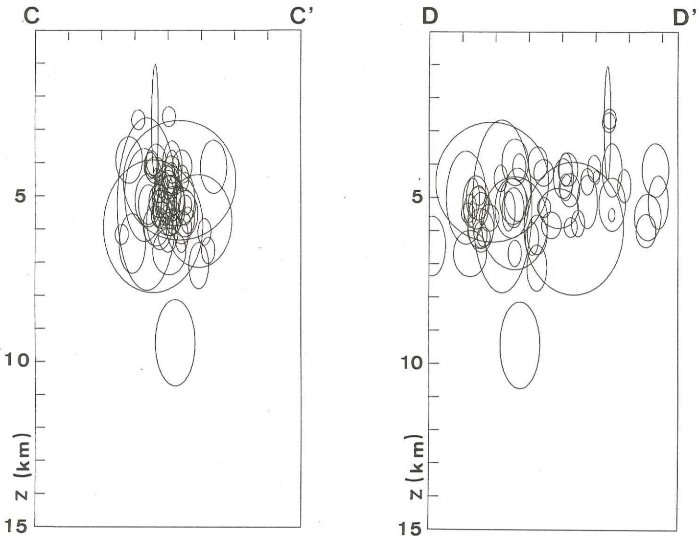
Figure IV.5 coupes E-w et N-S correspondant aux segments CC' et DD' de la figure IV.4. Les ellipses, centrées sur les foyers correspondent aux erreurs ERH et ERZ données par le programme HYP071. Expérience d'Arudy 1980.
