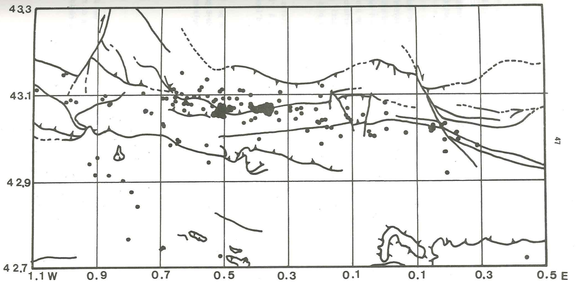
Figure IV.9 Relation entre la sismicité et les accidents géologiques de la carte structurale de P. Choukroune et M. Séguret.
