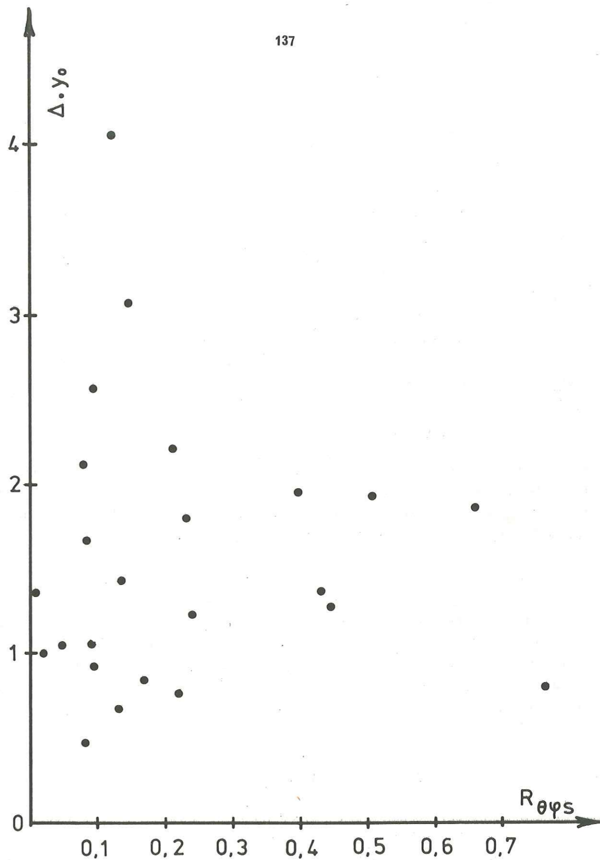
Figure IV.9 Valeurs du niveau plat \gamma_{0S} des spectres de l'onde S corrigés de l'expansion géométrique (multipliés par la distance hypocentrale), en fonction du facteur de radiation théorique R_{\theta\psi S} calculé à partir des solutions focales de la première partie.
