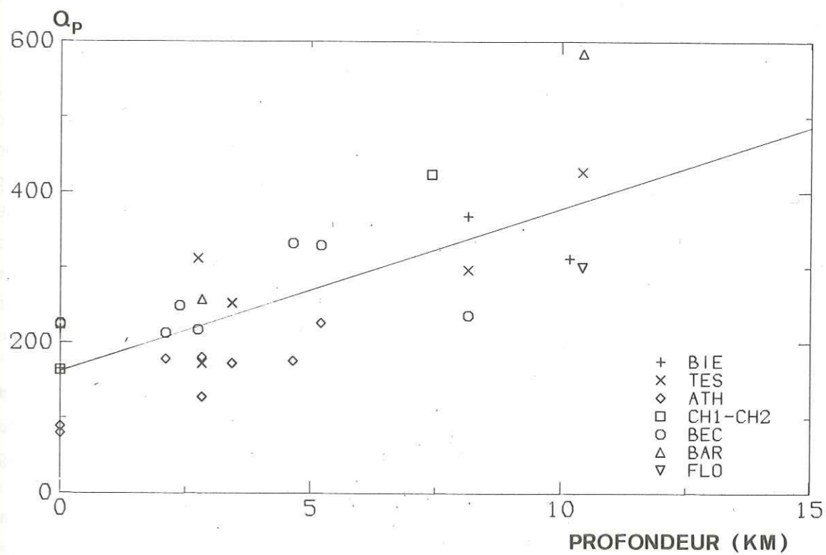
Figure IV.4 Variation du facteur de qualité Q avec la profondeur des foyers pour chaque couple sisme-station dont les distances hypocentrales sont comprises entre 10 et 20 km. En haut pour l'onde S, en bas pour l'onde P. Des symboles différents ont été utilisés pour chaque station.
