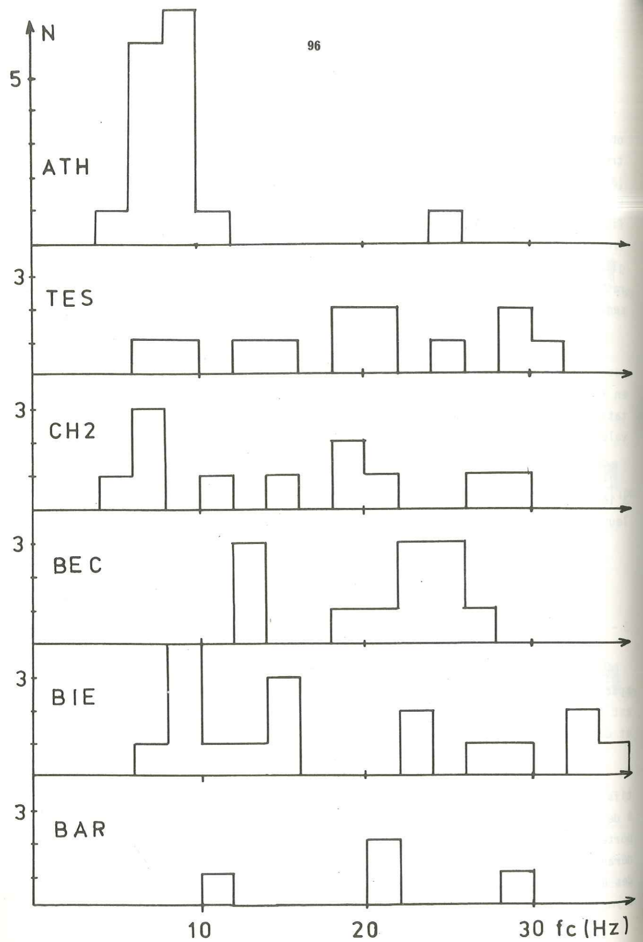
Figure III.3 Histogrammes par station des fréquences coin des spectres des ondes P.
