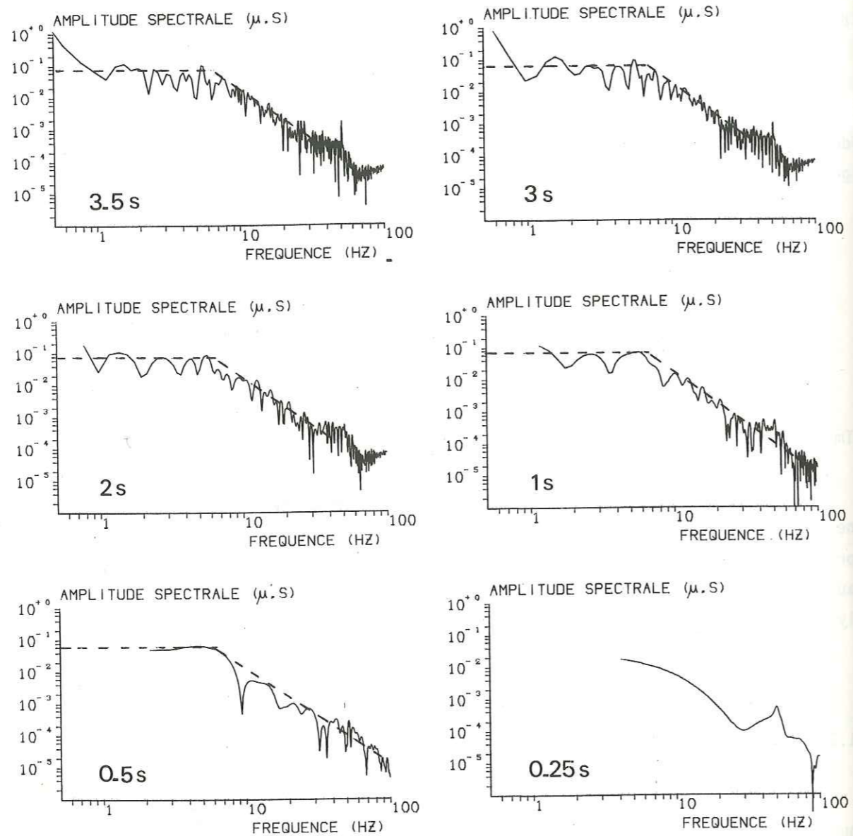
Figure II.2 Influence de la longueur de l'échantillon. Spectres de l'onde P d'un même séisme calculés avec des longueurs d'échantillon de 0,25 s à 3,5 s.
