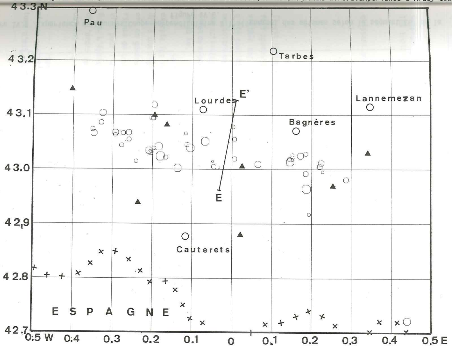
Figure IV.6 Epicentres des séismes localisés lors de l'expérience de Lourdes. \circ séismes, la taille des symboles est proportionnelle à la magnitude locale. \blacktriangle stations utilisées.
