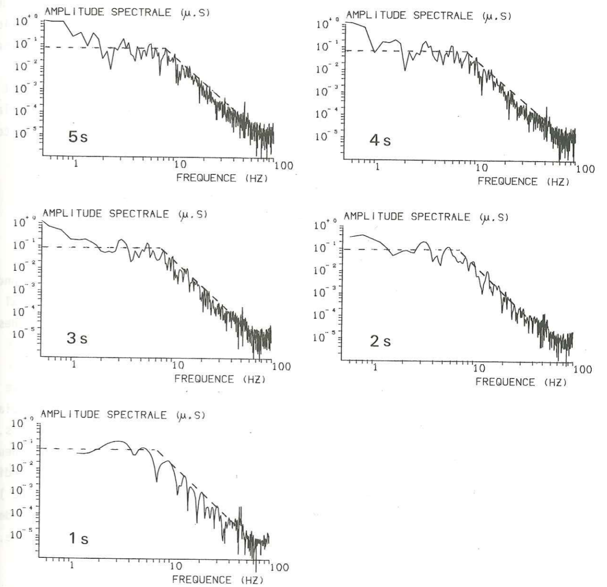
Figure II.3 Influence de la longueur de l'échantillon. Spectres de l'onde S d'un même séisme calculés avec des longueurs d'échantillon de 1s à 5s.
