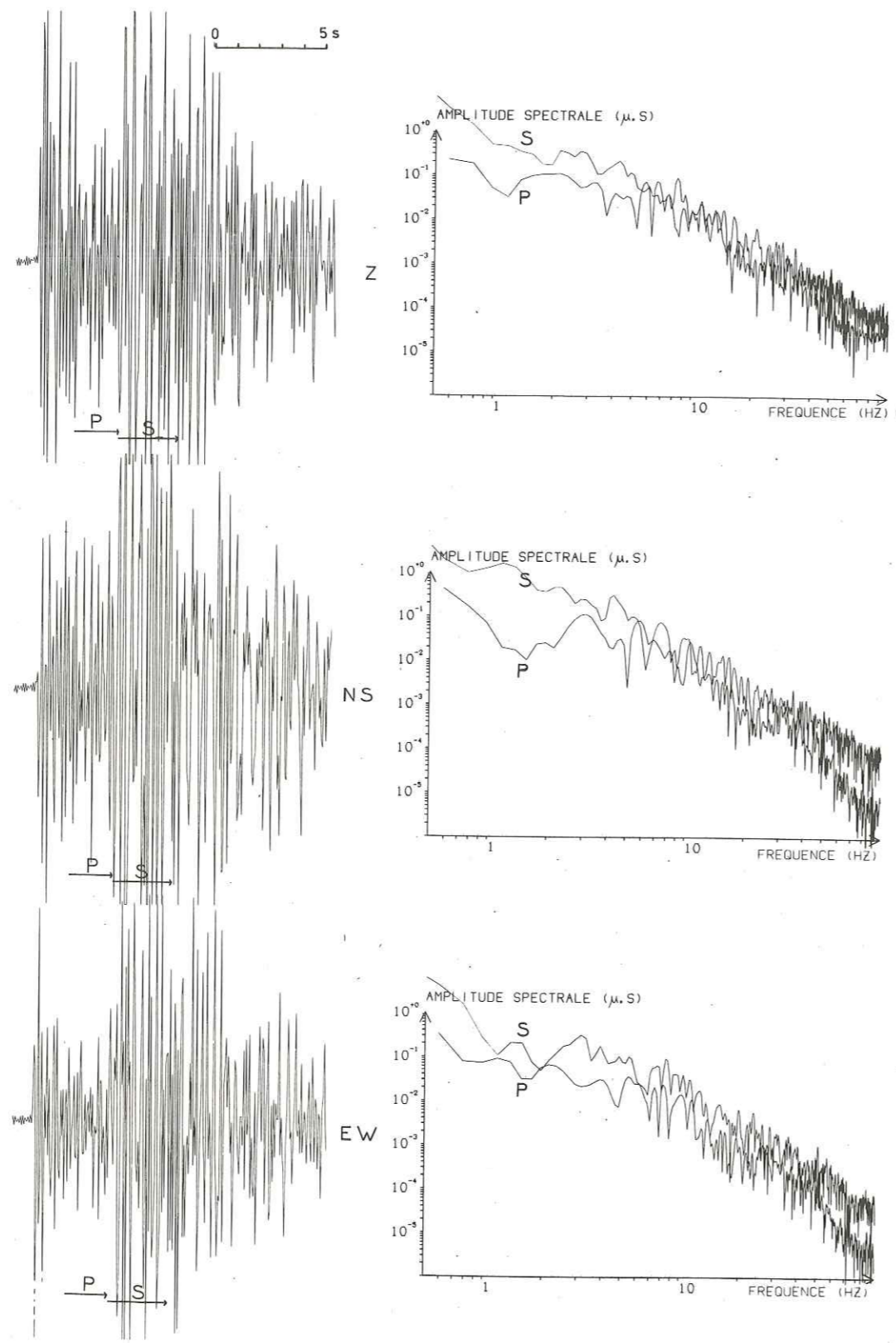
Figure III.6 (suite) Influence de la coda de l'onde P sur le spectre de l'onde S, pour les trois composantes de la station BIE (séisme N° 8). Les flèches sur les sismogrammes indiquent les échantillons analysés pour les deux phases.
