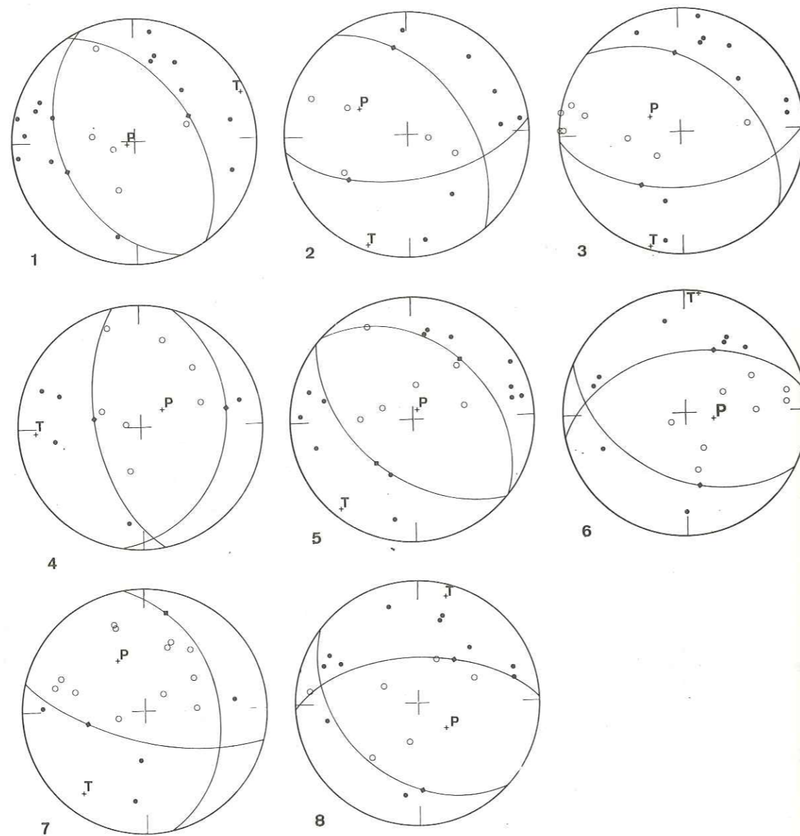
Figure V.3 Solutions focales obtenues à partir des enregistrements de l'expérience Arudy 1980. ○ dilatations, ● compressions, ◆ pôles des plans nodaux, P et T directions des axes de pression et de tension maximales.
