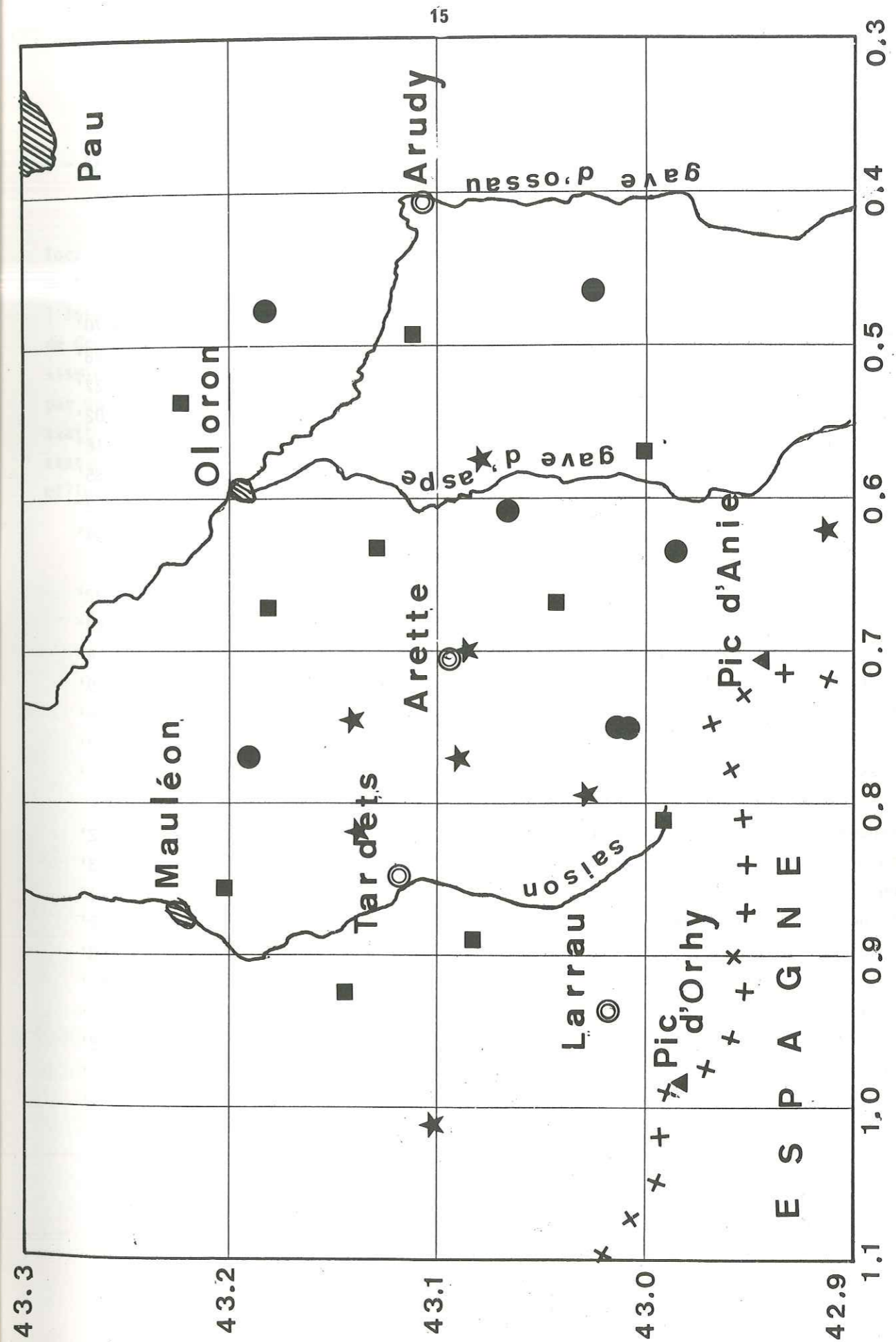
Figure II.1 Emplacement des stations utilisées pendant l'expérience Arette 1978. ● stations magnétiques analogiques, ■ stations MEQ800, ★ stations du réseau permanent.
