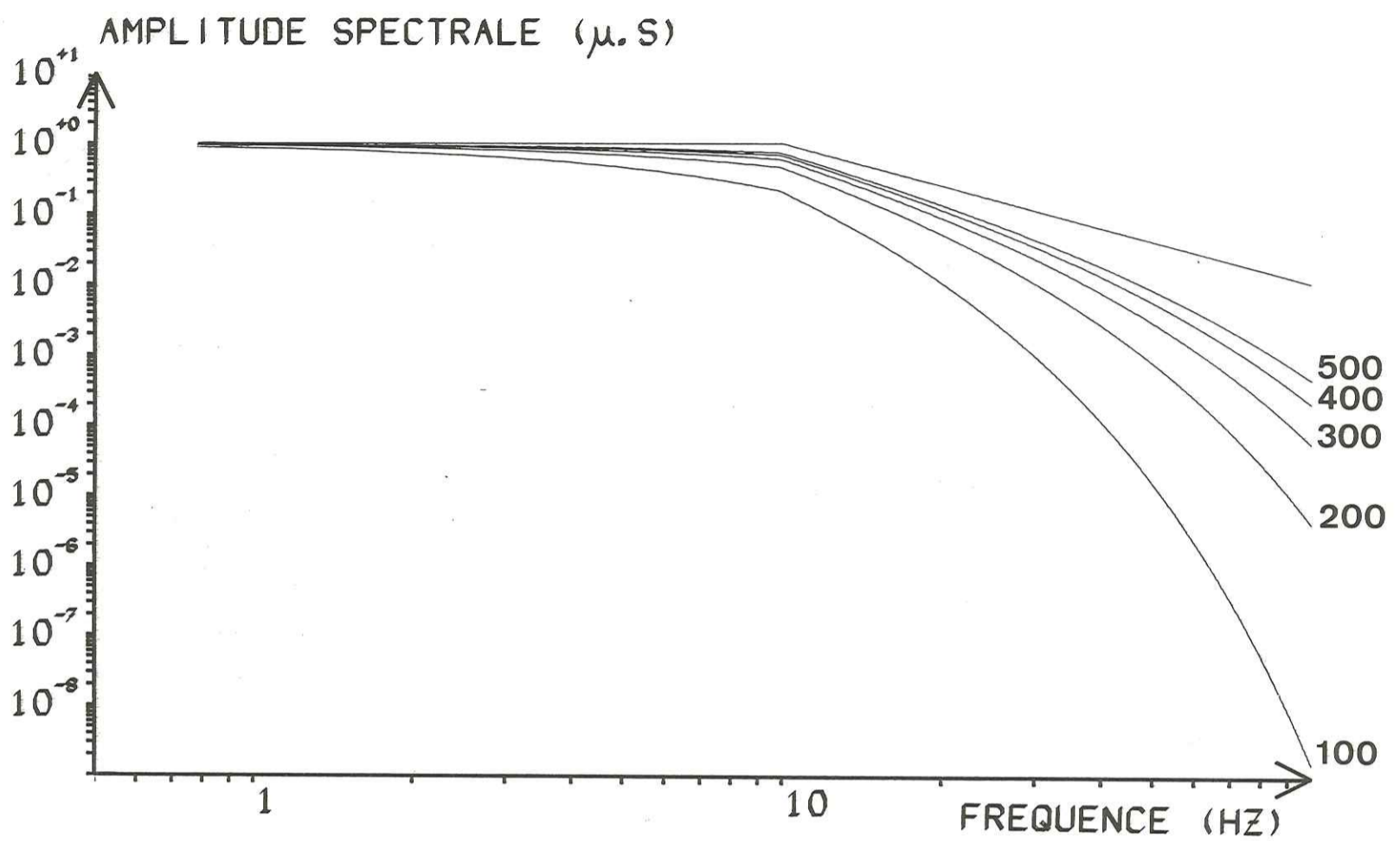
Figure IV.1 Effet de l'atténuation anélastique sur un spectre à la source symbolisé par ses deux asymptotes (spectre du haut), pour des valeurs du facteur de qualité allant de 100 à 500, une distance hypocentrale de 15 km et une vitesse de l'onde de 3 km/s.
