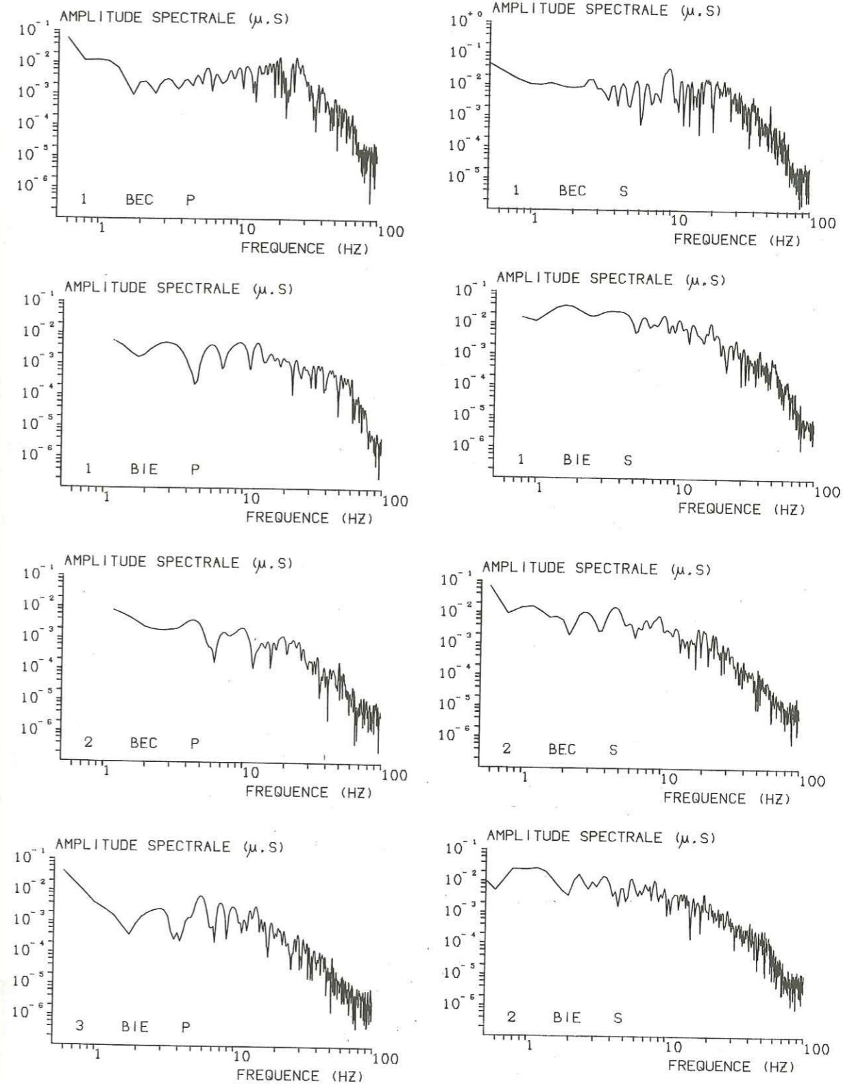
Figure III.7 spectres "totaux". L'amplitude spectrale est égale à la racine carrée de la somme des carrés des amplitudes spectrales des trois composantes. Sur chaque spectre sont notés le numero du séisme, la station et la phase.
