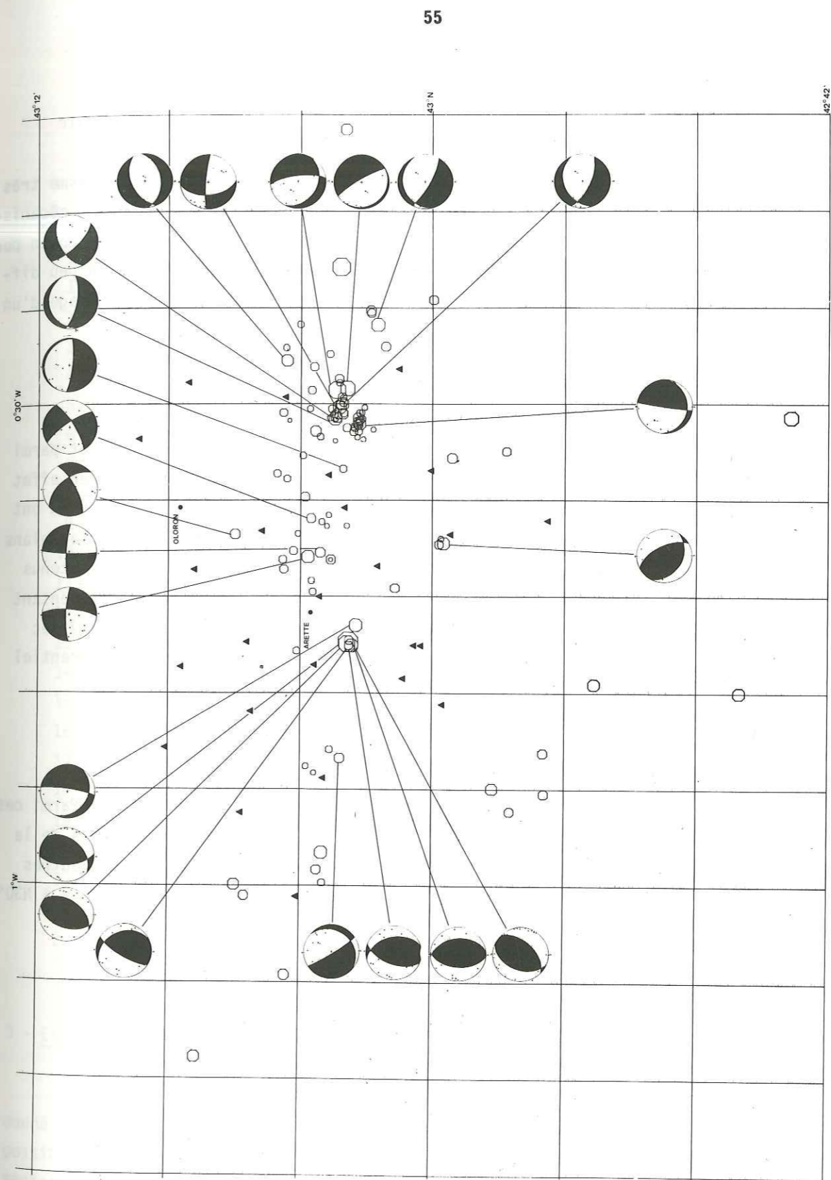
Figure V.2 Carte des mécanismes focaux obtenus à partir des données d'Arette. En noir, quadrant des compressions.
