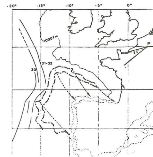
Figure I.3 Mouvement relatif de l'Ibérie par rapport au bloc européen. P représente le pôle de rotation. (Choukroune et al, 1973).
