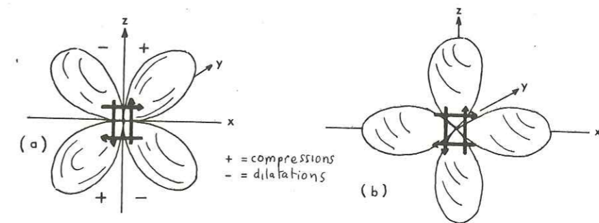
Figure IV.7 Diagrammes de radiation d'un mécanisme de double couple pour une onde P (a) et pour une onde S (b). Les plans nodaux sont les plans xoy et yoz.
