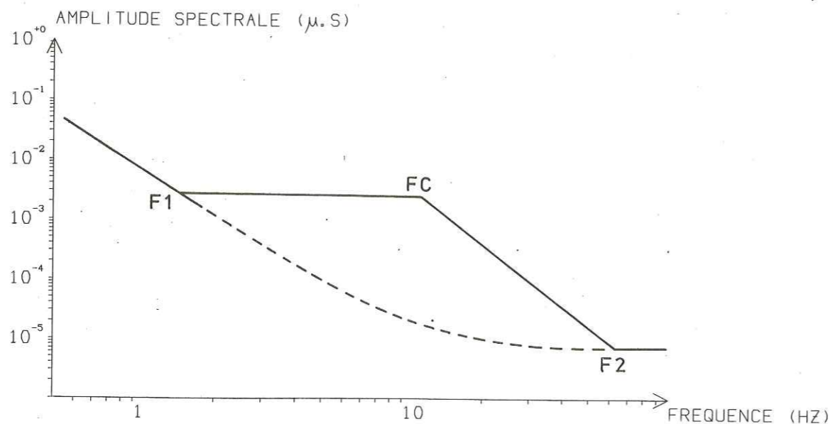
Figure III.1 Schéma du haut : en trait plein, spectre d'une onde P, en tireté, spectre du bruit de fond précédant cette onde. En bas, schématisation du spectre du haut. Cet aspect est caractéristique de l'ensemble des spectres.
