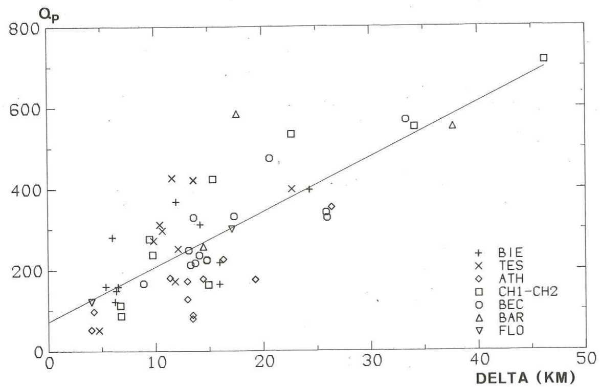
Figure IV.3 Variation du facteur de qualité Q avec la distance hypocentrale \delta pour chaque couple sisme-station. En haut pour les ondes S, en bas pour les ondes P. Des symboles différents ont été utilisés pour chaque station.
