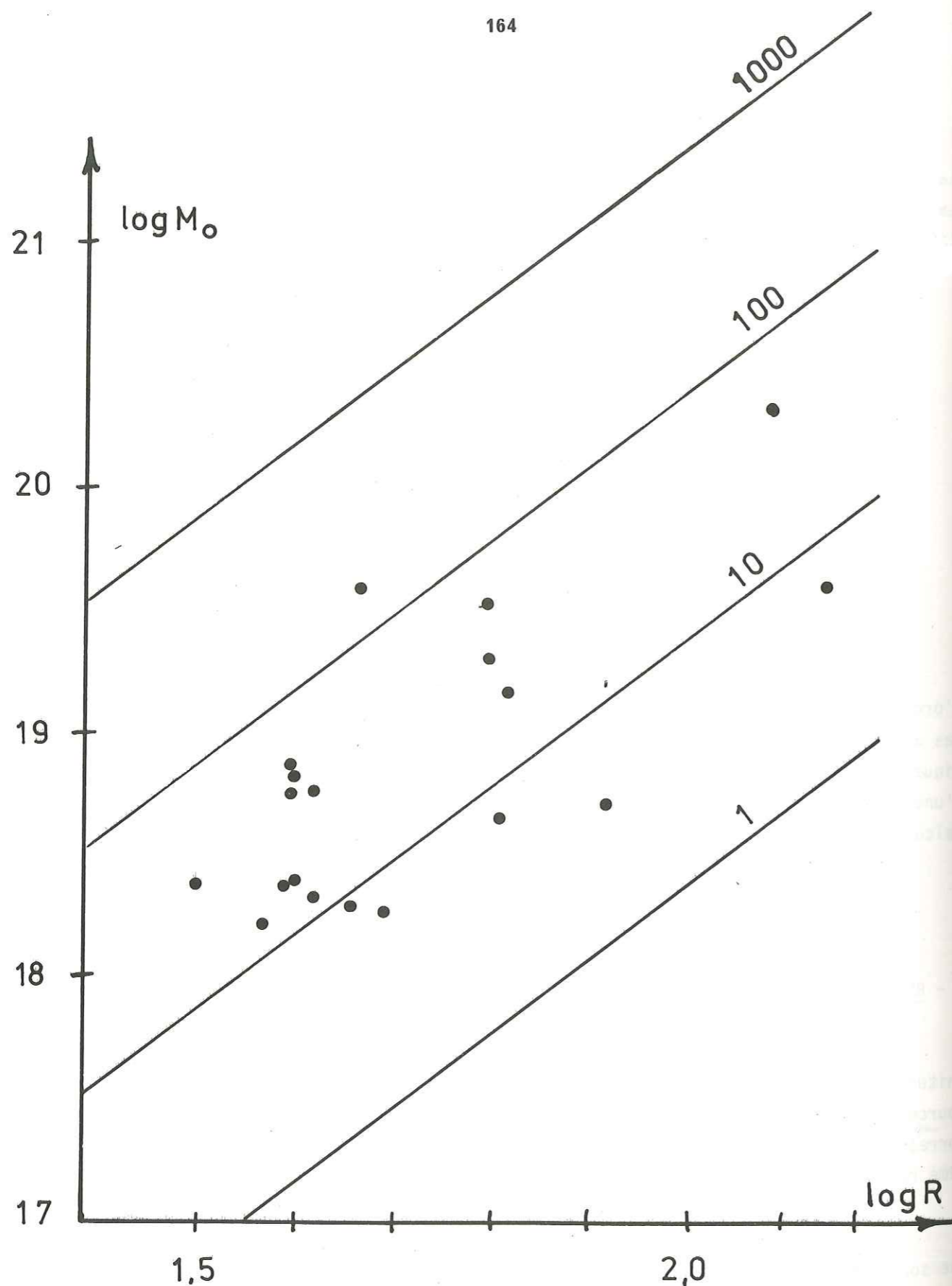
Figure V.6 Diagramme moment sismique M_0 - rayon de la source R avec les droites d'égales chutes de contraintes (Bar).
