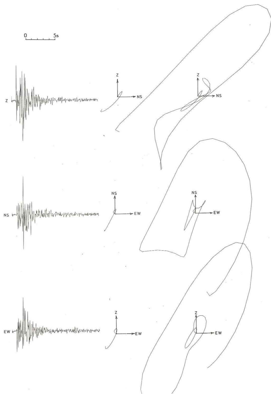
Figure III.5 Sismogrammes des trois composantes de la station BIE (séisme N° 5), et déplacement du sol dû à l'onde P projeté dans les trois plans perpendiculaires constitués par les couples de composantes. Au milieu 15 premiers centièmes de seconde de l'onde P. A droite 40 premiers centièmes de seconde de l'onde P.
