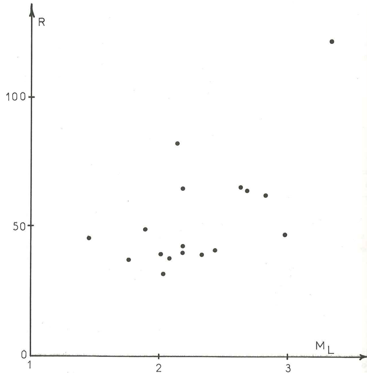
Figure V.5 Variations du rayon de la source R avec la magnitude locale M_L .
