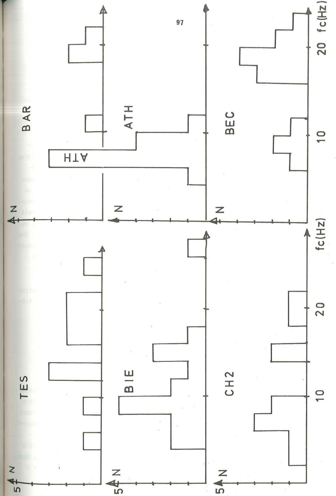
Figure III.3 (suite) Histogrammes par station des fréquences coin des spectres des ondes S.
