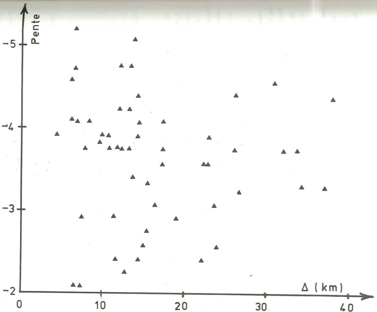
Figure IV.2 Pentas des spectres en fonction de la distance hypocentrale pour chaque couple sisme-station.
