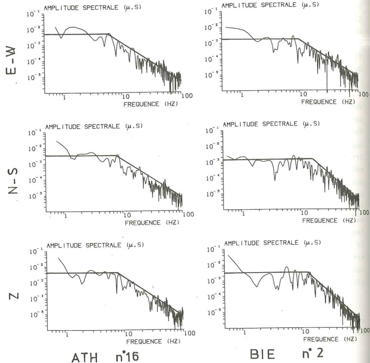
Figure III.2 Comparaison entre les spectres obtenus sur les trois composantes d'une station pour un séisme donné. Alors que les spectres de gauche sont identiques, il n'en est pas de même pour ceux de droite qui présentent des différences notables pour la fréquence coin et l'asymptote hautes fréquences.
