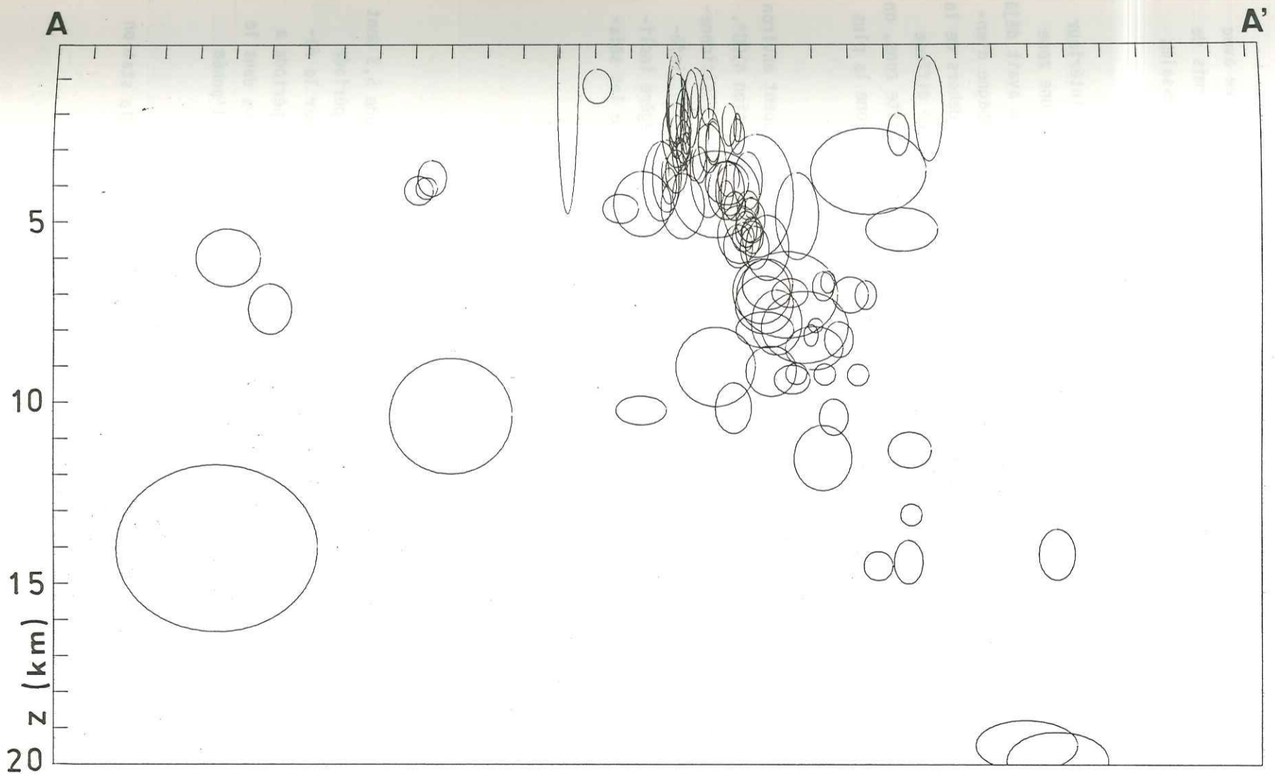
Figure IV.1 Séismes localisés à partir de l'expérience d'Arette. \circ séismes, la taille des symboles est proportionnelle
