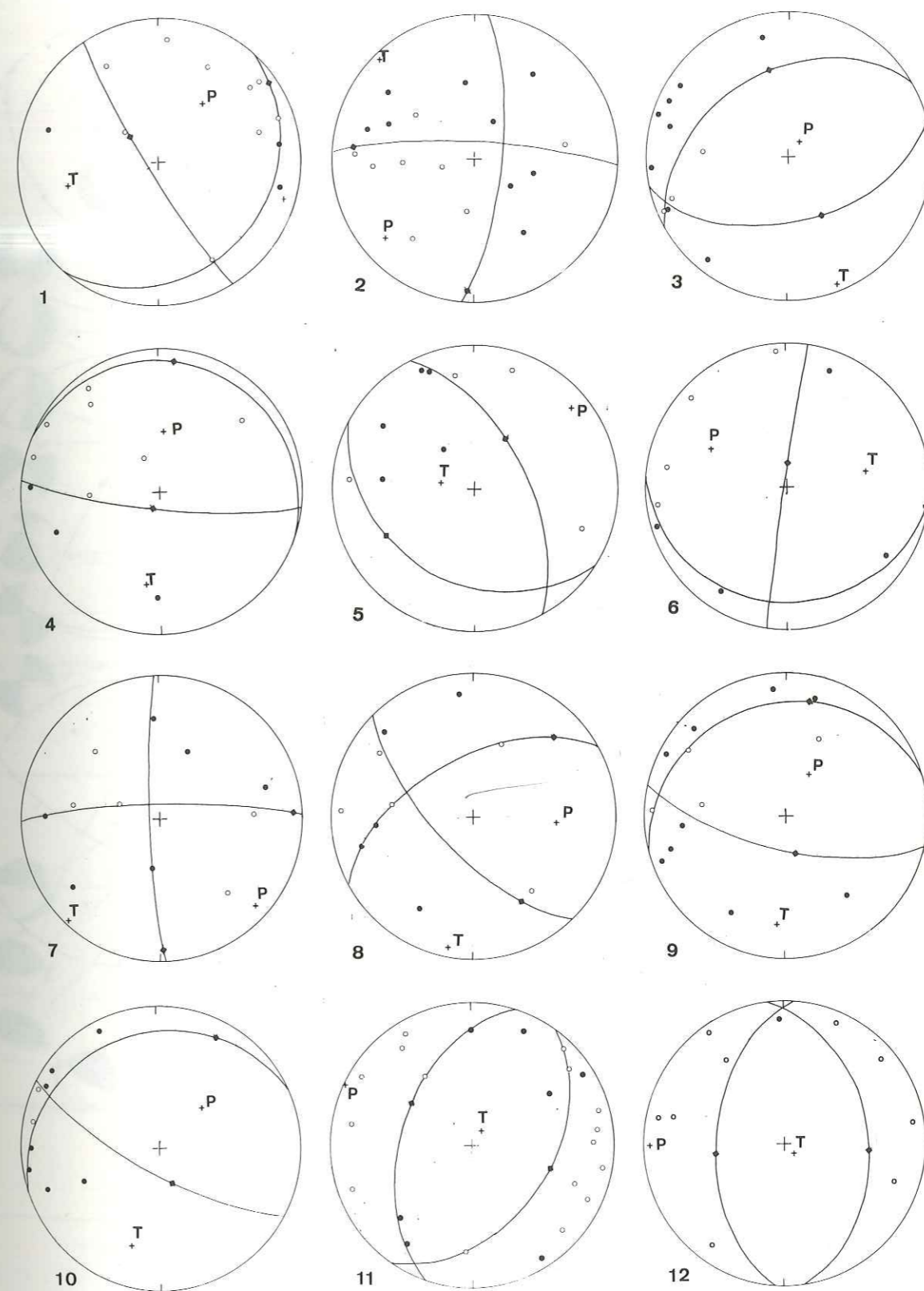
Figure V.1 Solutions focales obtenues à partir des enregistrements de l'expérience Arette 1978. ○ dilatations, ● compressions, ◆ pôles des plans nodaux, P et T directions des axes de pression et de tension maximales.
