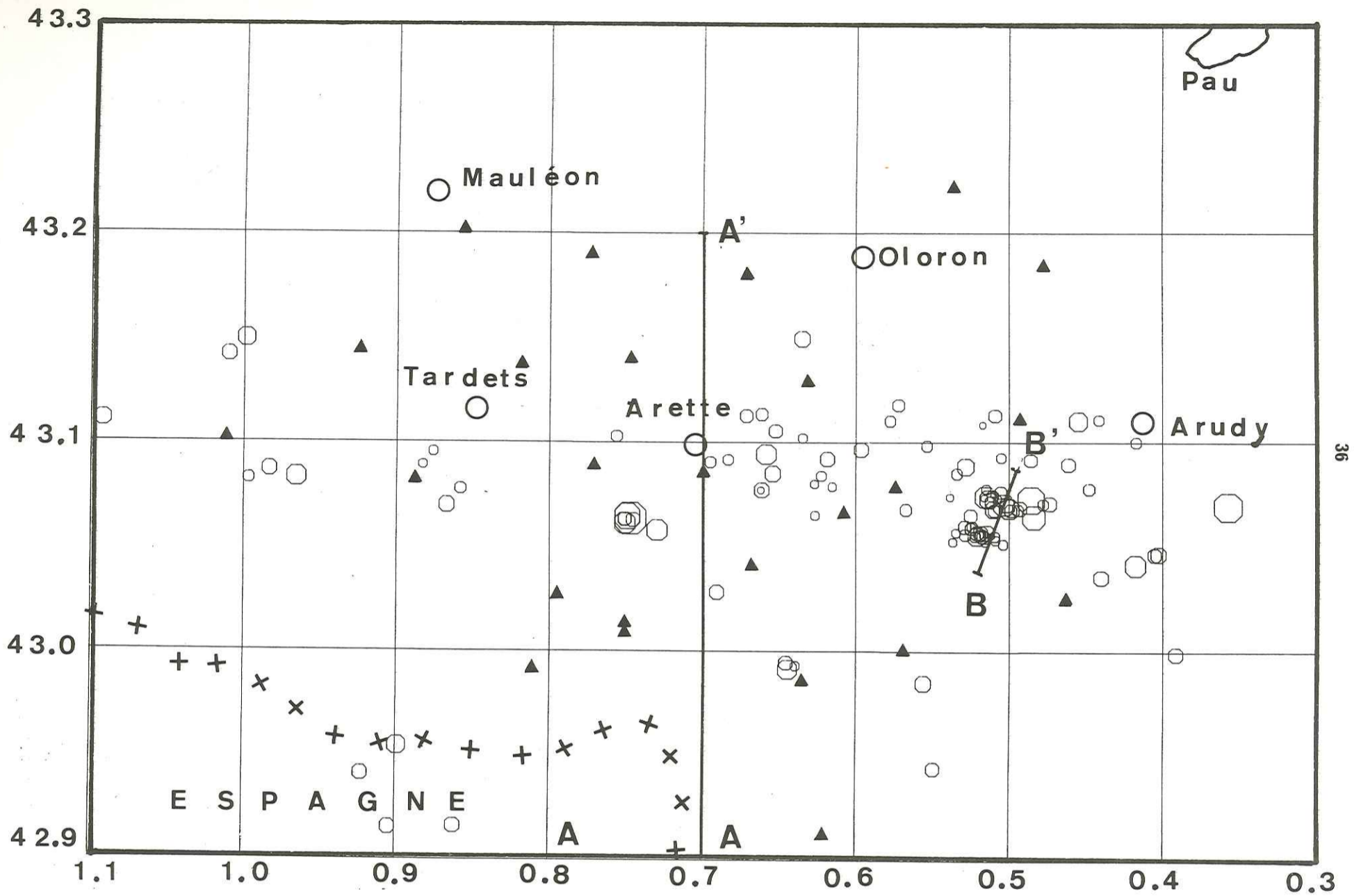
Figure IV.1 Séismes localisés à partir de l'expérience d'Arette. \circ séismes, la taille des symboles est proportionnelle
