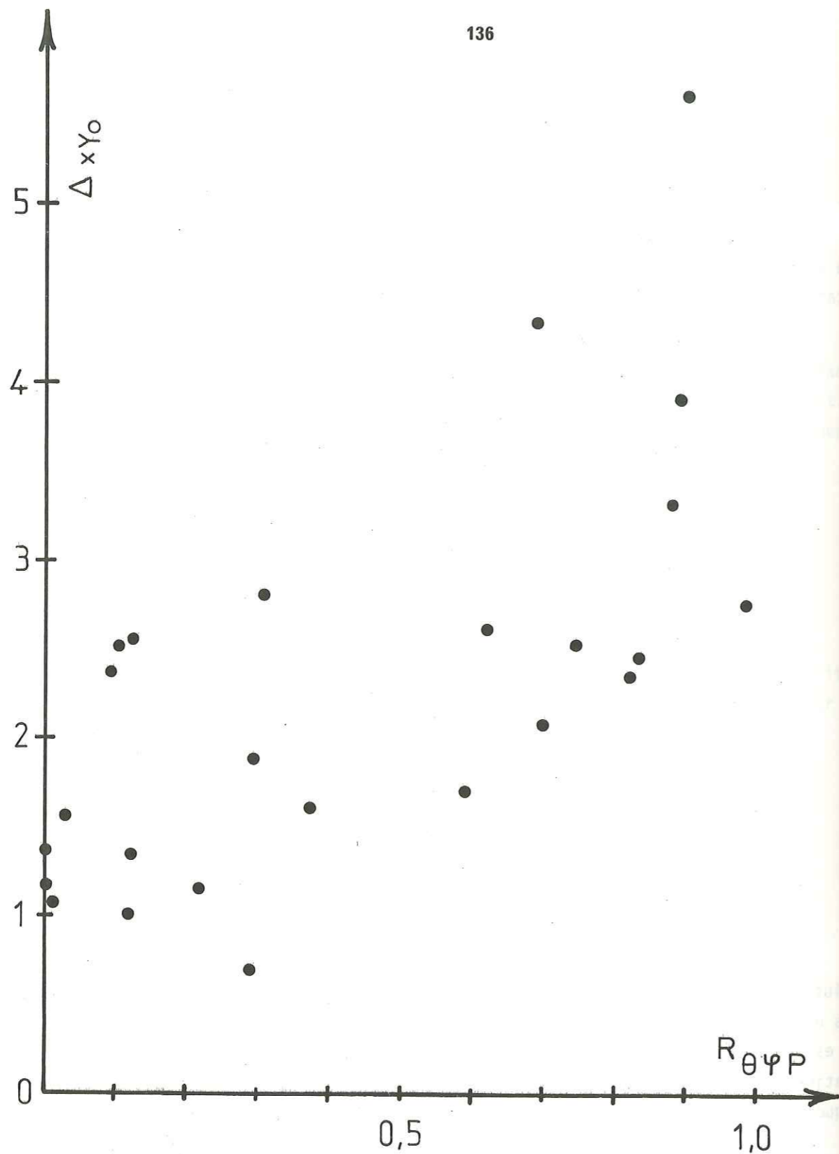
Figure IV.8 Valeurs du niveau plat \gamma_{0P} des spectres de l'onde P corrigés de l'expansion géométrique (multipliés par la distance hypocentrale), en fonction du facteur de radiation théorique R_{\theta\psi P} calculé à partir des solutions focales de la première partie.
