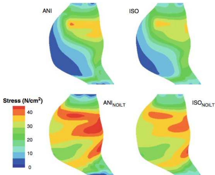
FIGURE 3.3 – Résultats de Vande Geest et al [70] montrant la répartition de la contrainte principale maximum pour un cas d'AAA. ANI = paroi anisotrope, ISO = paroi isotrope, NOILT = pas de thrombus intra luminal dans la simulation.
