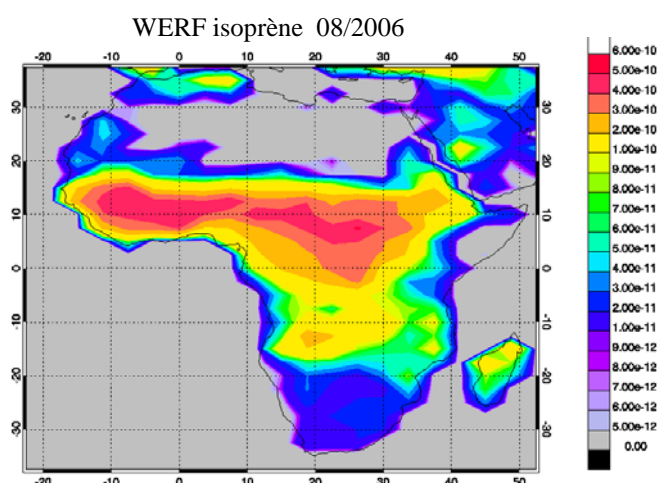
FIG. 1.16 – Flux d'émissions totales d'isoprène [Kg (C)/m 2 /s] en Afrique en août 2006 dans le cadastre d'émissions WERF.
