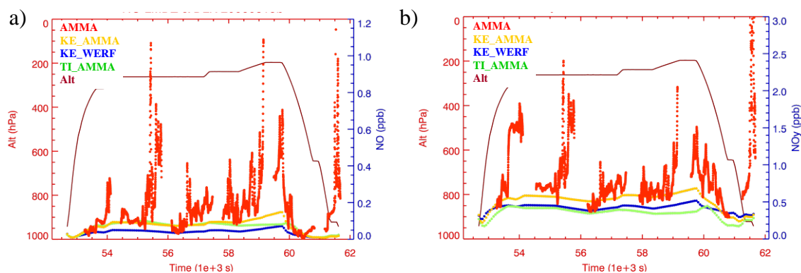
FIG 3.16 - Données (en rouge) NO (a) et NO y (b) en ppbv observées le long du vol du D_F20 le 15 août 2006; Simulations du modèle (KE_WERF, TI_AMMA, KE_AMMA).
