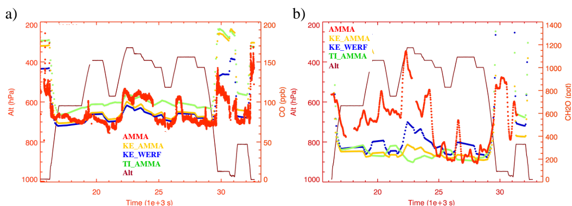
FIG. 3.10 - Données de CO (a) (ppbv) et HCHO (b) (pptv) observées au long du vol du B_146 le 15 août 2006. Simulations du modèle (KE_WERF, TI_AMMA, KE_AMMA).
