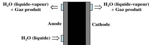
Figure 2- 5 : structure canaux électrolyseur [Lebb09][Barn05]
