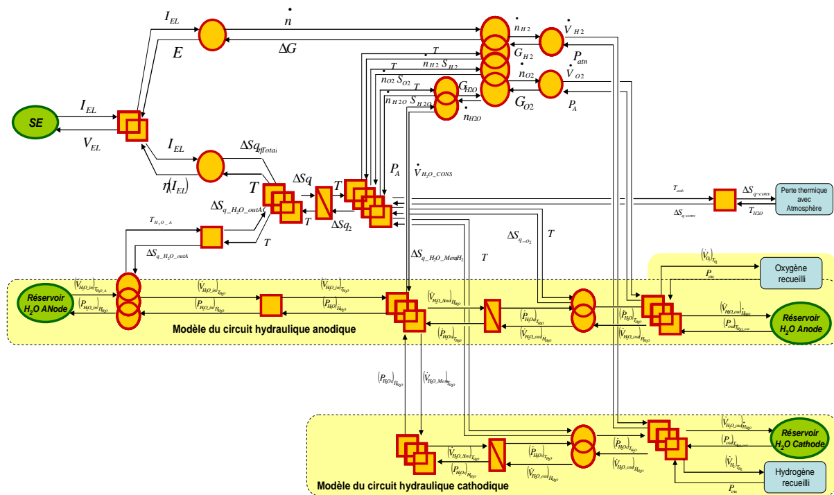
Fig. C. 5 : REM globale de l'électrolyseur avec régulation de la température du réservoir
