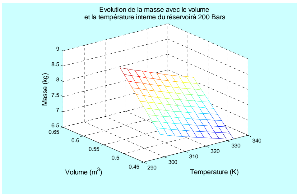
Figure 1- 11 : Masse d'hydrogène en fonction du volume et de la température
