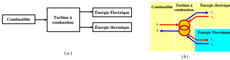
Figure 1- 18 : Distribution d'énergie ; (a) synthétique d'une cogénération par turbine à combustion ; (b) Représentation REM correspondante
