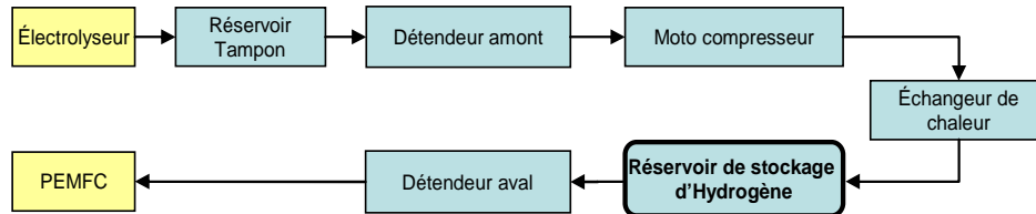
Figure 3- 15 : chaîne du circuit de stockage d'hydrogène
