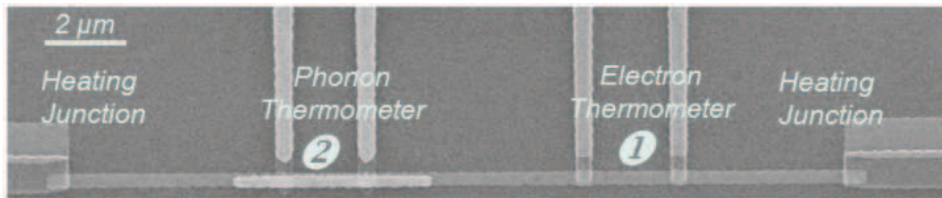
Figure 0.0.3: Image MEB du thermomètre à phonon
