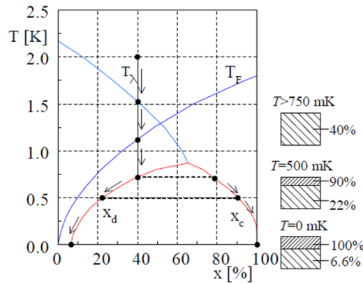
FIGURE 1.2 – Diagramme de phases de l' 3 He dans l' 4 He. En abscisse : le pourcentage d' 3 He dans le mélange et en ordonnée : la température en K
