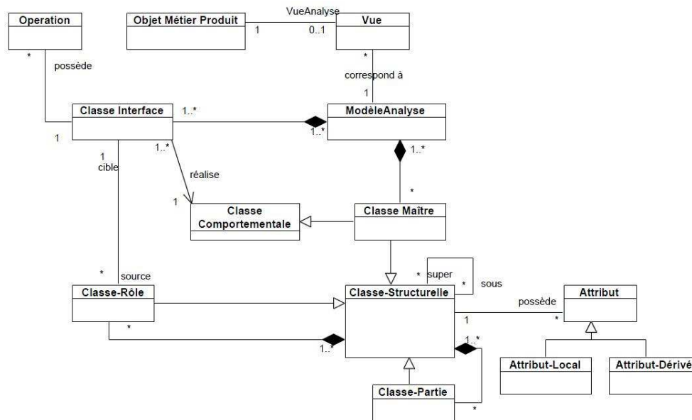
FIGURE 5.14 – Métamodèle des OM Symphony [Hassine, 2005]
