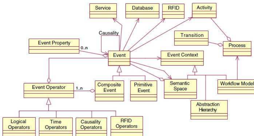
FIGURE 2.3 – Métamodèle brut d'évènements [Zang et al., 2008]
