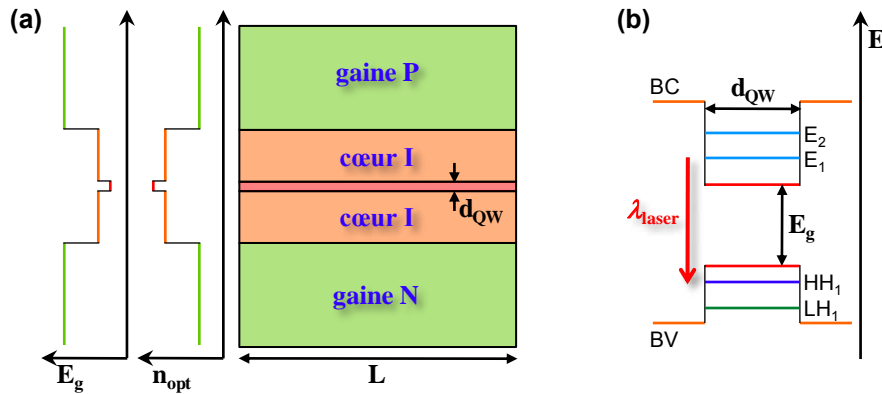
FIGURE 1.6: (a) Structure type d'une diode laser à hétérostructure et puits quantique, avec le profil de gap E_g et d'indice de réfraction n_{opt} . (b) Diagramme des niveaux énergétiques du puits quantique. BC (BV) : bande de conduction (de valence), E_i : niveaux électroniques, HH : niveau de trous lourds, LH : niveau de trous légers, E_g : énergie de gap, d_{QW} : largeur du puits quantique.
