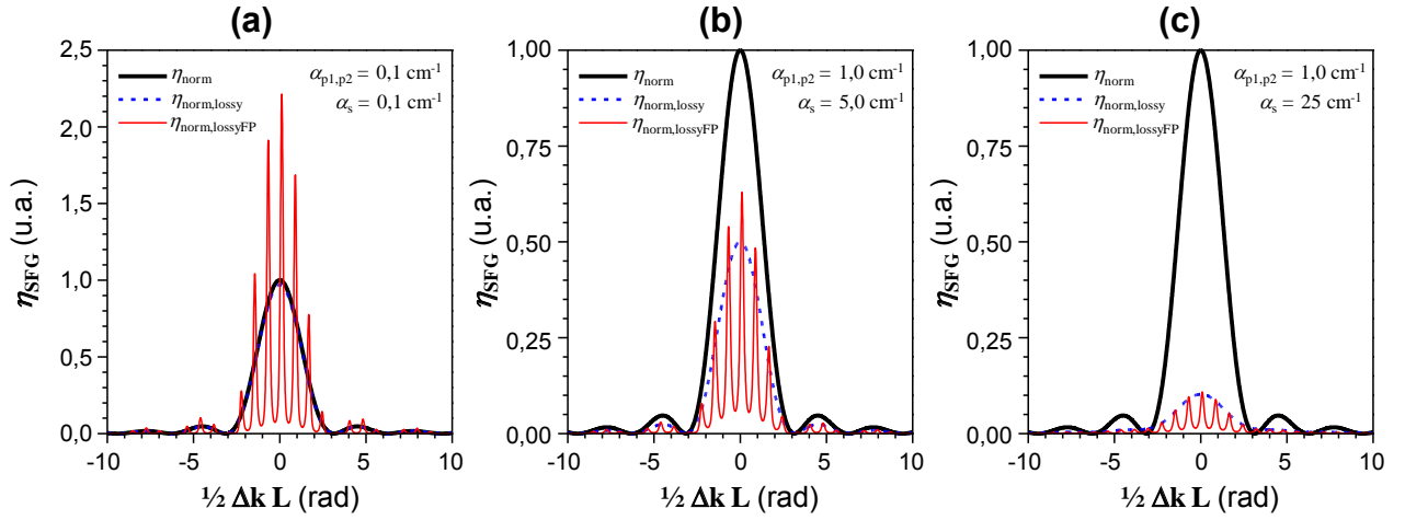
FIGURE 1.3: Simulations de l'influence des pertes modales et des effets de cavité sur l'efficacité de SFG (normalisée à 1 à l'accord de phase ( \Delta k = 0 ) en l'absence de pertes et de cavité). Nous avons considéré des réflectivités de facettes R = 30\% pour les trois modes et un guide de 2\text{ mm} de long, \alpha_{p1,p2} désigne les pertes par propagation des deux modes de pompe et \alpha_{SFG} celles du mode de SFG.
