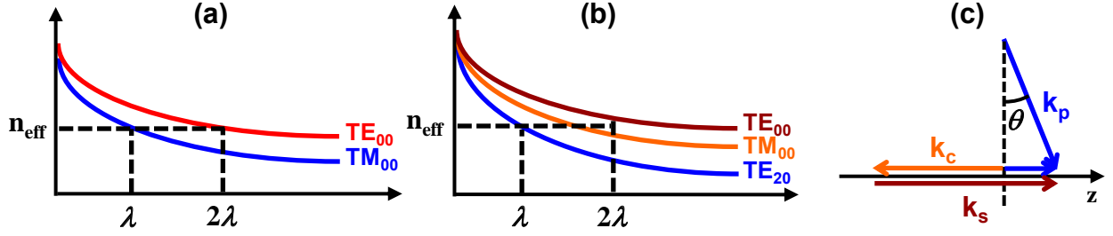
FIGURE 1.5: Stratégies d'accord de phase développées par notre équipe pour les guides d'onde en AlGaAs. (a) Accord de phase par biréfringence de forme. (b) Accord de phase modal. (c) Accord de phase contrapropageant.
