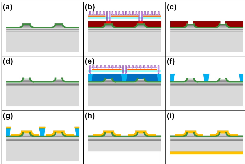
FIGURE 4.2: Étapes du dépôt de l'isolant et des contacts métalliques : (a) dépôt de SiN ; (b) enrésinement et insolation UV ; (c) développement de la résine insolée et gravure sèche pour l'ouverture du contact ; (d) nettoyage de la résine ; (e) enrésinement et insolation UV ; (f) développement de la résine ; (g) dépôt du contact P ; (h) amincissement du substrat après "lift-off" ; (i) dépôt du contact N.
