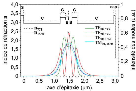
FIGURE 3.2: Profil d'indice et intensité des modes guidés dans la direction d'épitaxie d'une structure Al-free de diode à laser à photon jumeaux. "S" : substrat en GaAs, "C" : couche de gaine en \text{Al}_{0,50}\text{In}_{0,50}\text{P} (confinement), "G" : couche de cœur externe en \text{Ga}_{0,50}\text{In}_{0,50}\text{P} (exaltation du mode d'ordre 3 par rapport au mode fondamental), "B" : couche de cœur interne en \text{Al}_{0,19}\text{Ga}_{0,81}\text{As} (guidage), "cap" : casquette de protection en GaAs.
