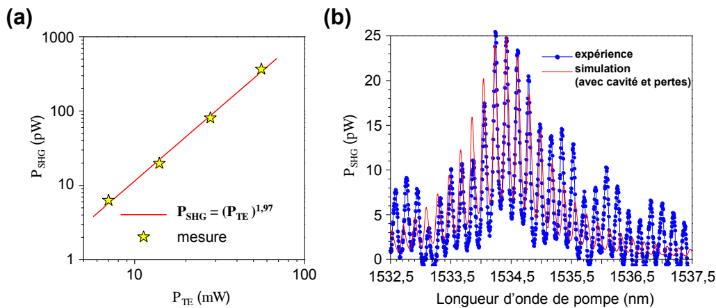
FIGURE 6.6: (a) évolution de la puissance de SHG (corrigée du bruit de fond) en fonction de la puissance infrarouge injectée sur le mode TE. (b) Spectre expérimental et simulé pour une puissance infrarouge injectée P_{TE}^{ext} = P_{TM}^{ext} = 14\text{mW} dans le guide 7 de la figure 6.3 (a). Remarque : l'asymétrie du spectre expérimental (il y a plus de puissance aux grandes longueurs d'ondes) provient principalement de la plus grande efficacité de l'amplificateur à erbium dans la plage de longueurs d'onde supérieures à 1535 nm environ.
