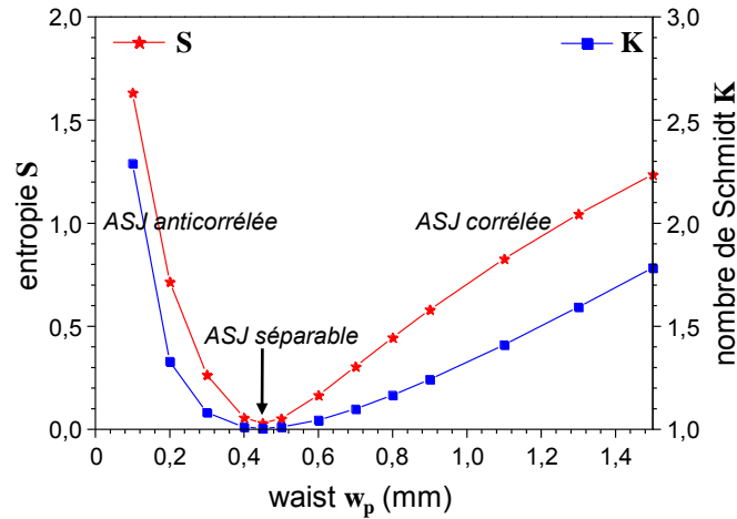
FIGURE 8.6: Evolution de l'entropie S et du nombre de Schmidt K en fonction du waist w_p du faisceau de pompe pour des impulsions de durée \tau_p = 3,5 ps. Pour w_p = 0,45 mm, l'état à deux photons décrit par l'amplitude spectrale jointe est séparable en fréquence.
