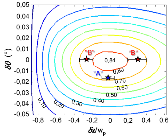
FIGURE 9.8: Evolution de la concurrence C en l'absence de bruit en fonction des décalages angulaire \delta\theta et spatial \delta z entre les deux faisceaux de pompe. Les résultats des mesures "A" et "B" sont indiqués respectivement par les étoiles bleues et rouges. Les barres d'incertitude sur \delta z sont déduites des barres d'erreur sur la valeur de concurrence.
