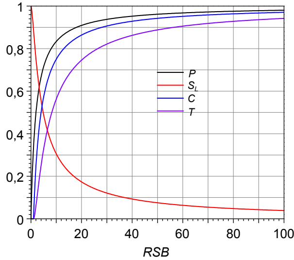
FIGURE 1.9: Fidélité maximale P , entropie linéaire S_L , concurrence C et tangle T en fonction du rapport signal à bruit pour un état de Werner. On observe que dès que RSB < 1 , aucune intrication n'est préservée et que la fidélité maximale est supérieure à 90% à partir d'un RSB de 18, et supérieure à 95% à partir d'un RSB de 38.
