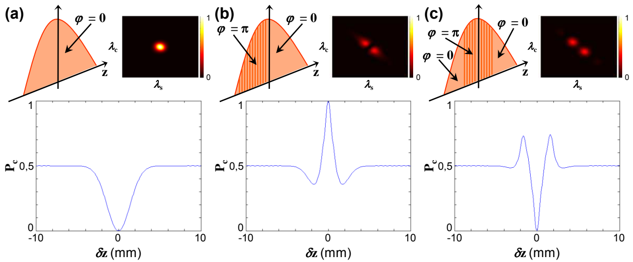
FIGURE 8.9: Probabilité de coïncidence P_c en fonction de la différence de marche \delta z de l'interférence de Hong-Ou-Mandel des photons d'une paire générée avec un faisceau de pompe gaussien de waist w_p = 0,45 \text{ mm} . Au-dessus des graphes, on a représenté le profil de phase du faisceau de pompe à gauche et l'ISJ correspondante à droite. (a) Sans aucun déphasage, on observe le fameux "dip" de Hong-Ou-Mandel. (b) Avec un déphasage de \pi sur la moitié des z < 0 , on observe au contraire un excès de coïncidences. (c) Avec un déphasage de \pi sur le centre du faisceau, on retrouve un creux de coïncidences avec deux lobes latéraux en plus.
