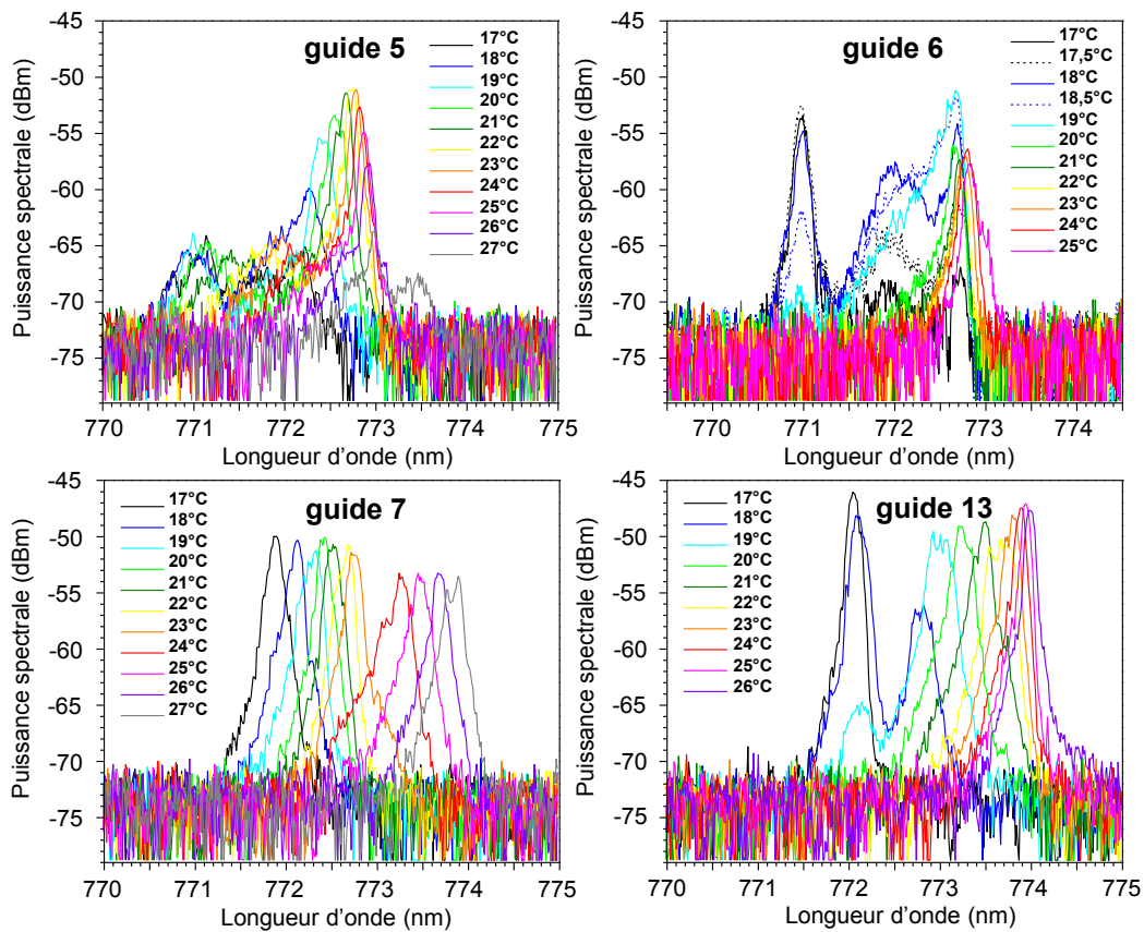
FIGURE 6.5: Spectre du mode laser, mesuré à l'analyseur de spectre optique (OSA), en fonction de la température du support pour quatre diodes. Les diodes sont les mêmes qu'en figure 6.3 (a).
