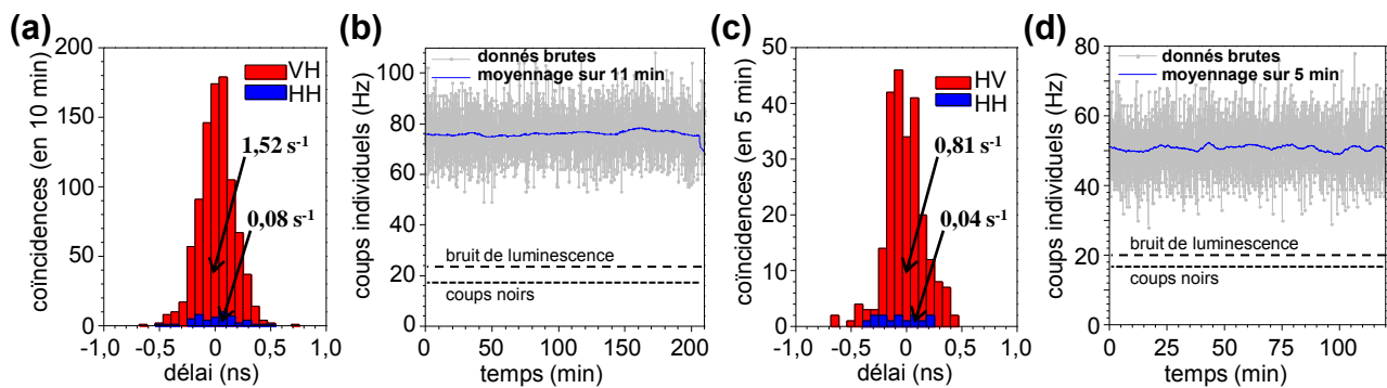
FIGURE 9.6: Rapport signal à bruit et stabilité des tomographies "A" (a,b) et "B" et (c,d) . (a) Deux histogrammes de coïncidences obtenus en 10 minutes pour les configurations HH et VH : on mesure 0,08 coïncidences accidentelles et 1,44 vraies coïncidences par seconde. (b) Nombre de photons détectés par seconde sur une des deux voies au cours de la tomographie : le taux de comptage est relativement stable sur les trois heures et demie d'acquisition. On a indiqué en traits tiretés les niveaux du bruit de coups noirs et du bruit de luminescence (obtenus respectivement en bloquant les photons de la voie et en décalant la longueur d'onde centrale du filtre Fabry-Perot). (c) Histogrammes HH et HV acquis en 5 minutes : on mesure 0,04 coïncidences accidentelles et 0,77 vraies coïncidences par seconde. (d) Nombre de photons détectés par seconde sur une des deux voies au cours de la tomographie : là encore, la manip était relativement stable sur les deux heures d'acquisition.
