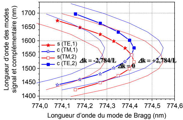
FIGURE 6.9: Courbes d'accord de phase simulées pour l'interaction de type 2 à 20°C sur la structure active nominale (traits épais). On a également représenté en traits fins les courbes d'accord de phase à mi-hauteur ( \Delta k = \pm \frac{2,784}{L} ) pour un échantillon de 2,1 mm.
