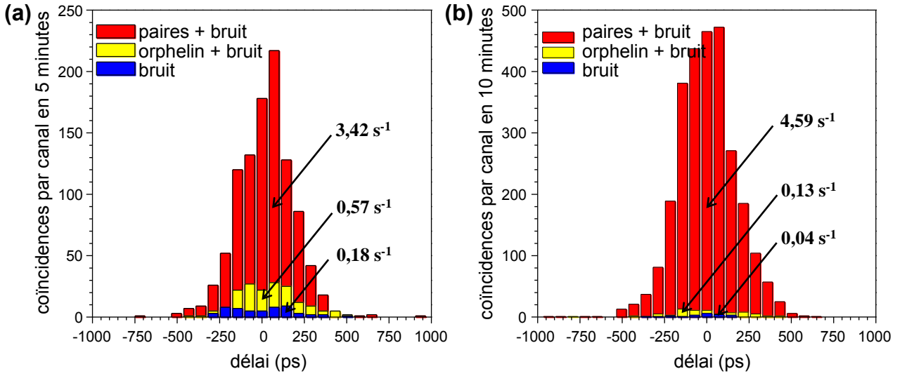
FIGURE 8.4: Histogrammes de coïncidences enregistrés avec des filtres interférentiels passe-bande de 12 nm (a) ou des filtres interférentiels passe-haut à 1450 nm associés à des filtres Fabry-Perot fibrés de 1,2 nm (b). Rouge : les deux filtres sont centrés sur les photons paramétriques, jaune : seul un des filtres est centré sur les photons paramétriques, bleu : les deux filtres sont centrés loin des photons paramétriques.
