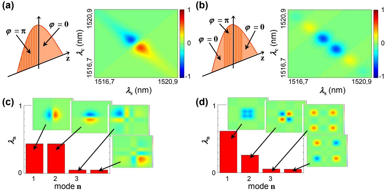
FIGURE 8.8: Deux exemples d'ASJ à deux lobes principaux (a,b) pouvant être obtenues avec un faisceau de pompe gaussien de waist w_p = 0,45 \text{ mm} et dont une portion est déphasée d'une phase \pi (schémas à gauche des ASJ), et leurs décompositions de Schmidt respectives (c,d). (a,c) Etat obtenu pour un déphasage de \pi sur la moitié des z < 0 . (Seule la partie imaginaire de l'ASJ est représentée, la partie réelle étant nulle.) (b,d) Etat obtenu pour un déphasage de \pi sur la partie centrale du faisceau ( -250\mu\text{m} < z < 250\mu\text{m} ). (Seule la partie réelle de l'ASJ est représentée, la partie imaginaire étant nulle.)
