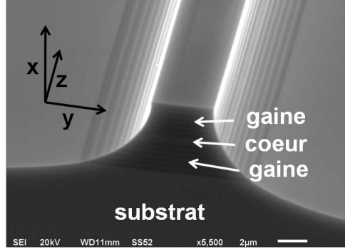
FIGURE 1.2: Image MEB (microscope électronique à balayage) d'un guide d'onde en AlGaAs (échantillon ABQ71) montrant la géométrie des guides rubans utilisés dans cette thèse.
