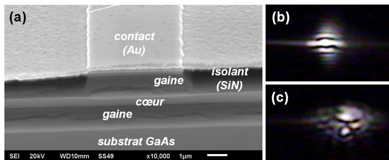
FIGURE 2.2: (a) Images MEB d'un échantillon de diode laser à mode d'ordre 3 : les deux couches de gaine sont entièrement oxydées et présentent des fissures. (b) Champ proche d'un mode d'ordre 3. (c) Champ proche du mode dégradé après quelques heures de fonctionnement.
