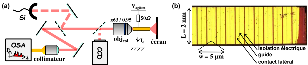
FIGURE 6.2: (a) Schéma du banc de test des diodes lasers. Si : puissance-mètre silicium, OSA : analyseur de spectre optique, CCD : caméra CCD silicium. Le module de refroidissement Peltier n'est pas représenté sur ce schéma. (b) Vue de dessus d'une barrette de diodes de 2 mm de long.
