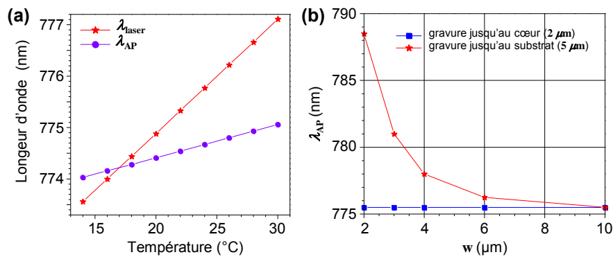
FIGURE 3.8: (a) Simulations de l'évolution des longueurs d'onde laser et d'accord de phase en fonction de la température pour la structure nominale. (b) Longueur d'onde d'accord de phase simulée en fonction de la largeur du guide ruban pour deux profondeurs de gravure : sur 2 \mu\text{m} jusqu'au cœur (carrés bleus) et sur 5 \mu\text{m} jusqu'au substrat (étoiles rouges). Les lignes sont juste un guide pour les yeux.
