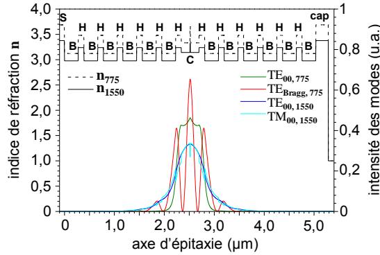
FIGURE 3.5: Profil d'indice et intensité des modes guidés dans la direction d'épitaxie d'une diode laser à photons jumeaux à miroirs de Bragg. "S" : substrat en GaAs, "H" : couches de haut indice en \text{Al}_{0,25}\text{Ga}_{0,75}\text{As} (miroirs de Bragg), "B" : couches de haut indice en \text{Al}_{0,80}\text{Ga}_{0,20}\text{As} (miroirs de Bragg), "C" : couche de cœur en \text{Al}_{0,45}\text{Ga}_{0,55}\text{As} (guidage), "cap" : casquette de protection en GaAs.
