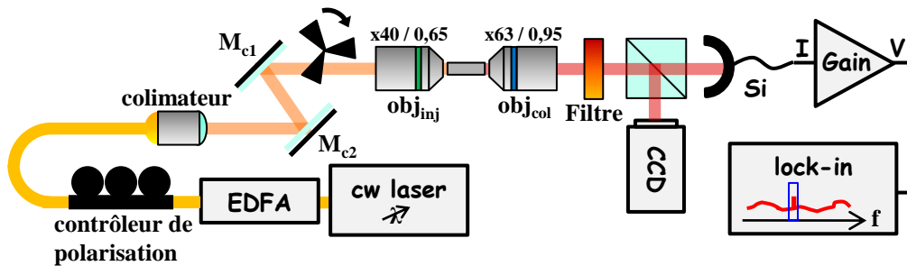
FIGURE 5.1: Montage utilisé pour l'expérience de SHG. Voir le texte pour le rôle des différents éléments. cw laser : laser continu accordable, EDFA : amplificateur à erbium, Filtre : filtre passe-bas, CCD : caméra CCD, Si : photodiode silicium, Gain : amplificateur transimpédance, lock-in : détection synchrone.
