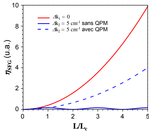
FIGURE 1.4: Comparaison de l'efficacité de SFG en fonction de la longueur du milieu non linéaire dans le cas d'un accord de phase parfait (en trait plein rouge), d'un désaccord de phase (en trait plein bleu) et d'un quasi-accord de phase (en trait tireté bleu). L_c désigne la longueur de cohérence : elle dépend du désaccord de phase et correspond à la longueur sur laquelle l'interaction non linéaire reste constructive. Pour obtenir un quasi-accord de phase optimal, la période d'inversion doit être égale à L_c .
