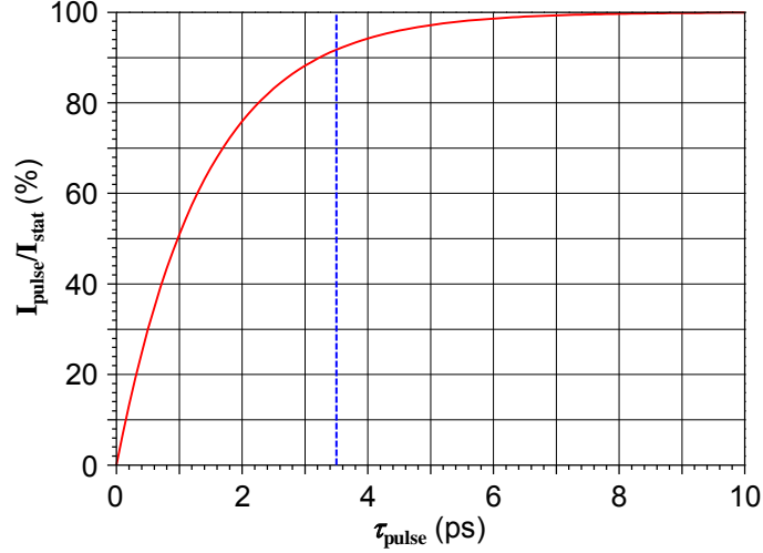
FIGURE 8.2: Amplification de la microcavité verticale en fonction de la durée de l'impulsion laser. Le trait tireté vertical correspond à la durée de l'impulsion de pompe utilisée.
