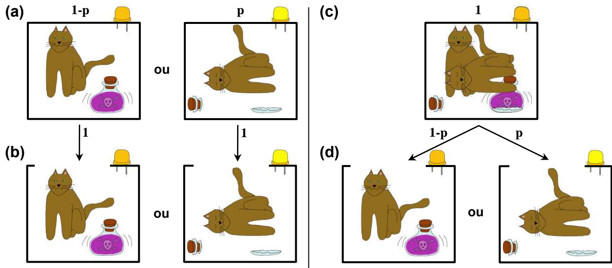
FIGURE 1.8: Expérience de pensée dite du "Chat de Schrödinger" : On place le chat et la fiole de produit chimique dans une boîte munie d'un témoin lumineux (LED jaune) et on ferme la boîte. Etat classique : (a) boîte fermée, le chat peut être vivant avec une probabilité 1 - p ou mort avec une probabilité p : le témoin nous renseigne sur l'état du chat ; (b) après ouverture de la boîte, le chat est dans l'état qu'indiquait le témoin avec une probabilité 1. Etat intriqué : (c) boîte fermée, le chat est vivant et mort : le témoin ne peut pas nous renseigner sur l'état du chat ; (d) après ouverture de la boîte, le chat est vivant avec une probabilité 1 - p ou mort avec une probabilité p .
