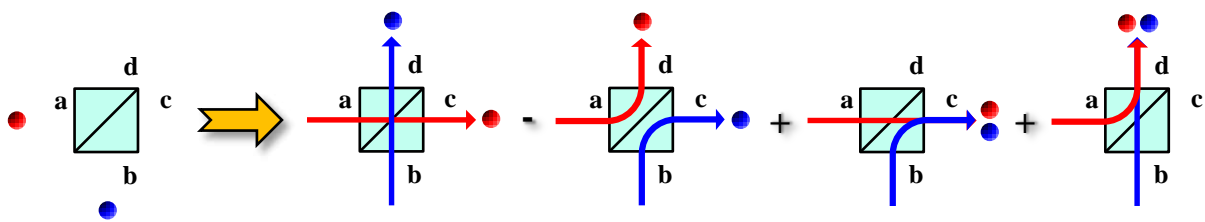
FIGURE 7.3: Vision schématique de l'interférence à deux photons sur une séparatrice 50-50 : si les photons sont indiscernables, leurs probabilités de sortie par deux voies différentes s'annulent tandis que celles de sortie groupée sur une même voie s'additionnent. Les photons sortent donc de la séparatrice tous les deux par la même voie et on n'enregistre aucune détection en coïncidence derrière la séparatrice.
