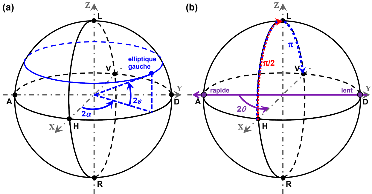
FIGURE 1.7: Sphère de Poincaré. (a) Géographie de la sphère. (b) Effet d'une lame d'onde sur les polarisations (voir le texte).
