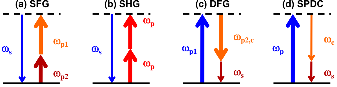
FIGURE 1.1: Interactions non linéaires à 3 photons : (a) génération de somme de fréquence, (b) génération de seconde harmonique (cas particulier de la SFG), (c) génération de différence de fréquence, (d) fluorescence paramétrique. L'indice "p" désigne le(s) champ(s) de pompe et les indices "s" et "c" désignent le signal et le complémentaire résultant de l'interaction.
