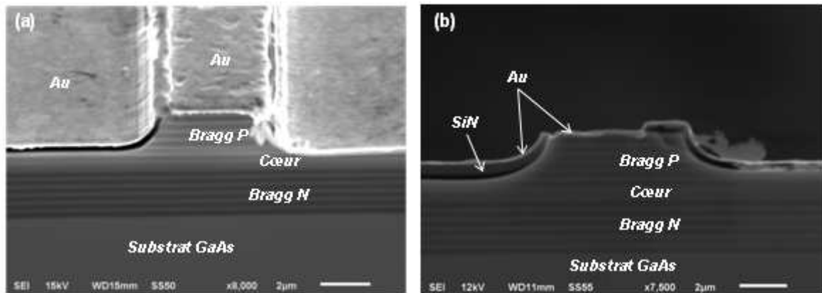
FIGURE 6.1: Images MEB de deux échantillons de diode laser à mode de Bragg. On distingue nettement les différentes couches de l'empilement. On distingue aussi la différence entre les dopages N et P (les couches dopées N sont plus sombres). (a) Echantillon B3R151 vu de dessus. (b) Echantillon C4T46 vu de la facette.
