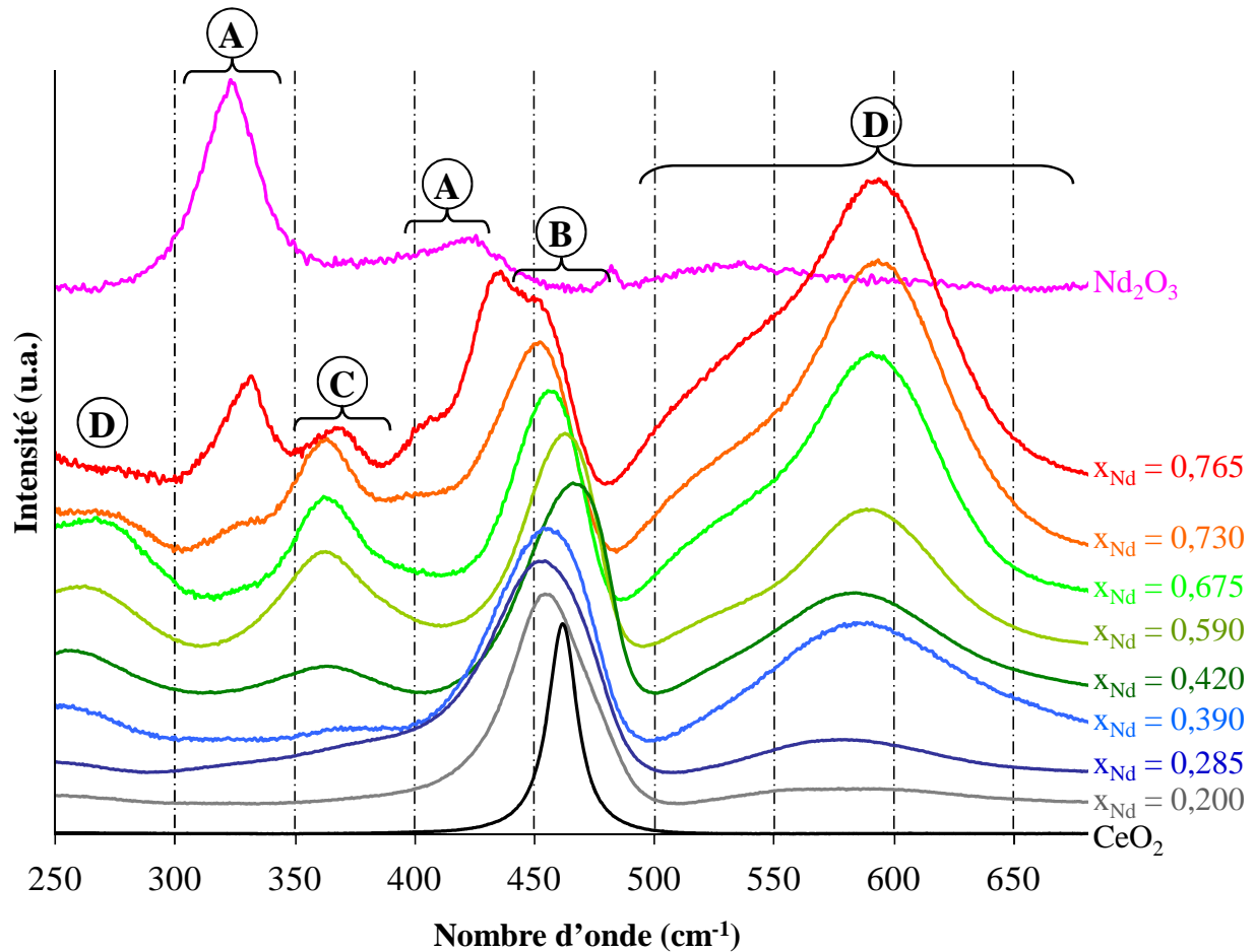
Figure 23. Spectres \mu -Raman enregistrés pour \text{Ce}_{1-x}\text{Nd}_x\text{O}_{2-x/2} . Les lettres entourées pointent les bandes caractéristiques des modes de vibration de la structure de type A 127 ( A ), des modes de vibration F_{2g} de la structure fluorine de \text{CeO}_2 ( B ), des modes de vibration liés à la structure de type C ( C ), et des modes de vibrations de la liaison M-O dans les structures de type F et C, pour laquelle le cation est coordonné par au moins une lacune en oxygène ( D ).
