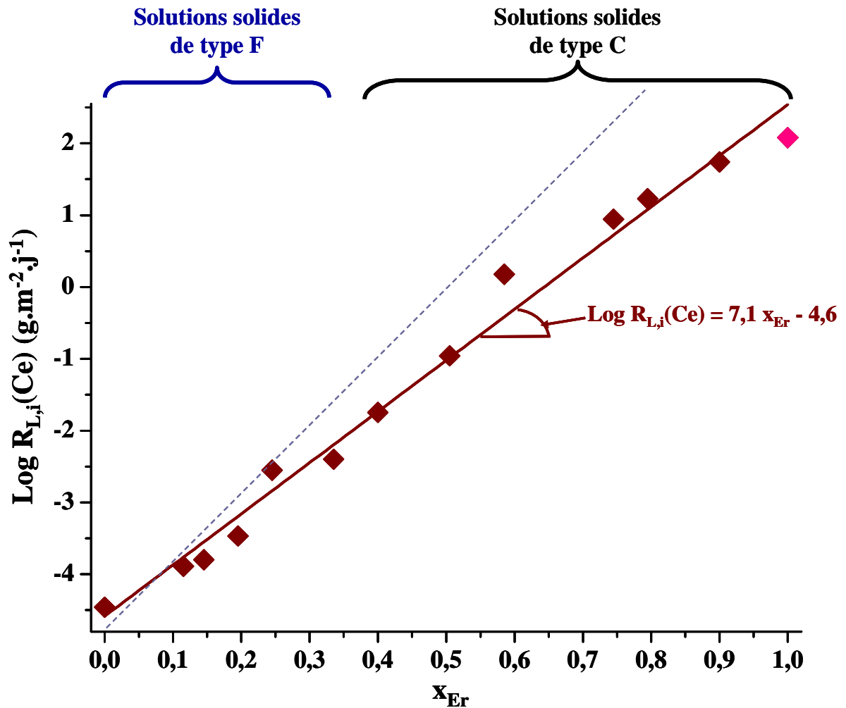
Figure A-4. Variation du logarithme de la vitesse de dissolution normalisée des solutions solides \text{Ce}_{1-x}\text{Er}_x\text{O}_{2-x/2} en fonction de la fraction en erbium x_{\text{Er}} ( \text{HNO}_3 4M, T = 60^\circ\text{C} ). La droite marron correspond à la régression linéaire des points expérimentaux tandis que le trait pointillé bleu indique à titre de comparaison la régression linéaire obtenue pour le système \text{Ce}_{1-x}\text{Nd}_x\text{O}_{2-x/2} dans les mêmes conditions expérimentales.
