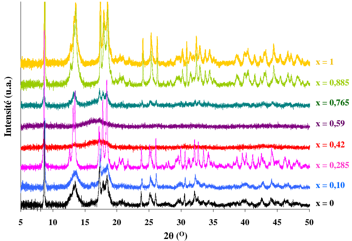
Figure 6. Diffractogrammes RX sur poudre obtenus pour les oxalates \text{Ce}_{1-x}\text{Nd}_x(\text{C}_2\text{O}_4)_{1,5} \cdot y\text{H}_2\text{O} .
